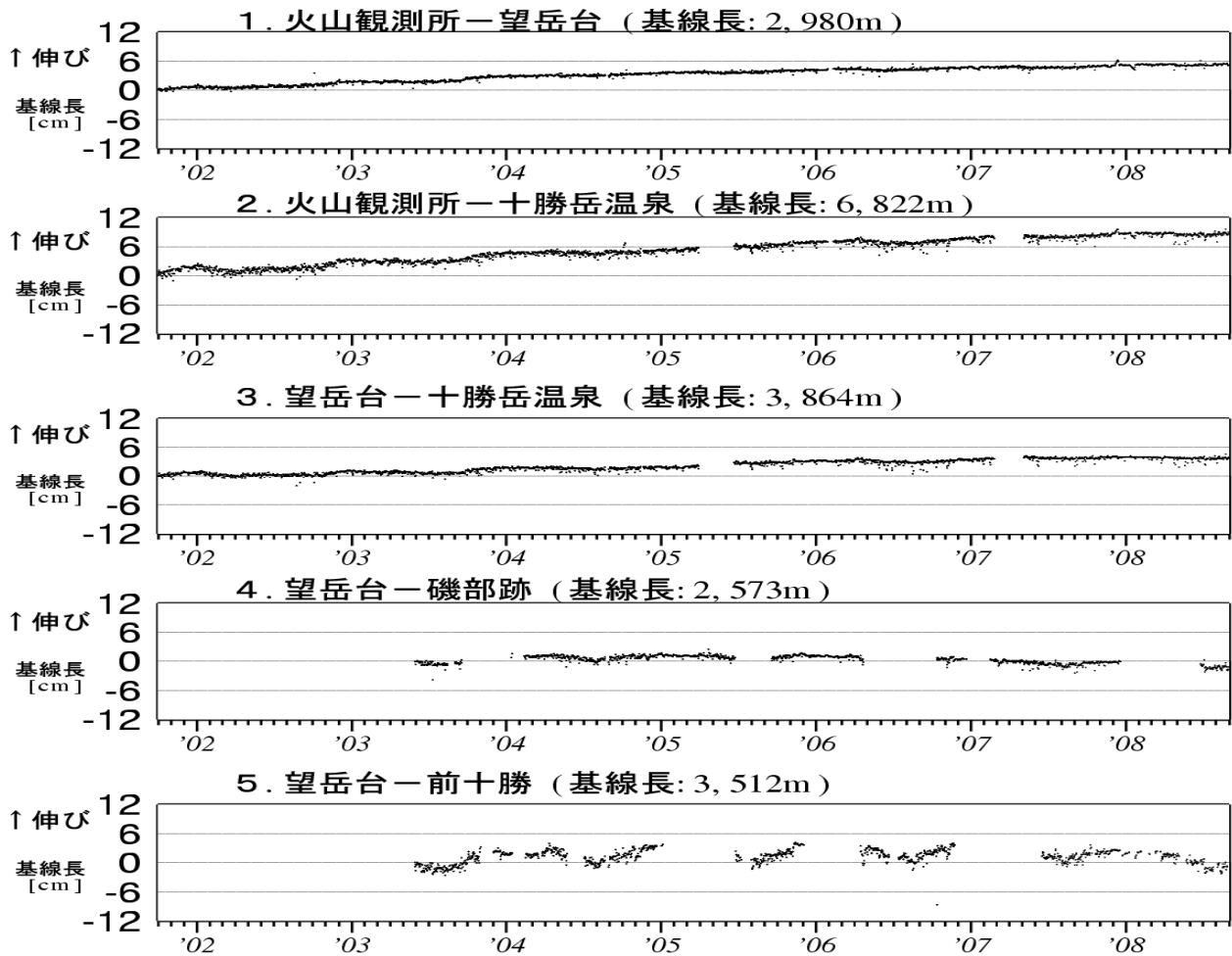
図 5※ 十勝岳 GPS 連続観測による基線長変化（2001 年 10 月～2008 年 8 月） グラフの空白部分は欠測。
