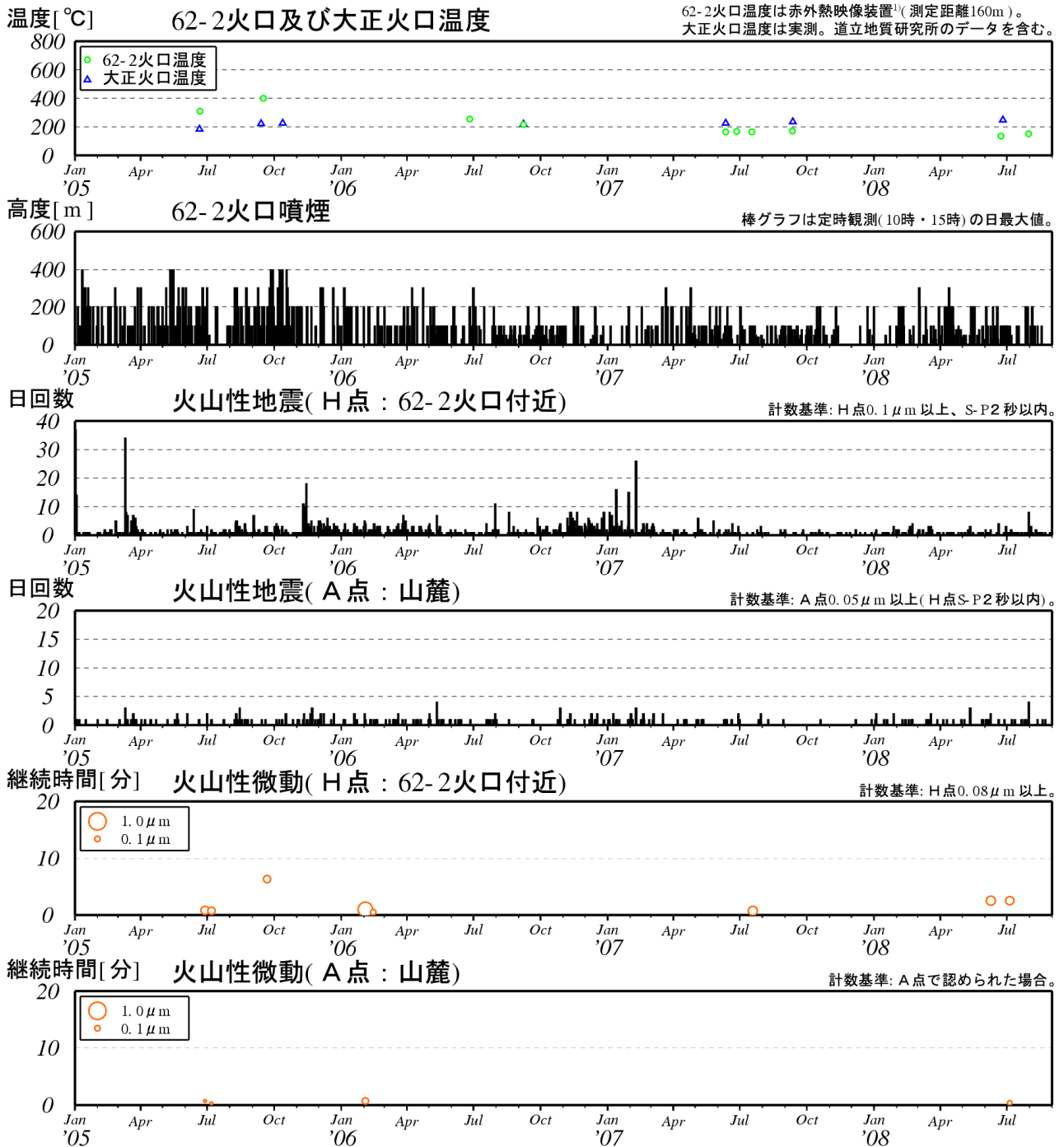
図 3 ※ 十勝岳 最近の火山活動経過図（2005 年 1 月～2008 年 8 月）
