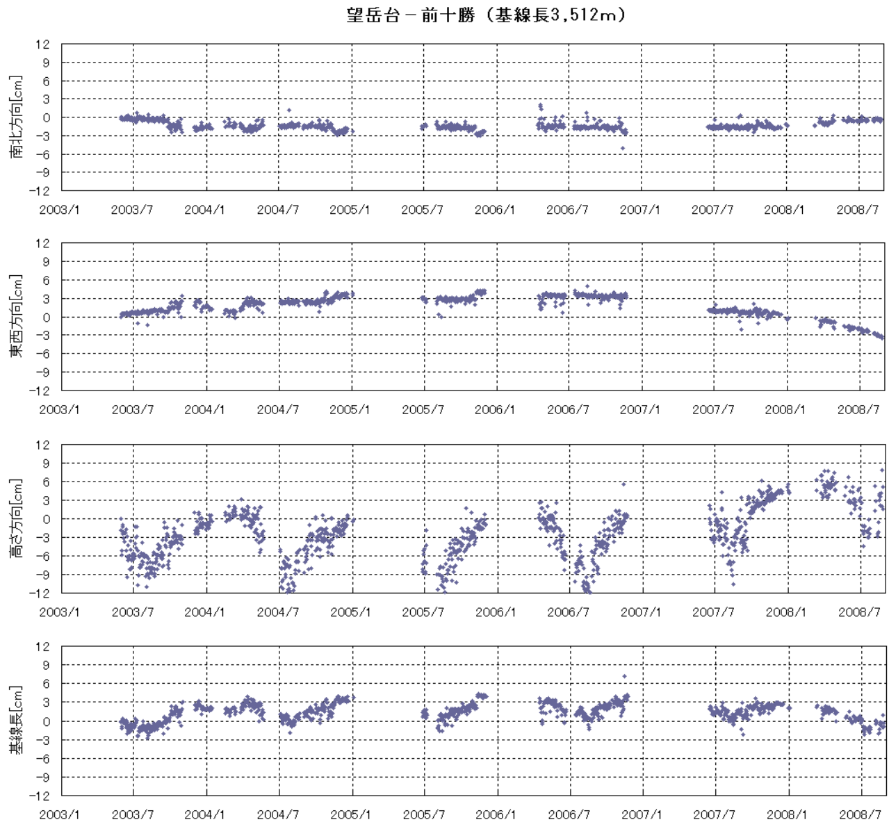
図 7※ 十勝岳 GPS による望岳台と前十勝の距離の成分毎時系列変化 (2003 年 5 月～2008 年 8 月)
