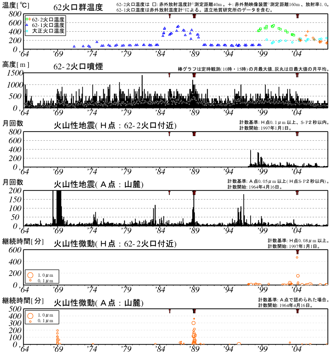
図 2 ※ 十勝岳 長期の火山活動経過図（1964 年 1 月～2008 年 8 月）
