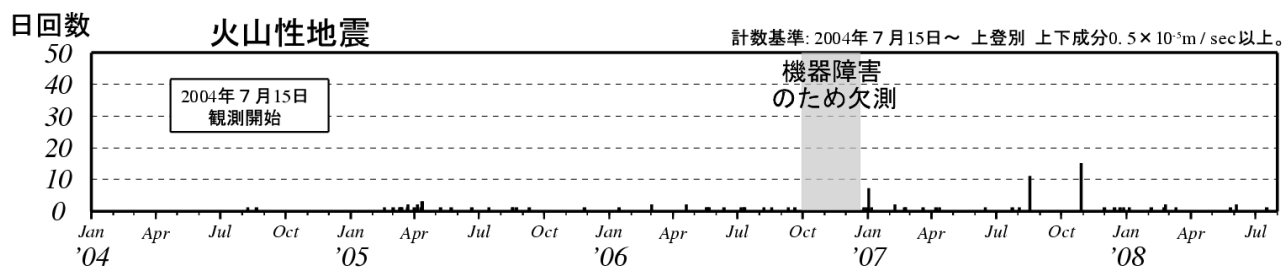
図 1 倶多楽 日別地震回数（2004 年 7 月～2008 年 7 月）
