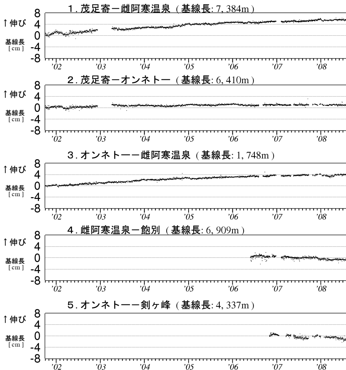
図5 雌阿寒岳 GPS 連続観測による基線長変化 (2001年10月~2008年7月) グラフの空白部分は欠測 図5の1~5は、図5のGPS基線①~⑤に対応しています。
