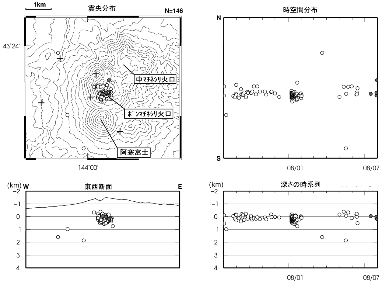
図 4 雌阿寒岳 震源分布図 (2007 年 8 月~2008 年 7 月、+は地震観測点)
