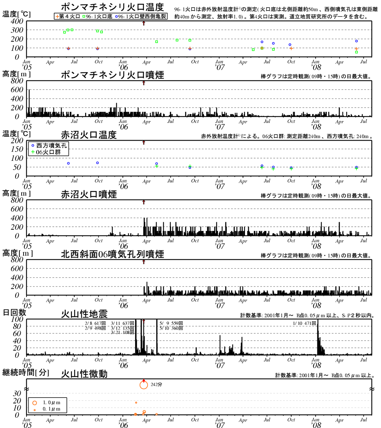
図3※ 雌阿寒岳 最近の火山活動経過図 (2005年1月～2008年7月) ↑印は噴火
