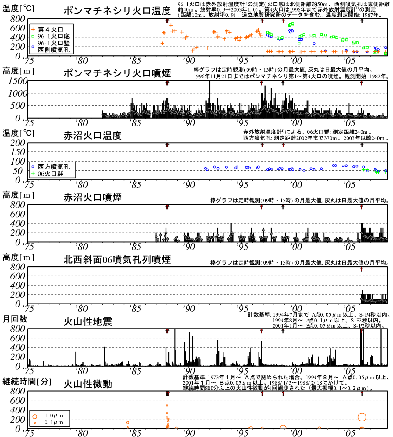
図 2* 雌阿寒岳 長期の火山活動経過図 (1975 年 1 月~2008 年 7 月) ↑印は噴火 (1988 年、1996 年、1998 年: ポンマチネシリ火口からの噴火、2006 年: 赤沼火口からの噴火)
