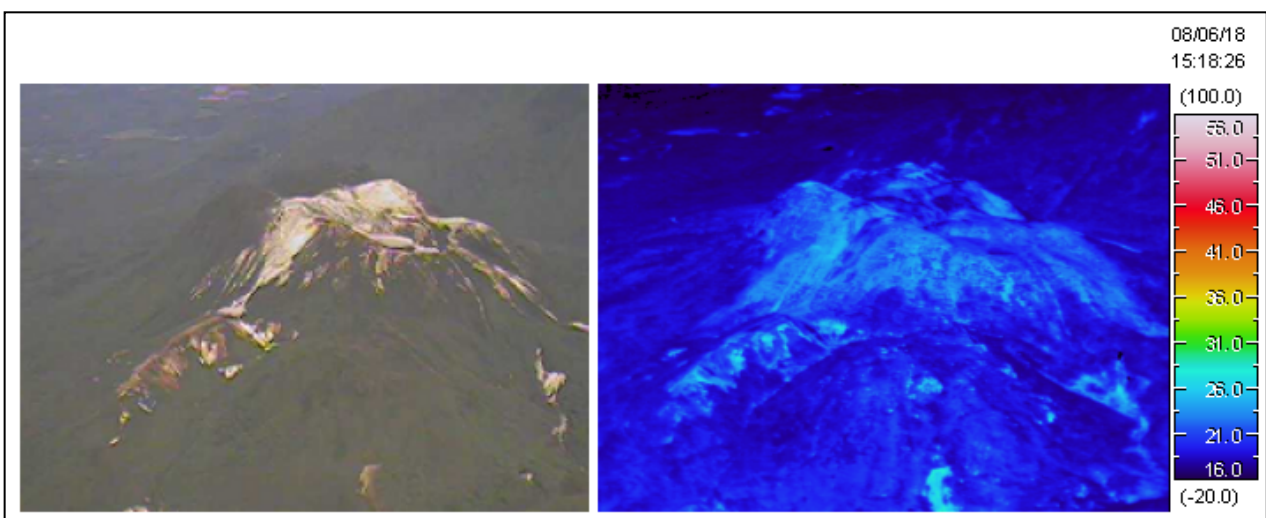
図 3 ニセコ 赤外熱映像装置 1) によるイワオヌプリ山頂付近の地表面温度分布 (2008 年 6 月 18 日 図 1 の②方向上空より撮影)
