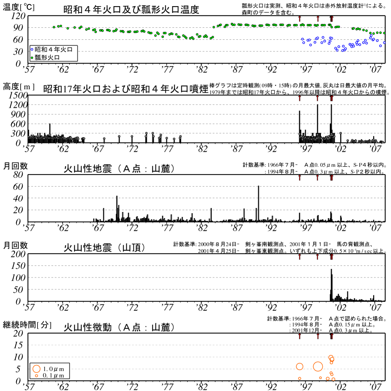
図 2 ※ 北海道駒ヶ岳 長期の火山活動経過図（1957 年 1 月～2008 年 6 月）↑印は噴火
