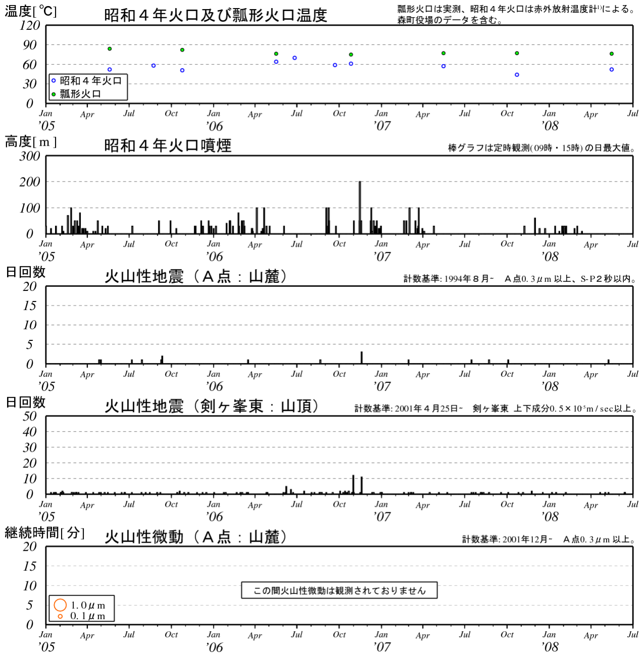
図 3※ 北海道駒ヶ岳 最近の火山活動経過図（2005 年 1 月～2008 年 6 月）
