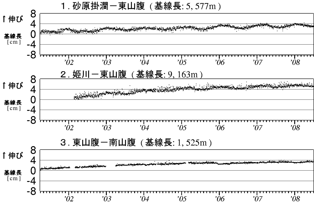
図5 北海道駒ヶ岳 GPS 連続観測による基線長変化（2001 年 4 月～2008 年 6 月）
