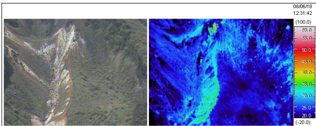
図 3 恵庭岳 赤外熱映像装置 1) による東側の爆裂火口付近の地表面温度分布 (2008 年 6 月 18 日 図 1 の矢印方向上空より撮影)
