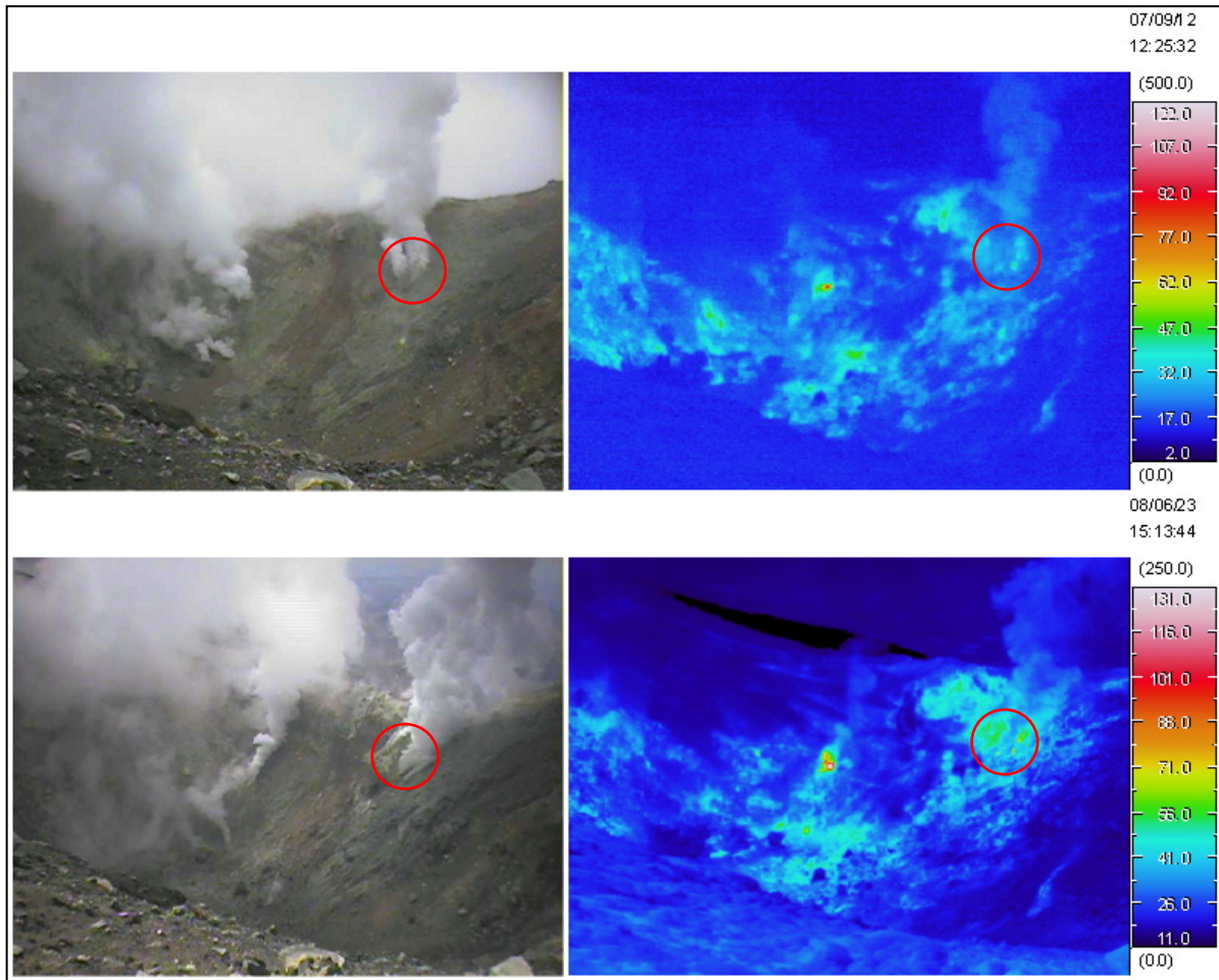
図 4 十勝岳 赤外熱映像装置 1) による62 - 2火口の地表面温度分布 ○：北側内壁の噴気孔 （上：2007年9月12日 下：2008年6月23日 図6 ■より撮影）
