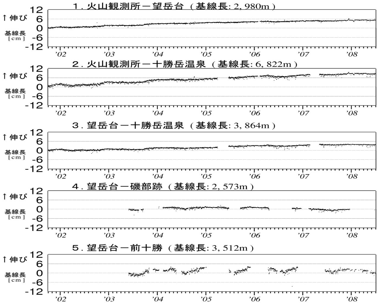
図 8※ 十勝岳 GPS 連続観測による基線長変化（2001 年 10 月～2008 年 6 月） グラフの空白部分は欠測。
