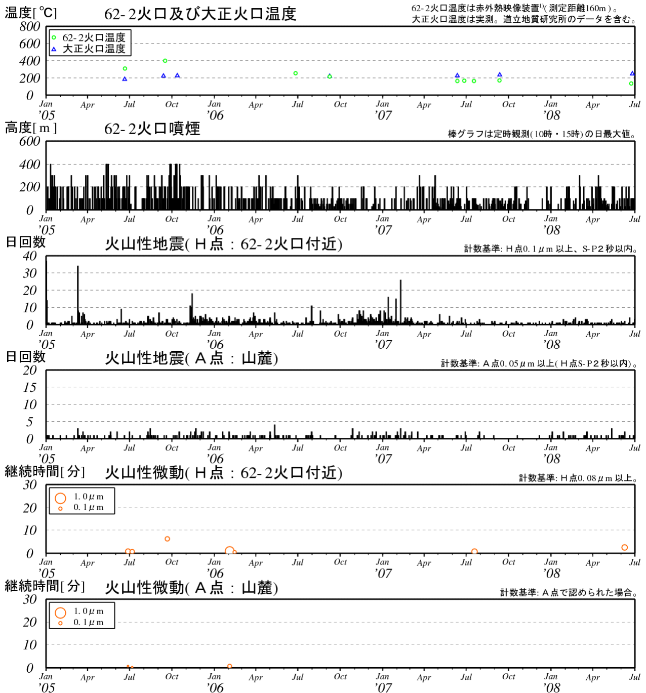
図3※ 十勝岳 最近の火山活動経過図（2005年1月～2008年6月）
