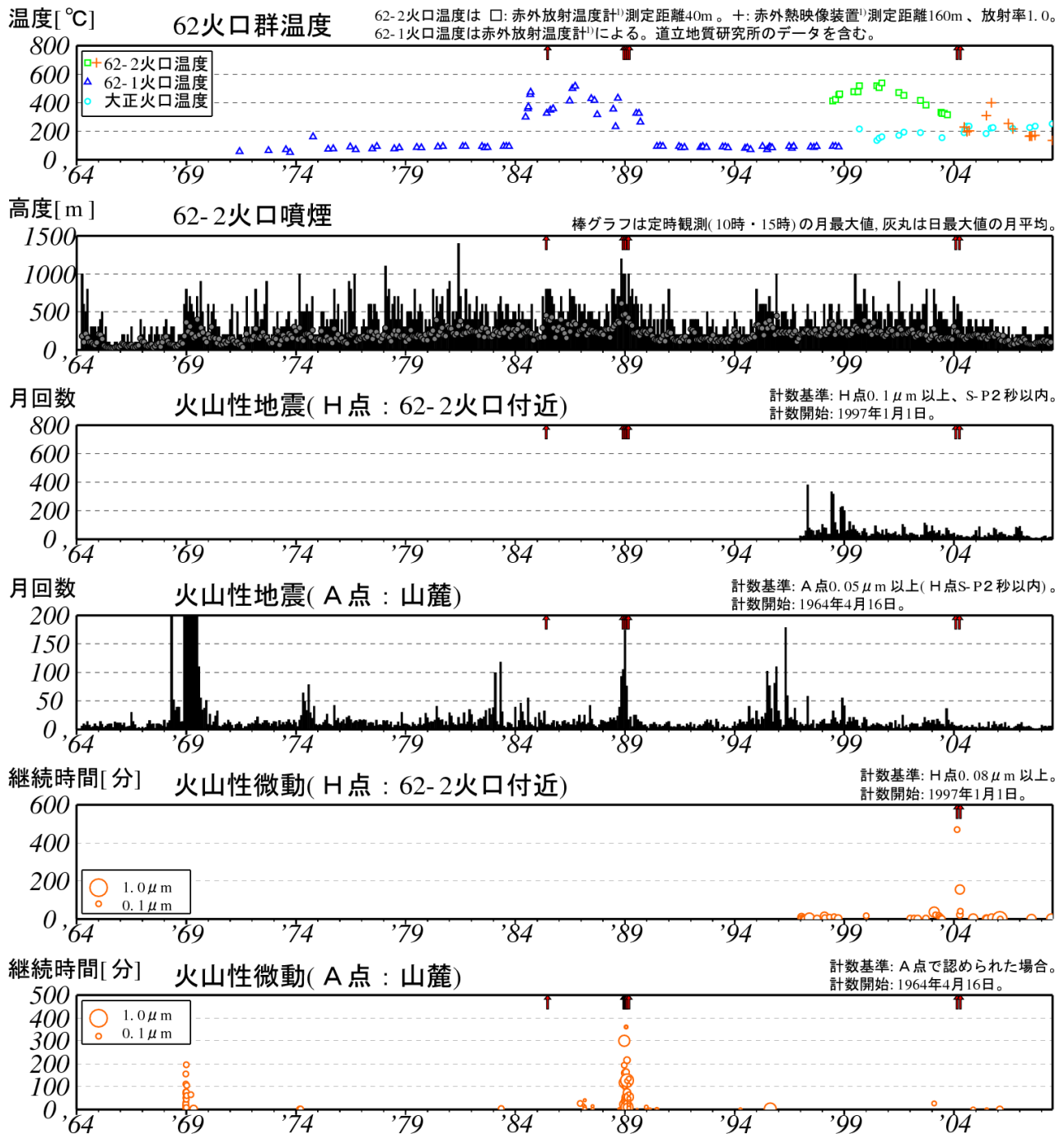
図 2※ 十勝岳 長期の火山活動経過図（1964 年 1 月～2008 年 6 月）
