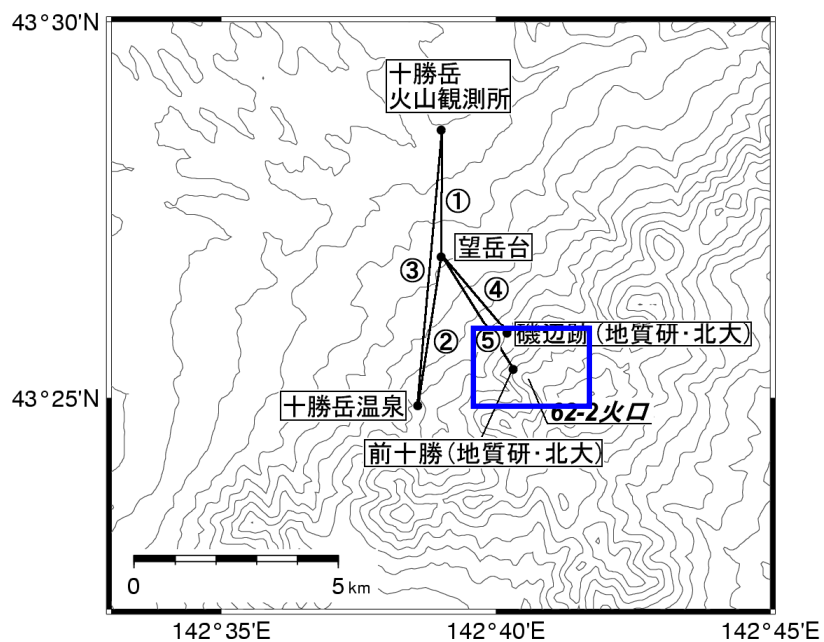
図 9 十勝岳 GPS 観測点配置図（□は図 10 の範囲）
