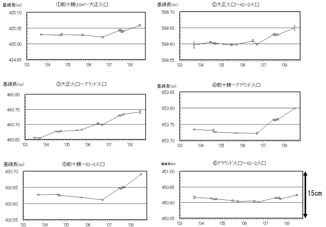
図 10※ 十勝岳 GPS 繰り返し観測による火口付近の基線長変化
