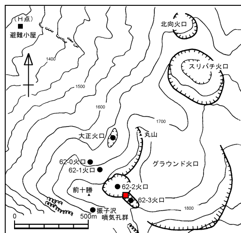
図 6 十勝岳 火口周辺図
