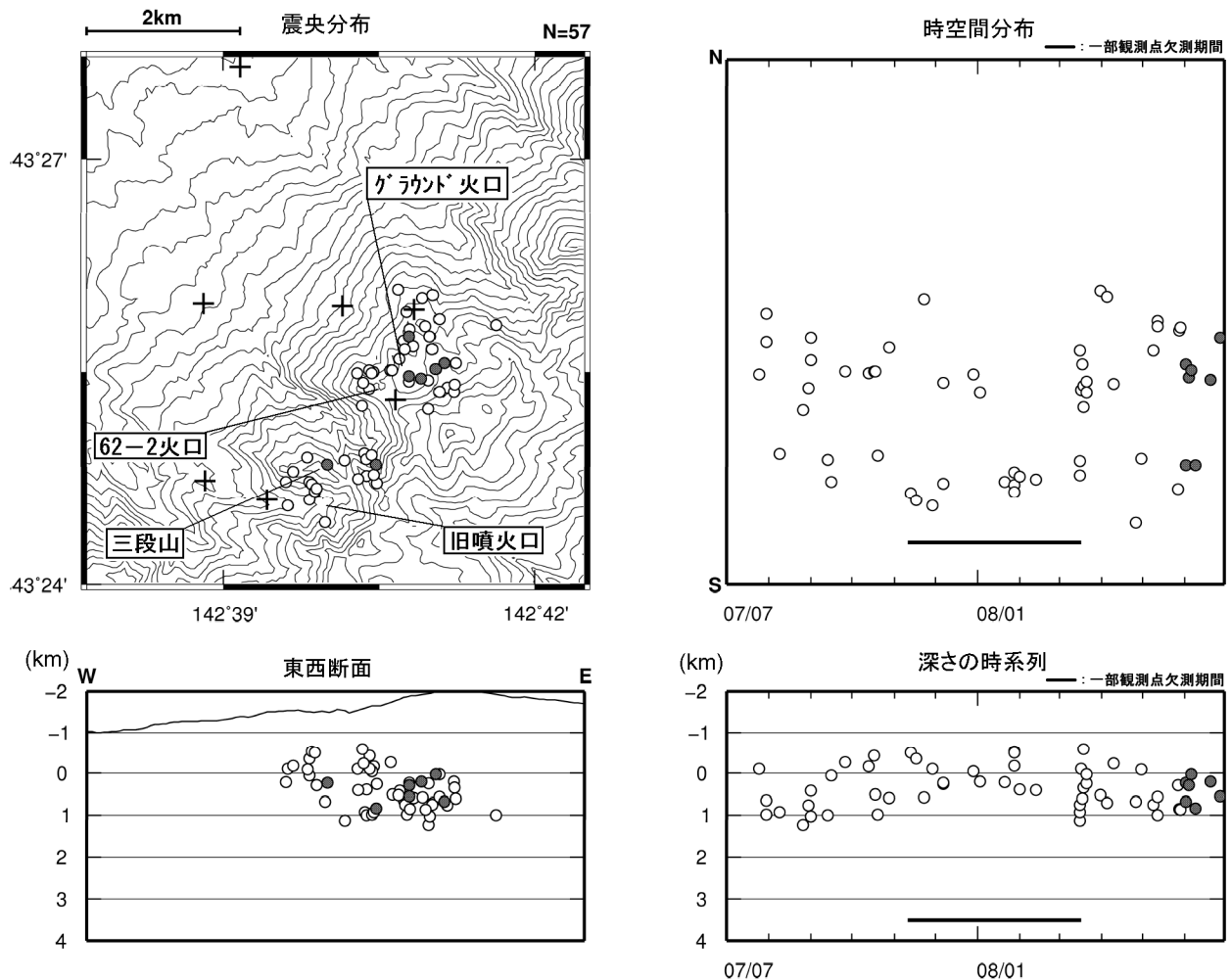
図 7 ※ 十勝岳 震源分布図（2007 年 7 月～2008 年 6 月、+は地震観測点）
