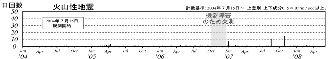
図 1 倶多楽 日別地震回数（2004 年 7 月～2008 年 5 月）
