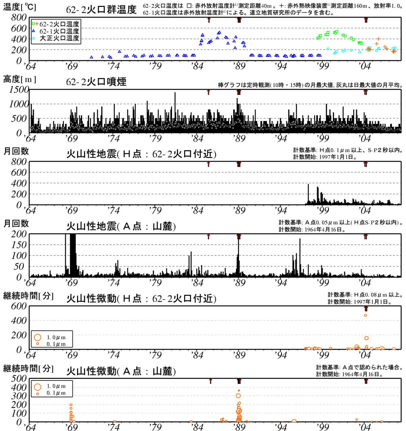
図 2※ 十勝岳 長期の火山活動経過図（1964 年 1 月～2008 年 5 月）
