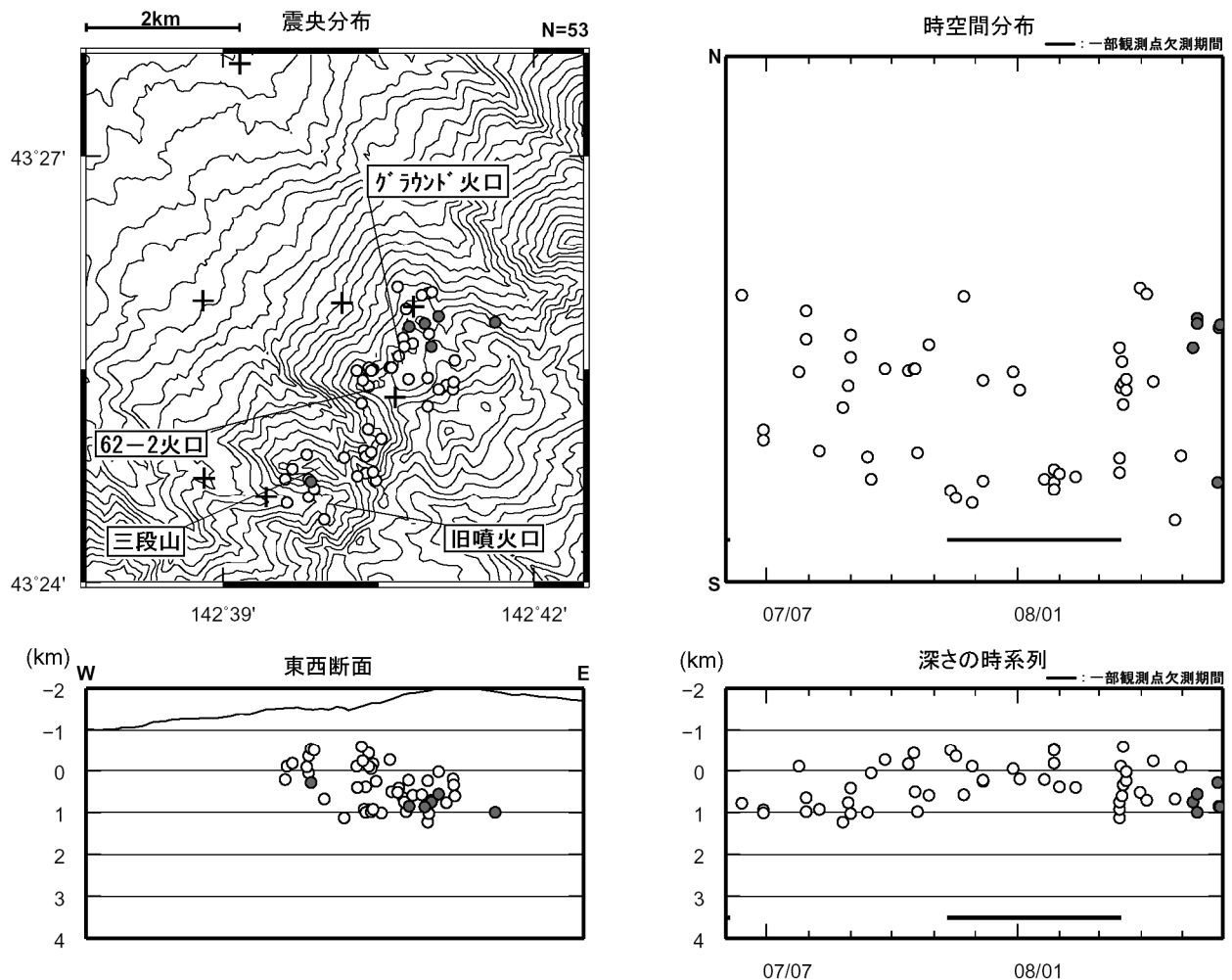
図 4 ※ 十勝岳 震源分布図（2007 年 6 月～2008 年 5 月、+は地震観測点）
