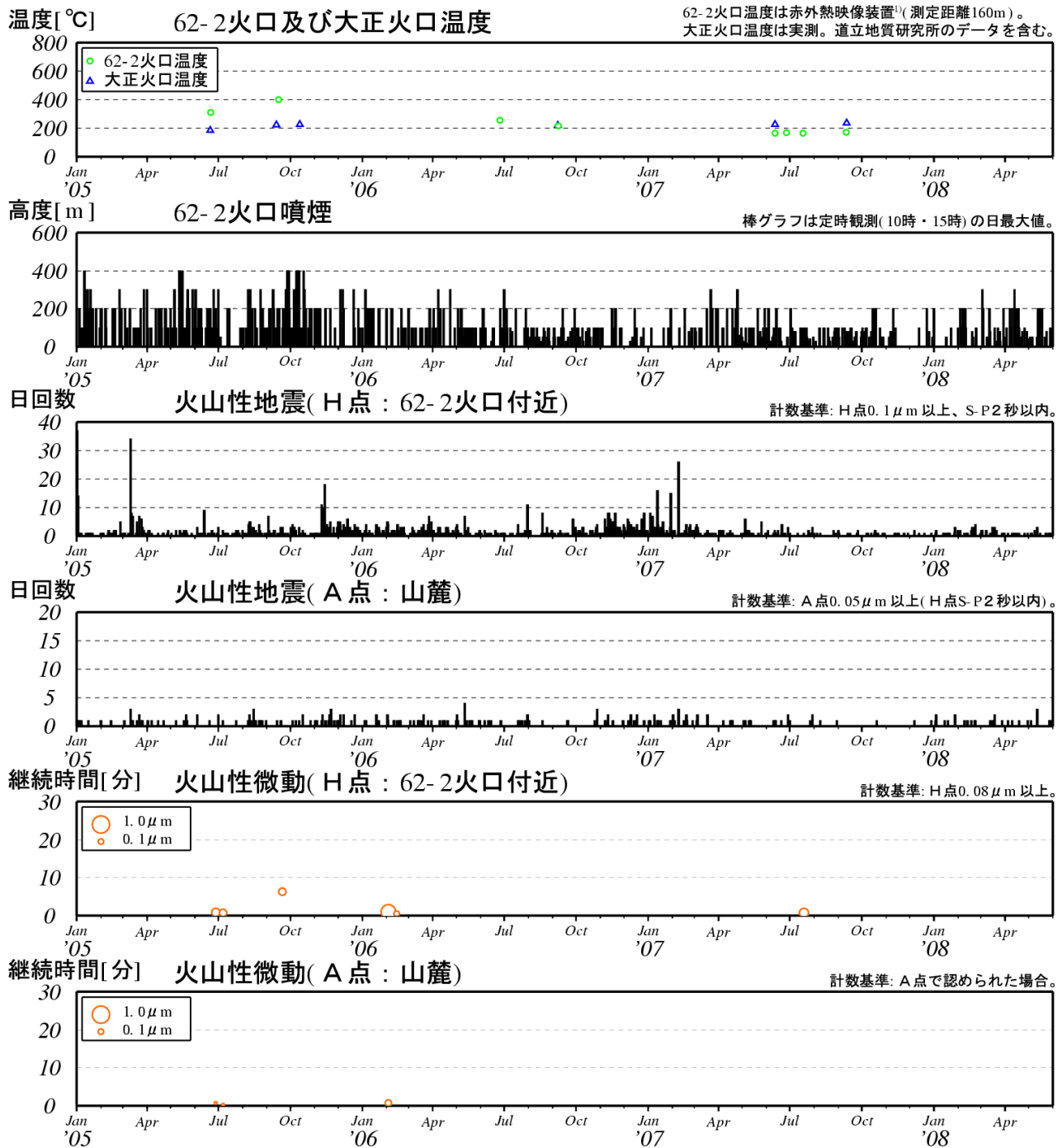
図 3 ※ 十勝岳 最近の火山活動経過図（2005 年 1 月～2008 年 5 月）
