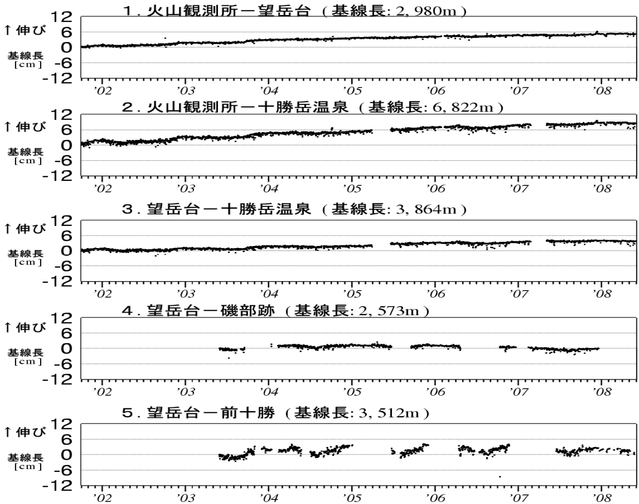
図5※ 十勝岳 GPS 連続観測による基線長変化（2001 年 10 月～2008 年 5 月） グラフの空白部分は欠測。
