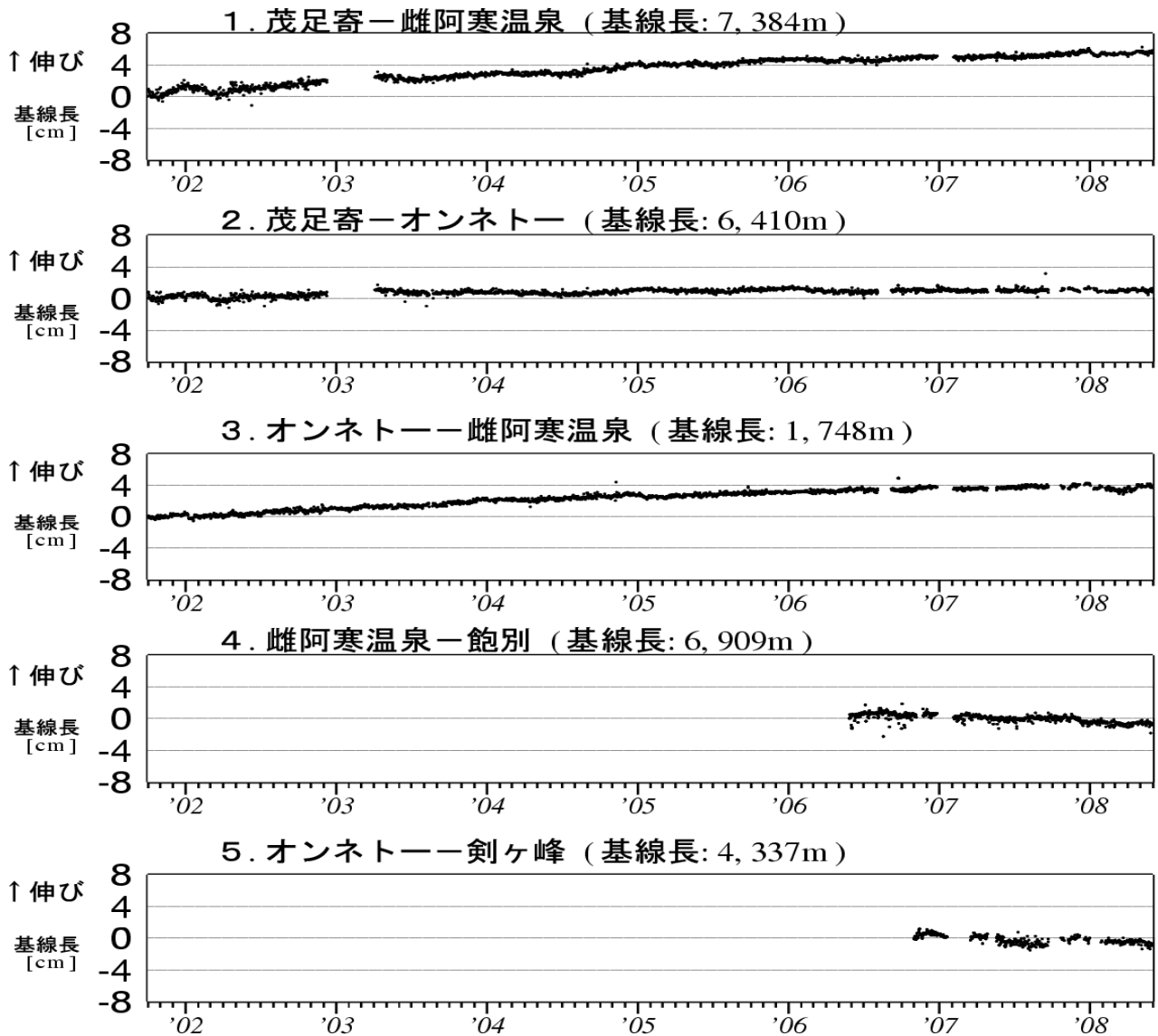
図5 雌阿寒岳 GPS 連続観測による基線長変化（2001 年 10 月～2008 年 5 月） グラフの空白部分は欠測 図5の1～5は、図6のGPS基線①～⑤に対応しています。
