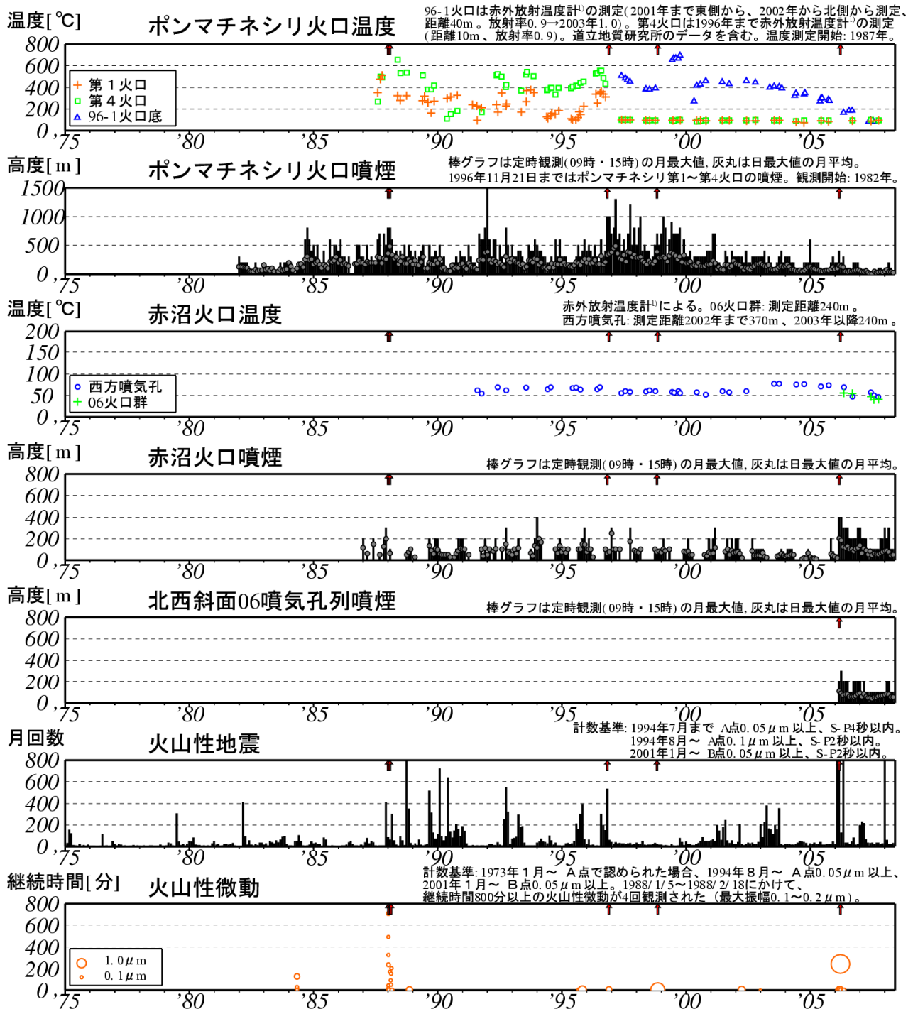
図2※ 雌阿寒岳 長期の火山活動経過図(1975年1月〜2008年5月) ↑印は噴火 (1988年、1996年、1998年:ポンマチネシリ火口からの噴火、2006年:赤沼火口からの噴火)
