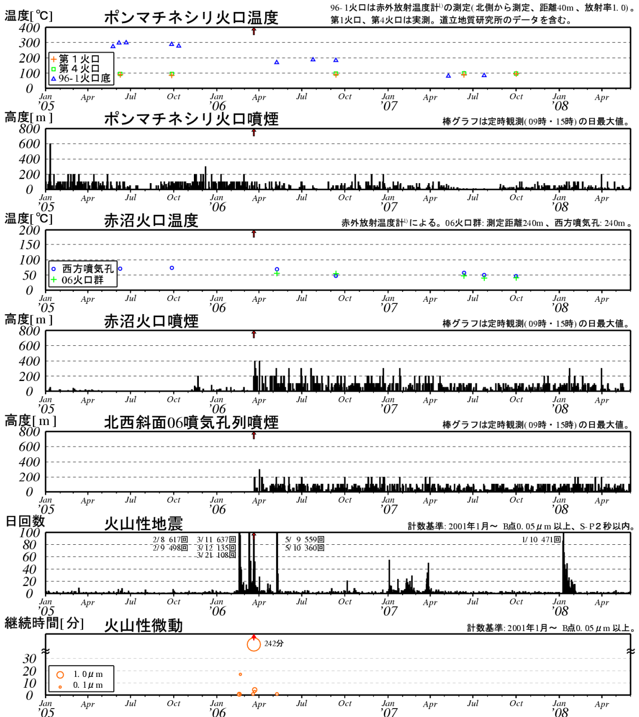
図3※ 雌阿寒岳 最近の火山活動経過図（2005年1月～2008年5月） ↑印は噴火
