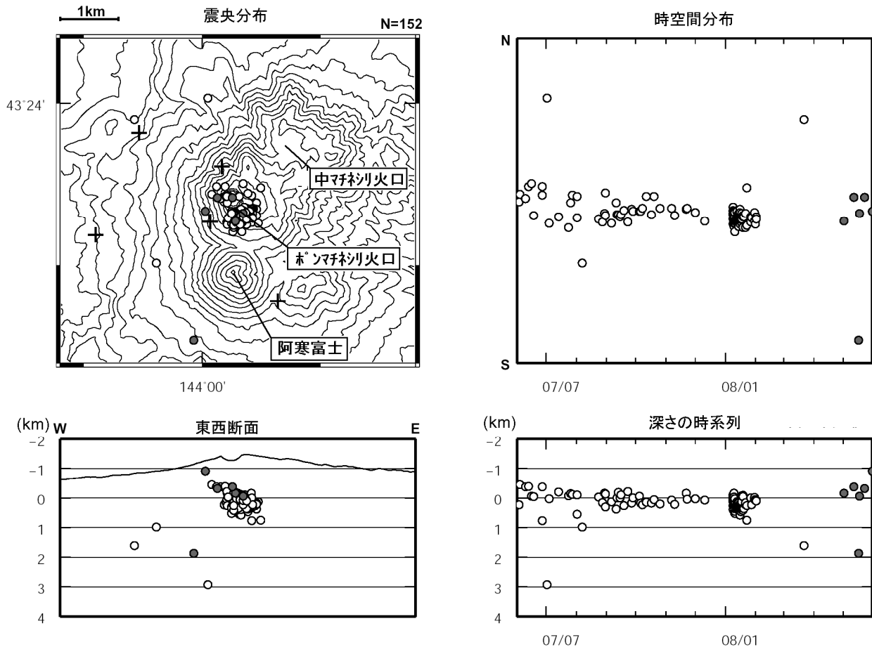
図 4 雌阿寒岳 震源分布図（2007 年 6 月～2008 年 5 月、+は地震観測点）
