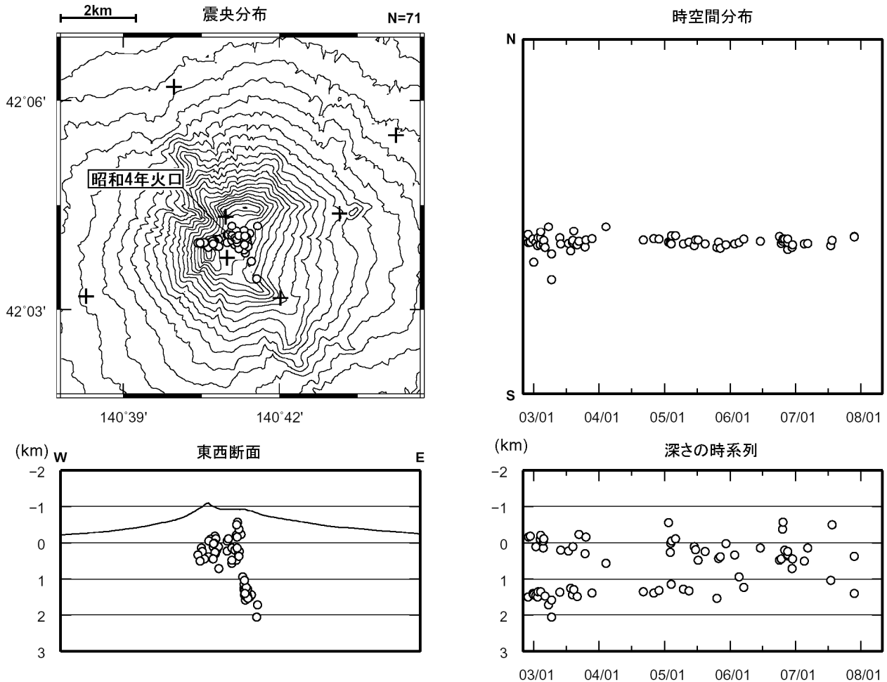
図 4 ※ 北海道駒ヶ岳 震源分布図（2002 年 11 月～2008 年 4 月、+は地震観測点）
