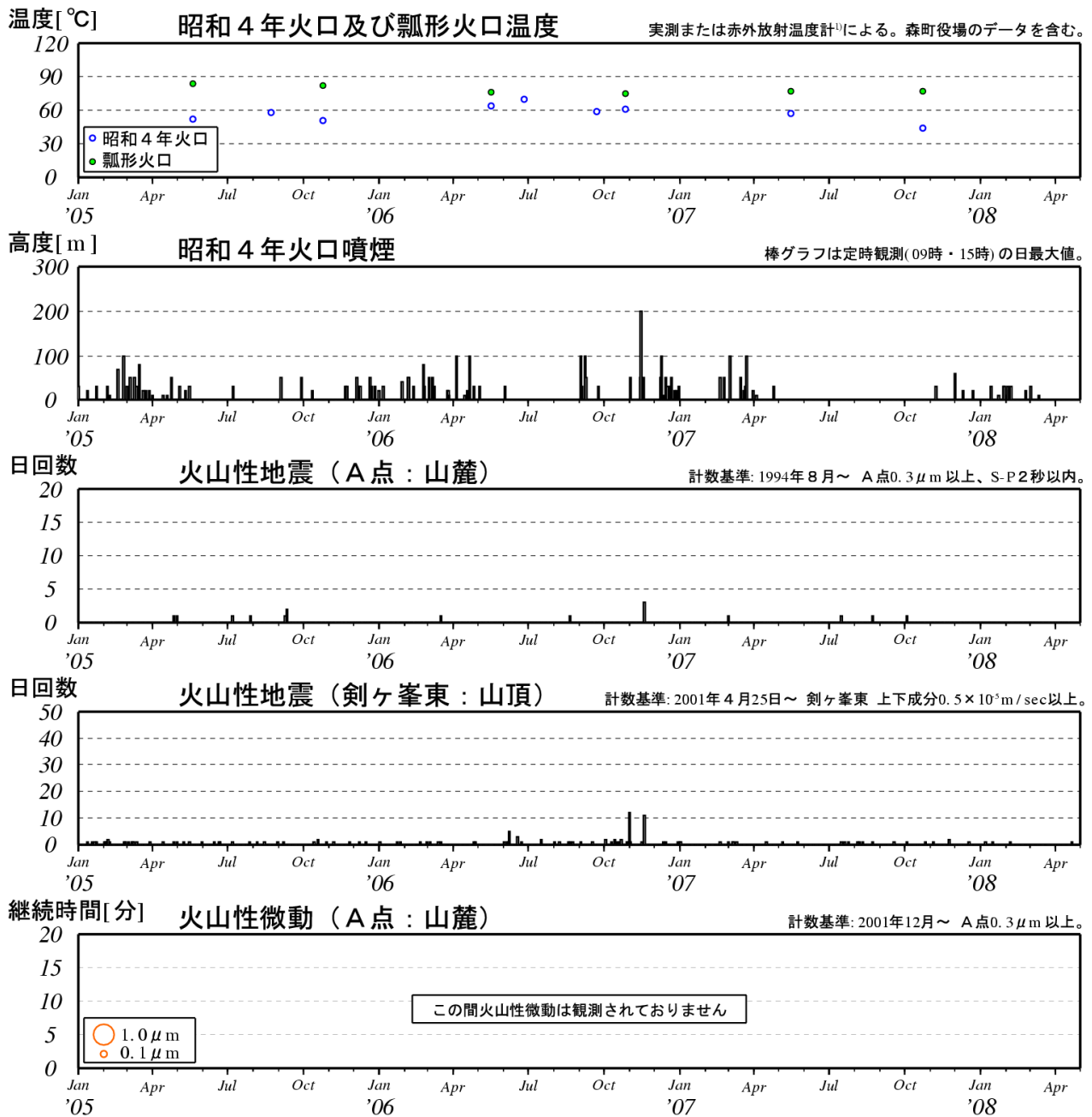
図 3※ 北海道駒ヶ岳 最近の火山活動経過図（2005 年 1 月～2008 年 4 月）
