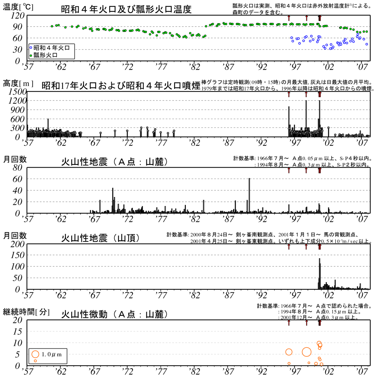
図 2 ※ 北海道駒ヶ岳 長期の火山活動経過図（1957 年 1 月～2008 年 4 月）↑印は噴火
