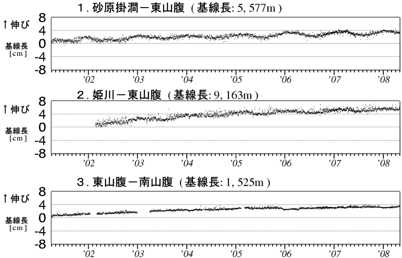
図 5 北海道駒ヶ岳 GPS 連続観測による基線長変化（2001 年 4 月～2008 年 4 月）
