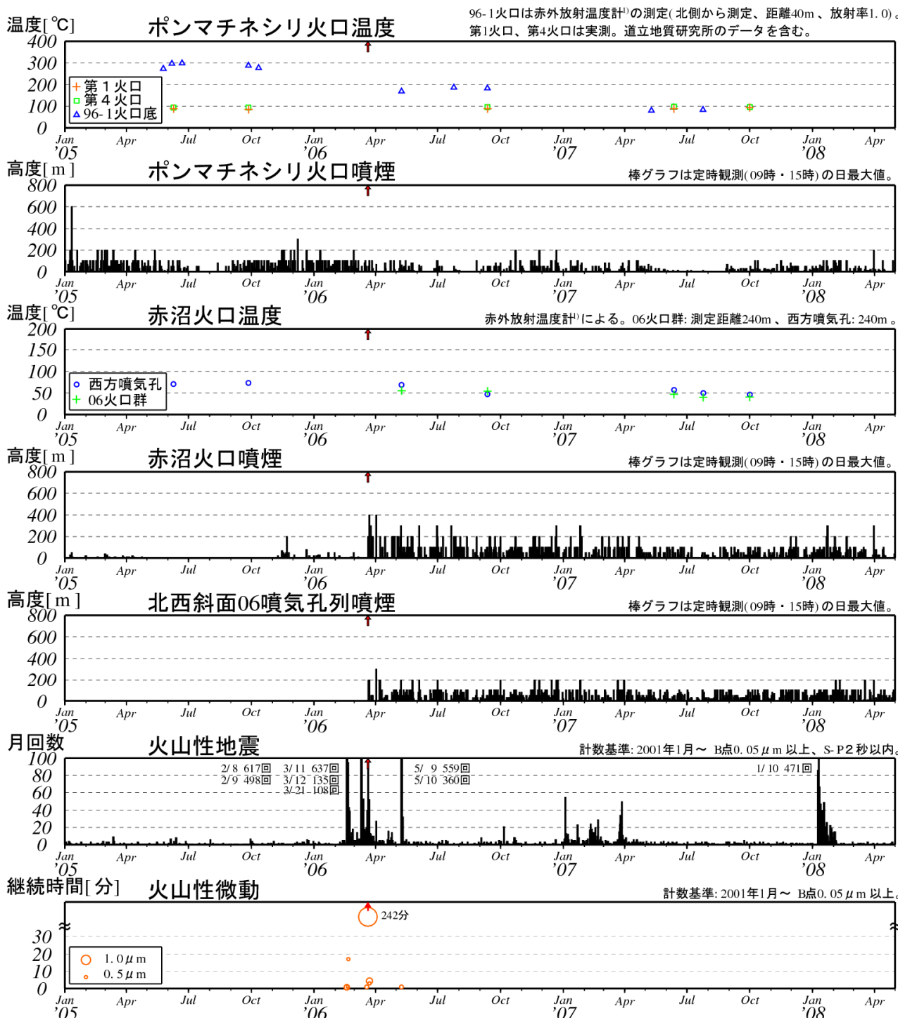
図3※ 雌阿寒岳 最近の火山活動経過図 (2005年1月～2008年4月) ↑印は噴火
