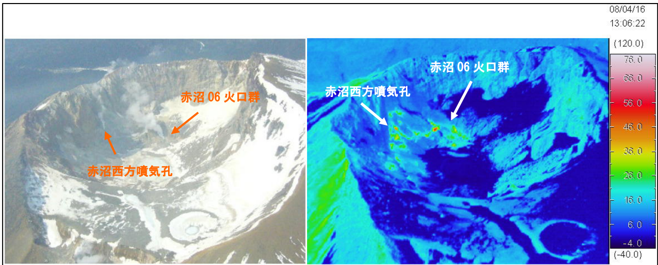
図4 雌阿寒岳 赤外熱映像装置 1) による赤沼火口付近の地表面温度分布 (2008年4月16日 図6の①方向上空より撮影)
