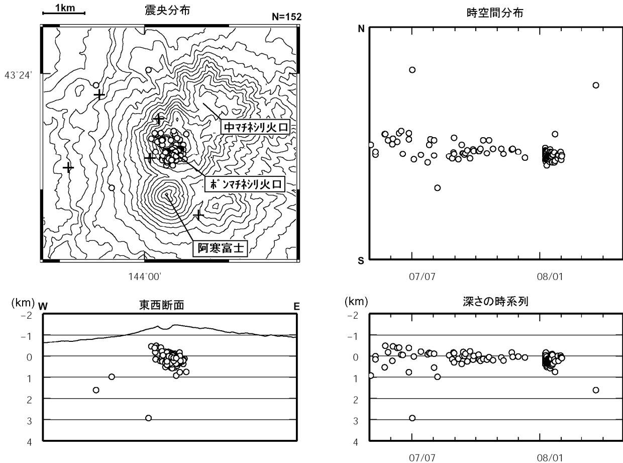
図 7 雌阿寒岳 震源分布図 (2007 年 5 月~2008 年 4 月、+は地震観測点) ○印は前期間までの 11 ヶ月間 (2007 年 5 月~2008 年 3 月) の震源 ・前期間までの震源の多くは、ポンマチネシリ火口直下の浅い所 (山頂から深さ 1~3 km 付近) に分布しています。今期間に求まった震源はありませんでした。
