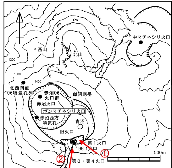
図6 雌阿寒岳 火口周辺図
