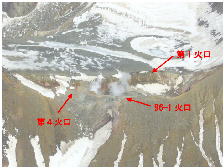
図5 雌阿寒岳 ポンマチネシリ火口の状況 (2008年4月16日 図6の②方向上空より撮影)
