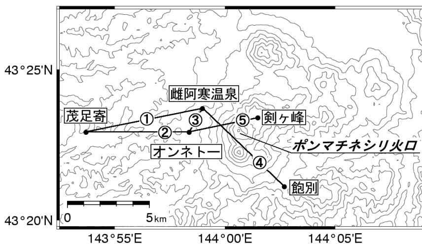
図 9 雌阿寒岳 GPS 連続観測点配置図
