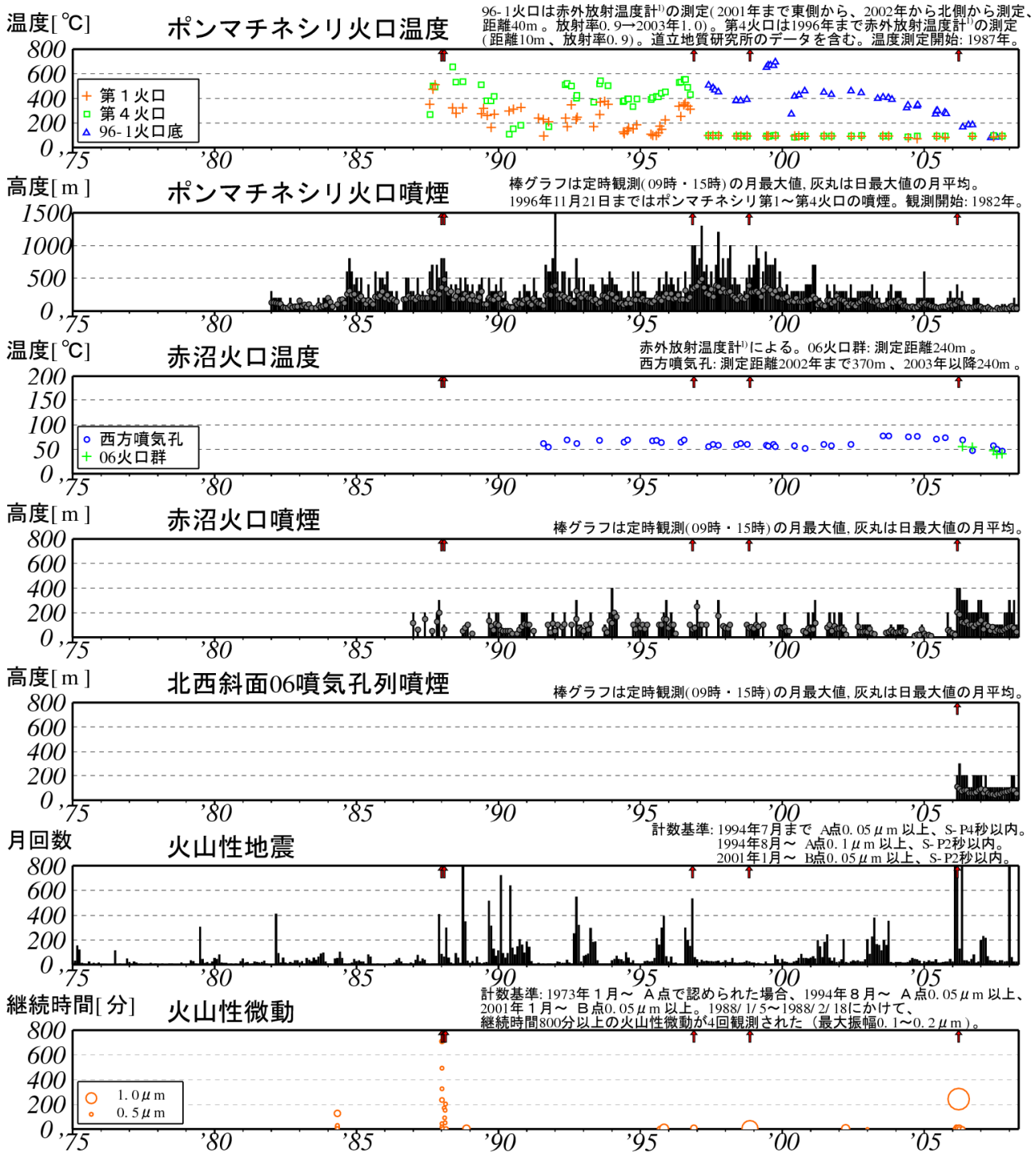
図2※ 雌阿寒岳 長期の火山活動経過図(1975年1月～2008年4月) ↑印は噴火 (1988年、1996年、1998年:ポンマチネシリ火口からの噴火、2006年:赤沼火口からの噴火)
