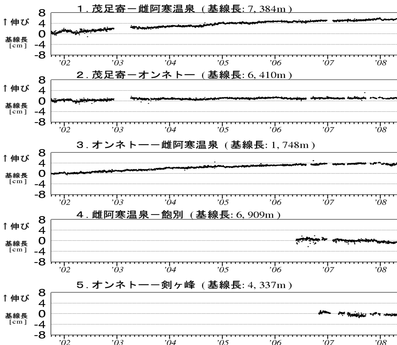
図 8 雌阿寒岳 GPS 連続観測による基線長変化 (2001 年 10 月～2008 年 4 月) グラフの空白部分は欠測 図 8 の 1～5 は、図 9 の GPS 基線①～⑤に対応しています。
