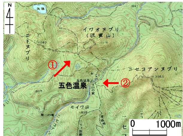
図 2 ニセコ 周辺図
