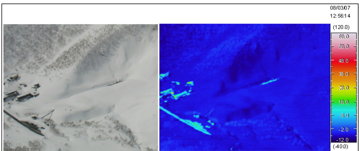
図 3 ニセコ 赤外熱映像装置 1) による五色温泉付近の地表面温度分布 (2008 年 3 月 7 日 図 2 の②方向上空より撮影)
