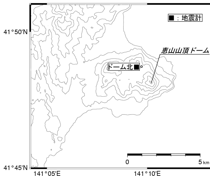
図 2 恵山 地震計配置図
