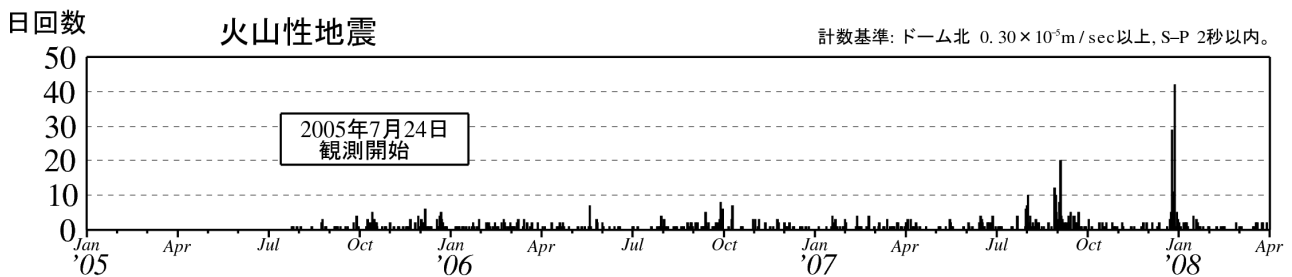
図 1 恵山 日別地震回数（2005 年 7 月～2008 年 3 月）
