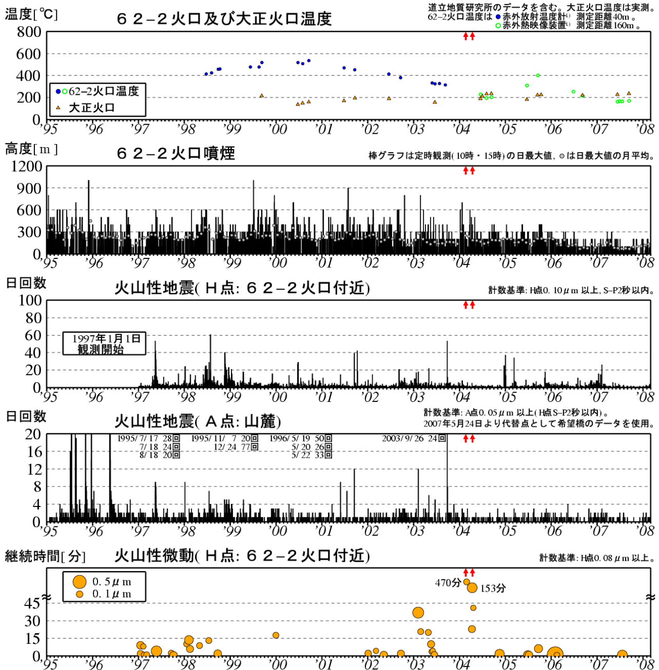
図 2※ 十勝岳 最近の火山活動経過図（1995 年 1 月～2008 年 2 月） ↑印はごく小規模な噴火
