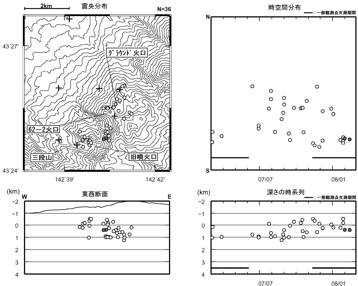
図 3※ 十勝岳 震源分布図（2007 年 3 月～2008 年 2 月、+は地震観測点）
