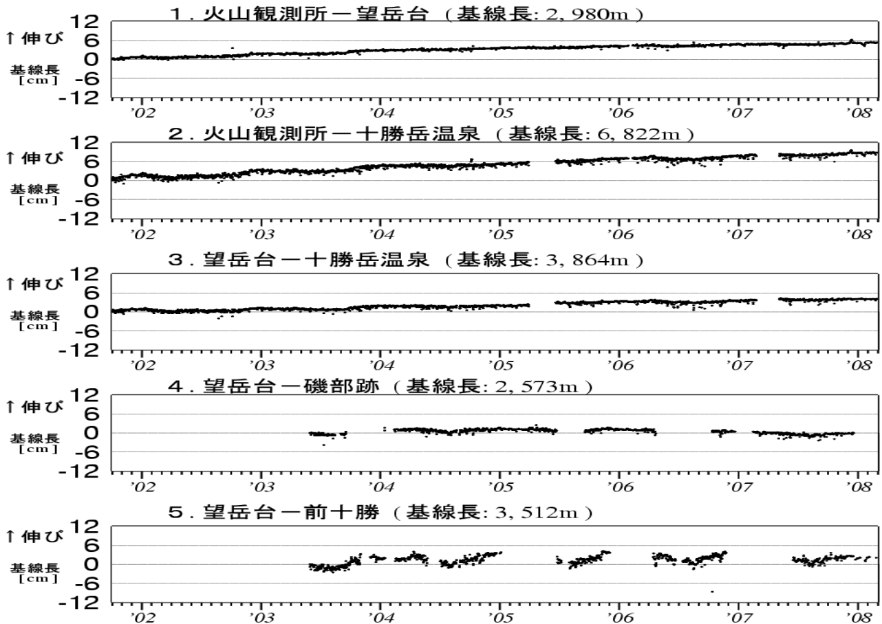
図 4※ 十勝岳 GPS 連続観測による基線長変化（2001 年 10 月～2008 年 2 月） グラフの空白部分は欠測。
