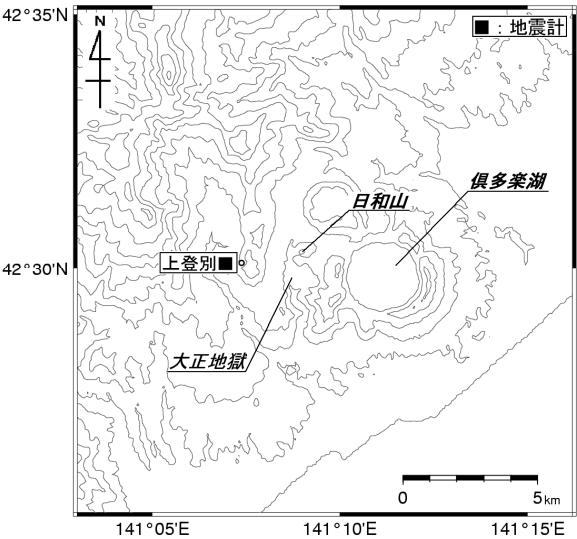
図 2 倶多楽 地震計配置図
