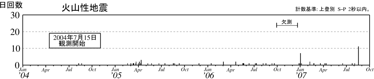
図 1 倶多楽 日別地震回数（2004 年 7 月～2007 年 9 月）
