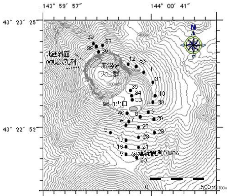
図 3 雌阿寒岳 全磁力連続観測点 MEA（図中の◎印） と繰り返し観測点（図中の●印）配置図 図 4 の番号は図 3 の観測点番号に対応しています。
