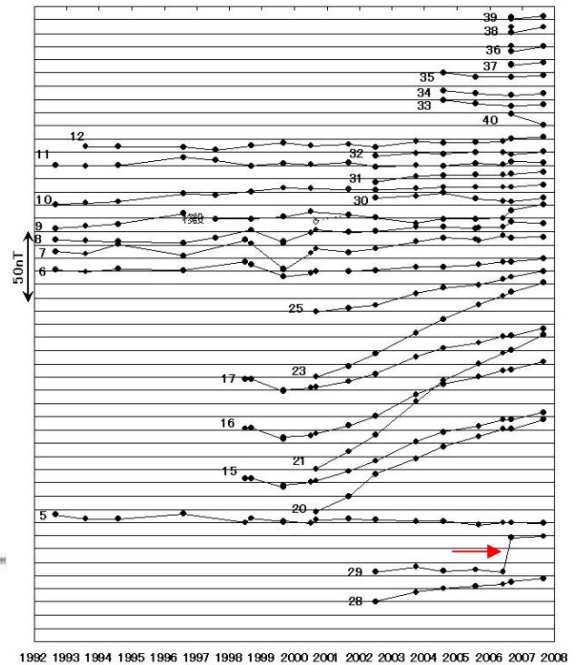
図 4 雌阿寒岳 全磁力繰返し観測結果 （1992 年～2007 年）
