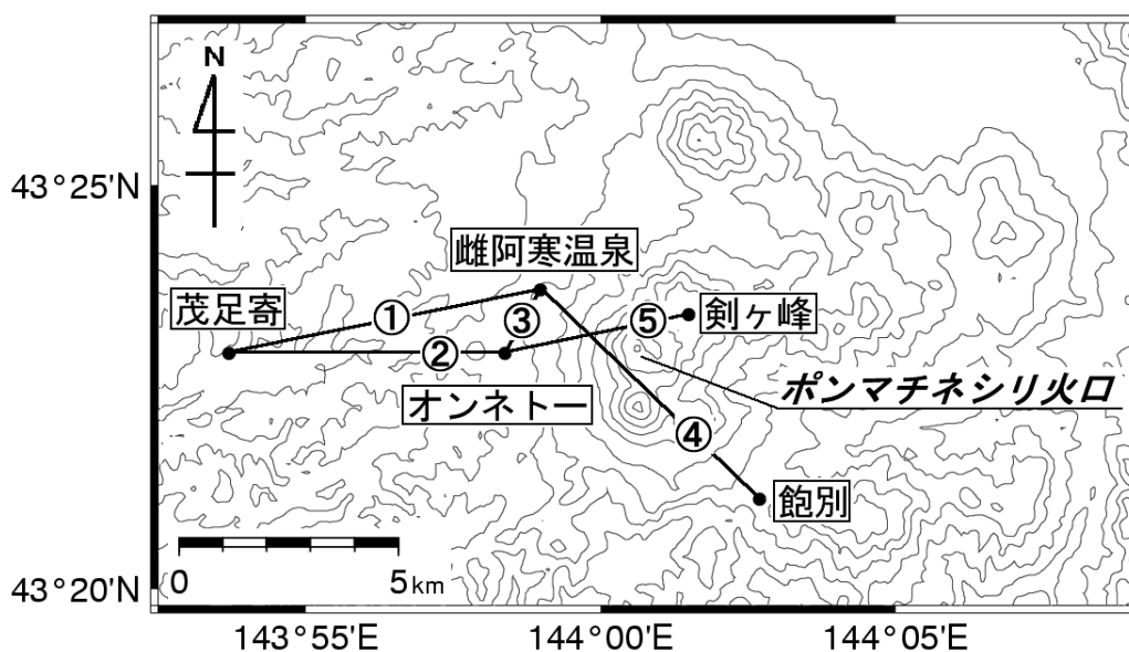
図8 雌阿寒岳 GPS 連続観測点配置図
