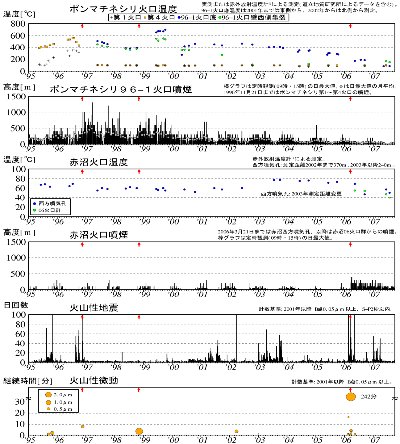
図 2※ 雌阿寒岳 最近の火山活動経過図 (1995 年 1 月～2007 年 9 月) ↑印は噴火
