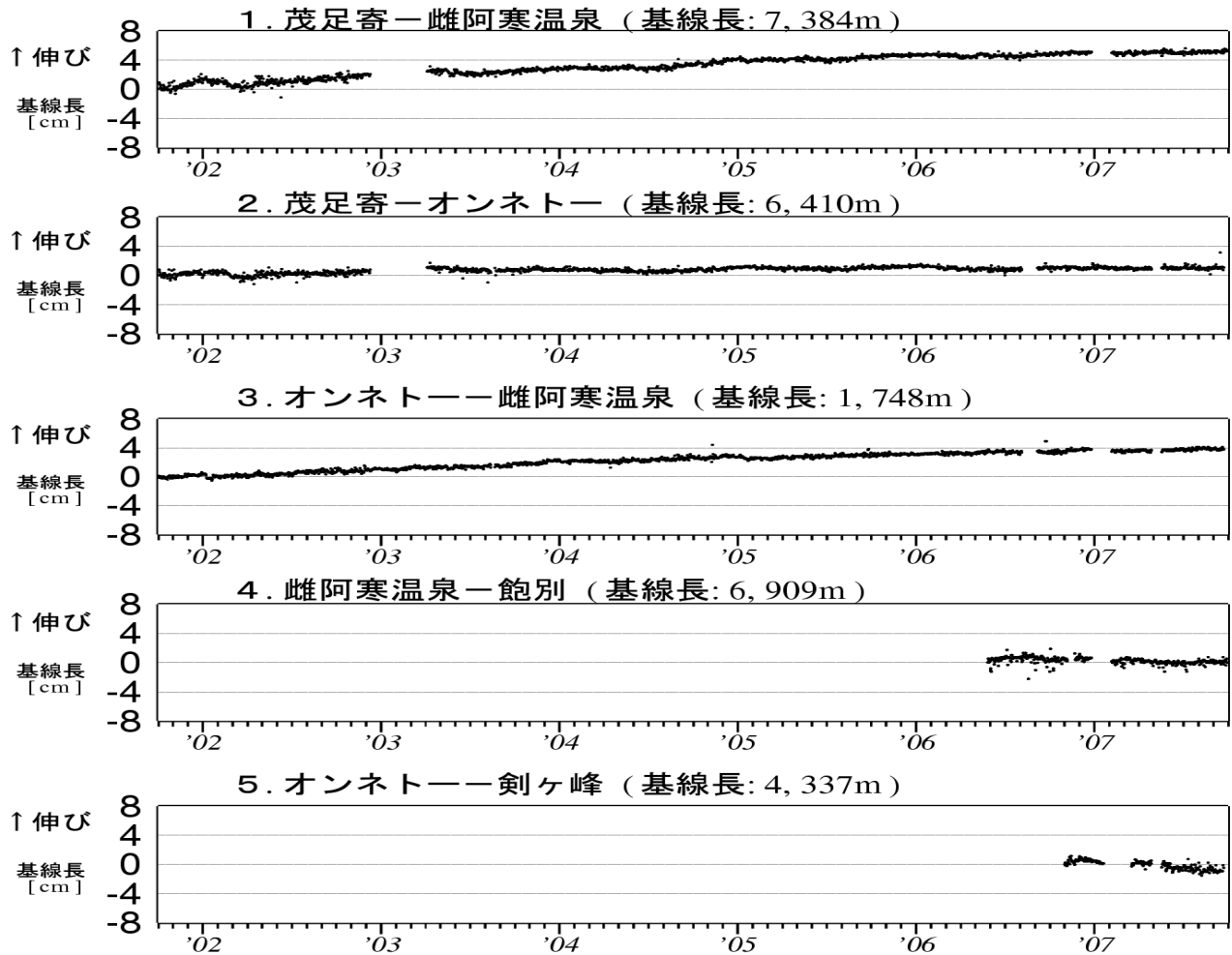
図7 雌阿寒岳 GPS 連続観測による基線長変化 （2001 年 10 月～2007 年 9 月）グラフの空白部分は欠測 図7の1～5は、図8のGPS基線①～⑤に対応しています。
