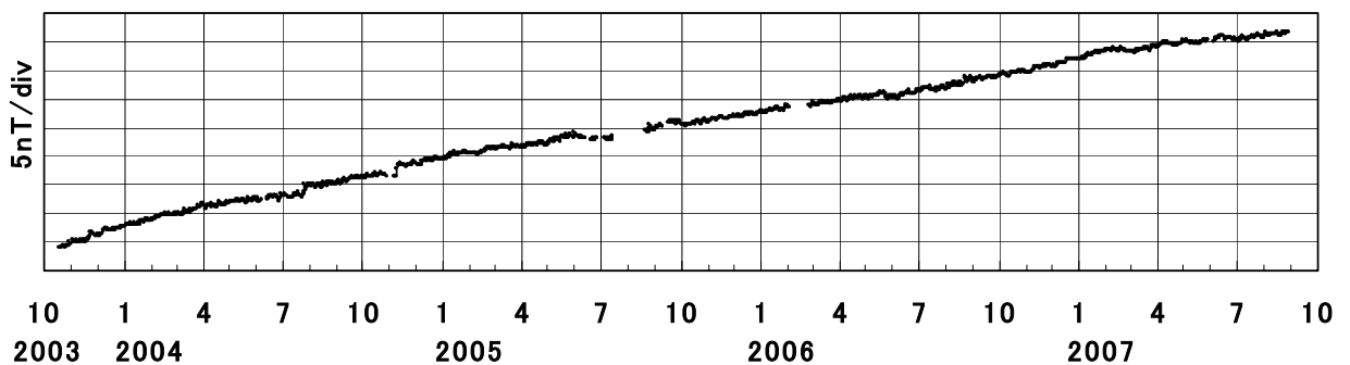
図 5 雌阿寒岳 全磁力連続観測結果 2) （2003 年 10 月～2007 年 9 月）
