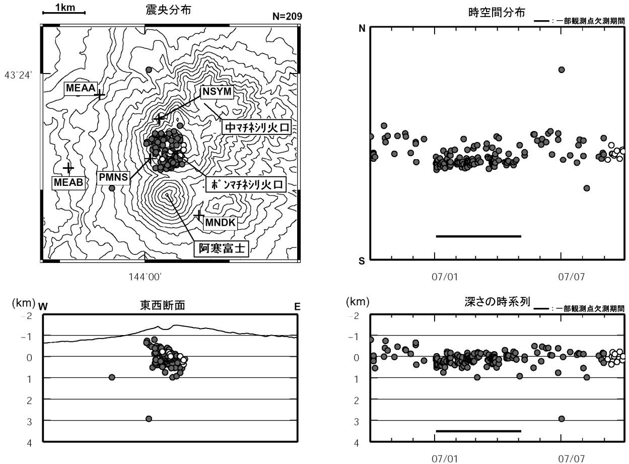
図 6 雌阿寒岳 震源分布図(2006 年 10 月～2007 年 9 月、+は地震観測点)
