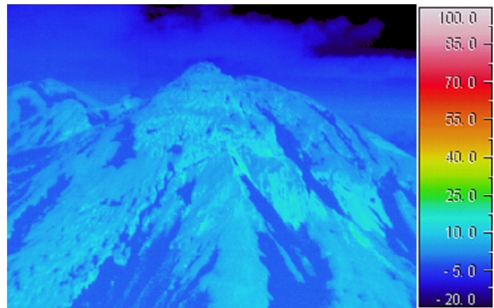
図 3 羅臼岳 赤外熱映像装置*による羅臼岳山頂部の表面温度分布 (2007 年 5 月 14 日 図 2 ②方向から撮影)
