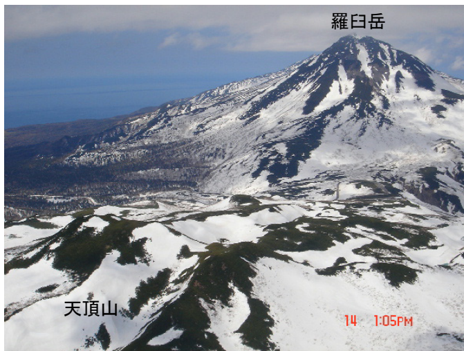
図 1 羅臼岳 南側上空から撮影した羅臼岳 (2007 年 5 月 14 日 図 2 ①方向より撮影)
