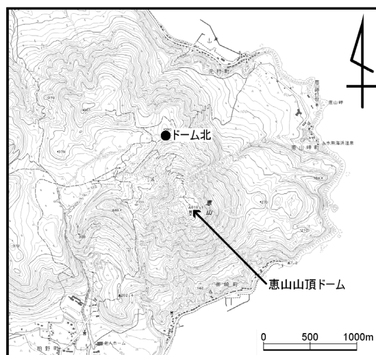
図2 恵山 地震計配置図 (図中●)
