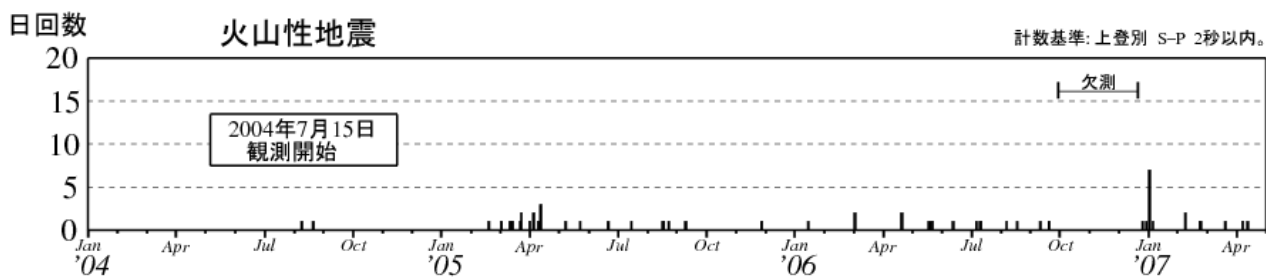
図 1 倶多楽 日別地震回数 (2004年7月15日~2007年4月30日)
