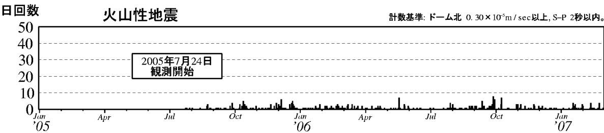
図 1 恵山 日別地震回数（2005 年 7 月 24 日～2007 年 2 月 28 日）
