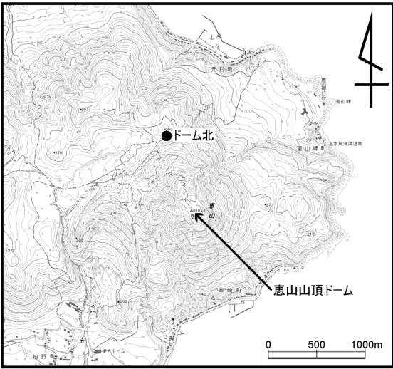
図 2 恵山 地震計配置図（図中●）
