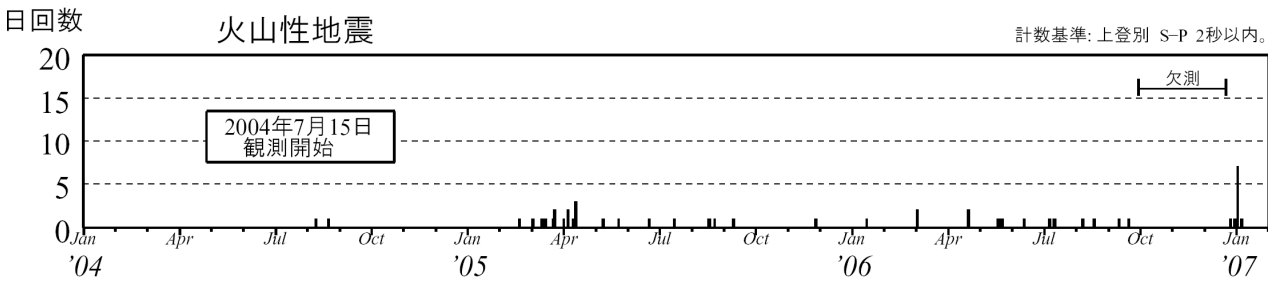
図 1 倶多楽 日別地震回数（2004 年 7 月 15 日～2007 年 1 月 31 日）
