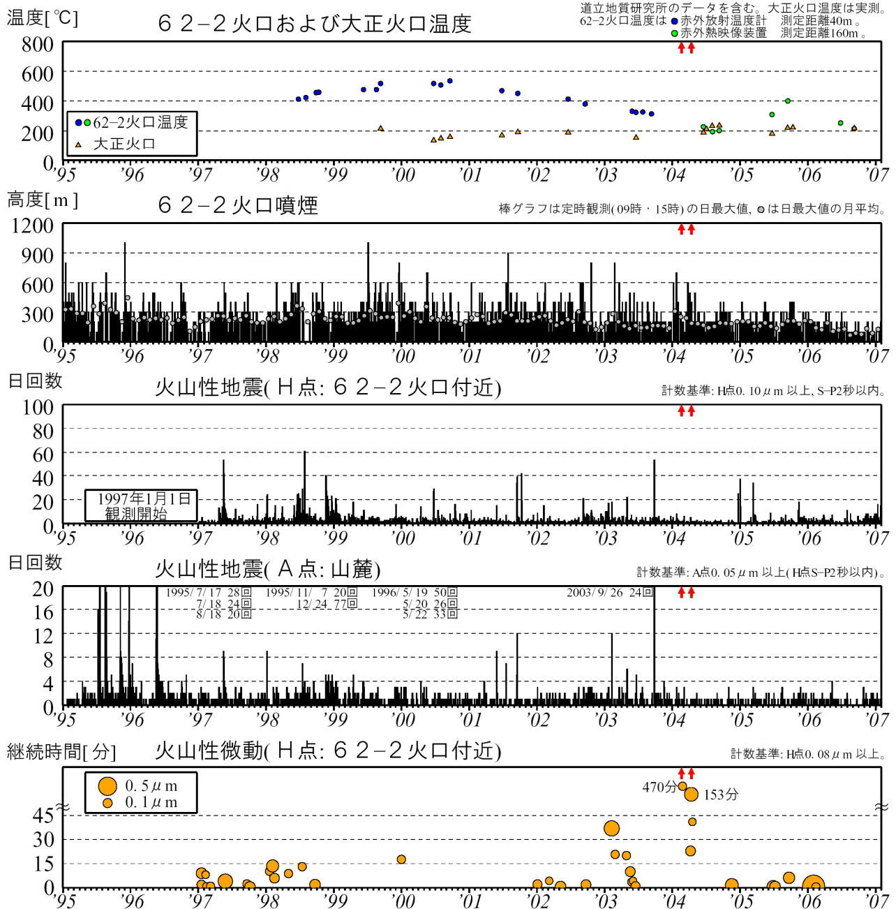
図 2※ 十勝岳 最近の火山活動経過図（1995 年 1 月～2007 年 1 月） ↑印はごく小規模な噴火 ・ 62-2 火口の噴煙活動はやや活発な状態が続いていますが、2006 年 1 月以降低下傾向が見られます。 ・ 地震活動は 1999 年後半から比較的静穏に経過しています。火山性微動は 2006 年 2 月 15 日以降発生していません。
