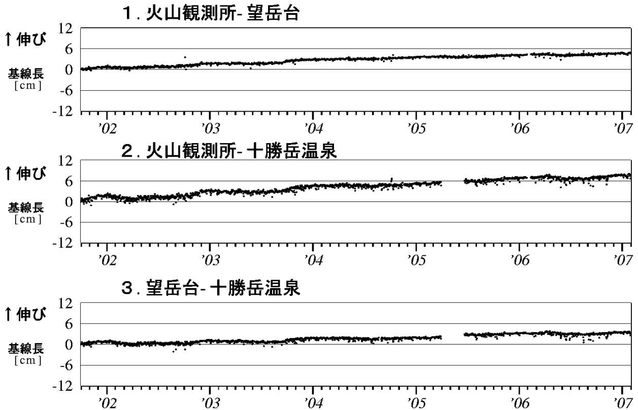
図 4 十勝岳 GPS 連続観測による基線長変化（2001 年 10 月～2007 年 1 月）
