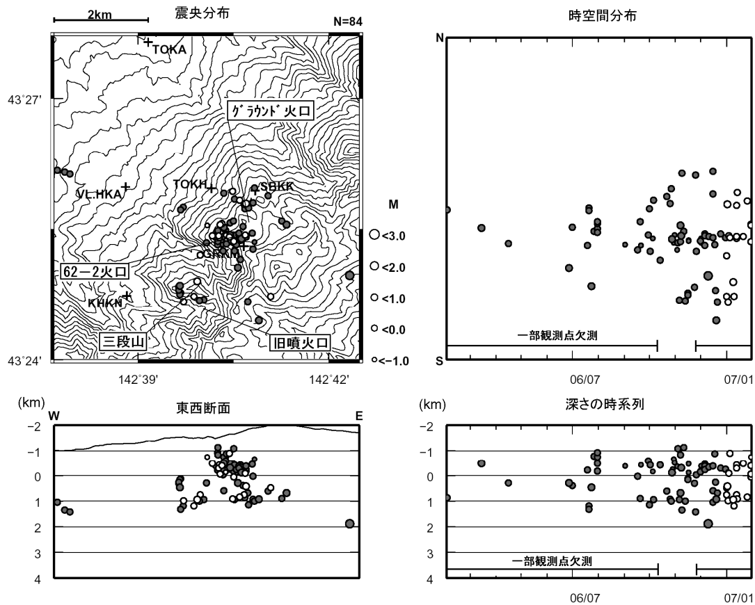
図 3※ 十勝岳の震源分布図（2006 年 2 月 1 日～2007 年 1 月 31 日、+は地震観測点）
