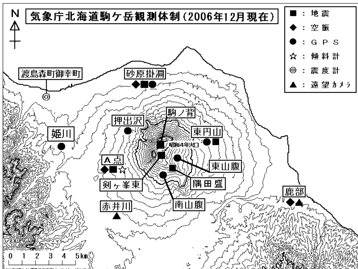
図 1 北海道駒ヶ岳火山観測点配置図
