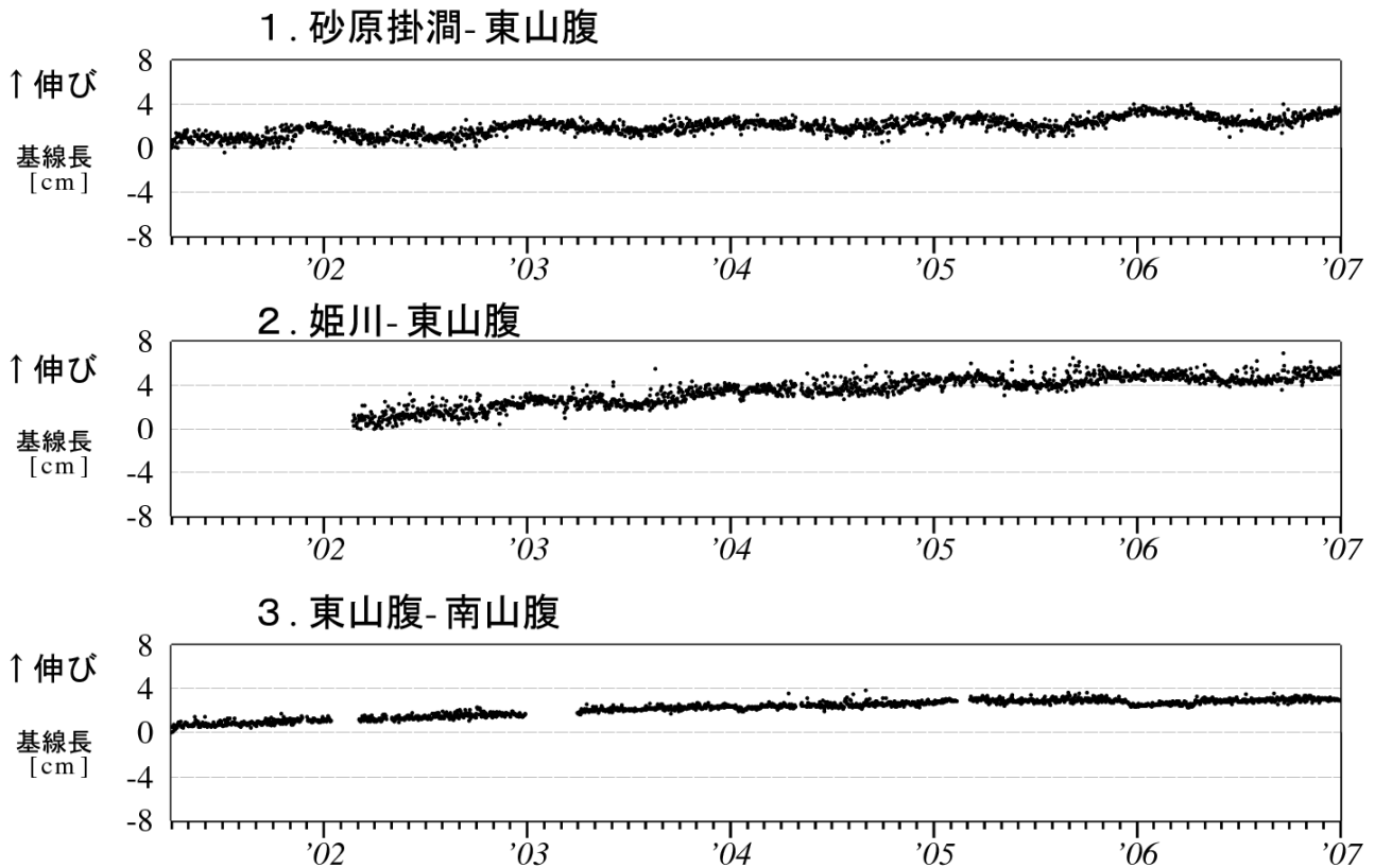
図 4 北海道駒ヶ岳 GPS 連続観測による基線長変化（2001 年 4 月～2006 年 12 月）
