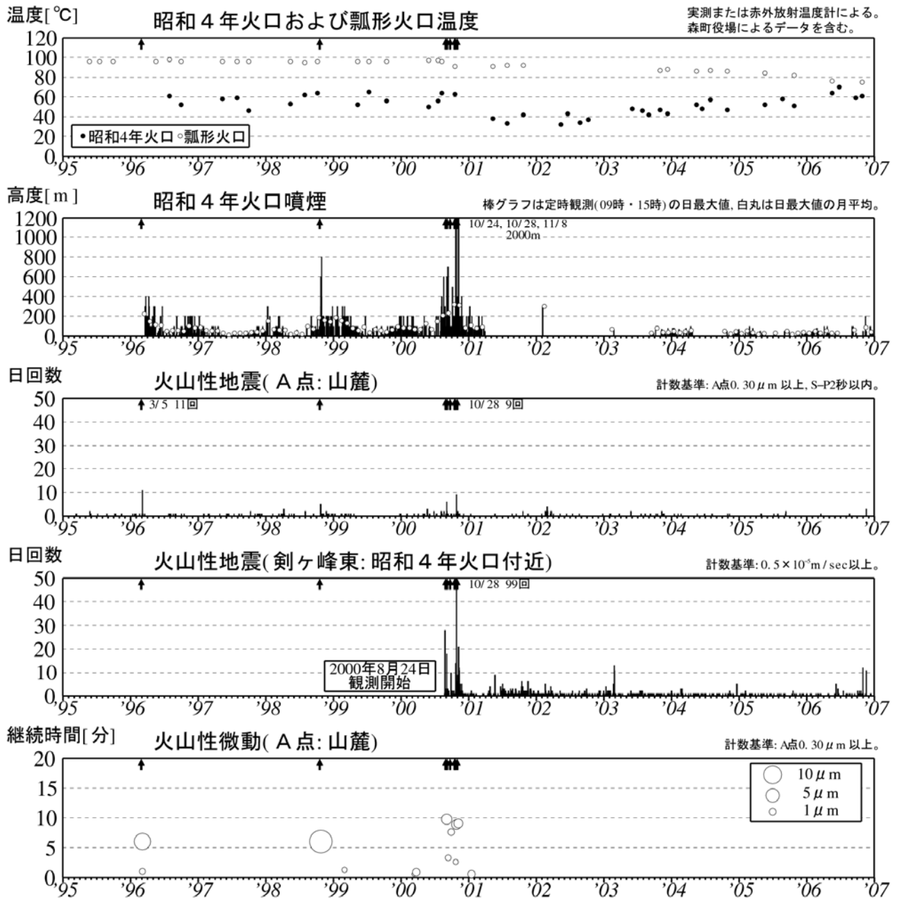
図 2 北海道駒ヶ岳 最近の火山活動経過図（1995 年 1 月～2006 年 12 月）↑印は噴火 ・昭和 4 年火口では 2003 年 9 月以降 10～50m 程度の噴煙が時折観測されています。 ・昭和 4 年火口の火口温度は、2002 年以降緩やかな上昇傾向が認められています。
