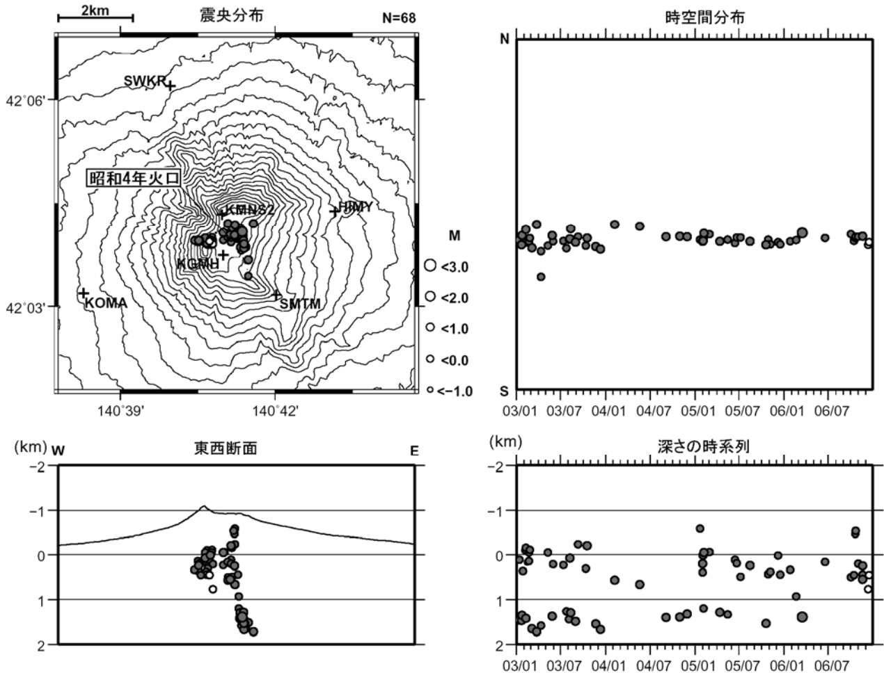
図 3 北海道駒ヶ岳の震源分布図（2003 年 1 月～2006 年 12 月、+は地震観測点）
