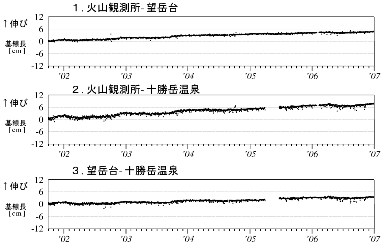
図 4 十勝岳 GPS 連続観測による基線長変化（2001 年 10 月～2006 年 12 月）
