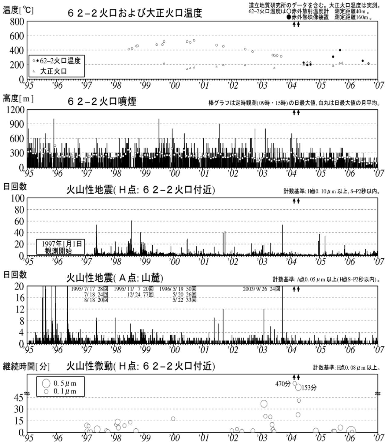
図2 十勝岳 最近の火山活動経過図（1995 年 1 月～2006 年 12 月） ↑印はごく小規模な噴火 ・62-2 火口の噴煙活動はやや活発な状態が続いていますが、2006 年 1 月以降低下傾向が見られます。 ・地震活動は 1999 年後半から比較的静穏に経過しています。火山性微動は 2006 年 2 月 15 日以降発生していません。
