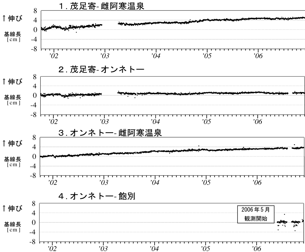
図 4 雌阿寒岳 GPS 連続観測による基線長変化（2001 年 9 月～2006 年 11 月）
