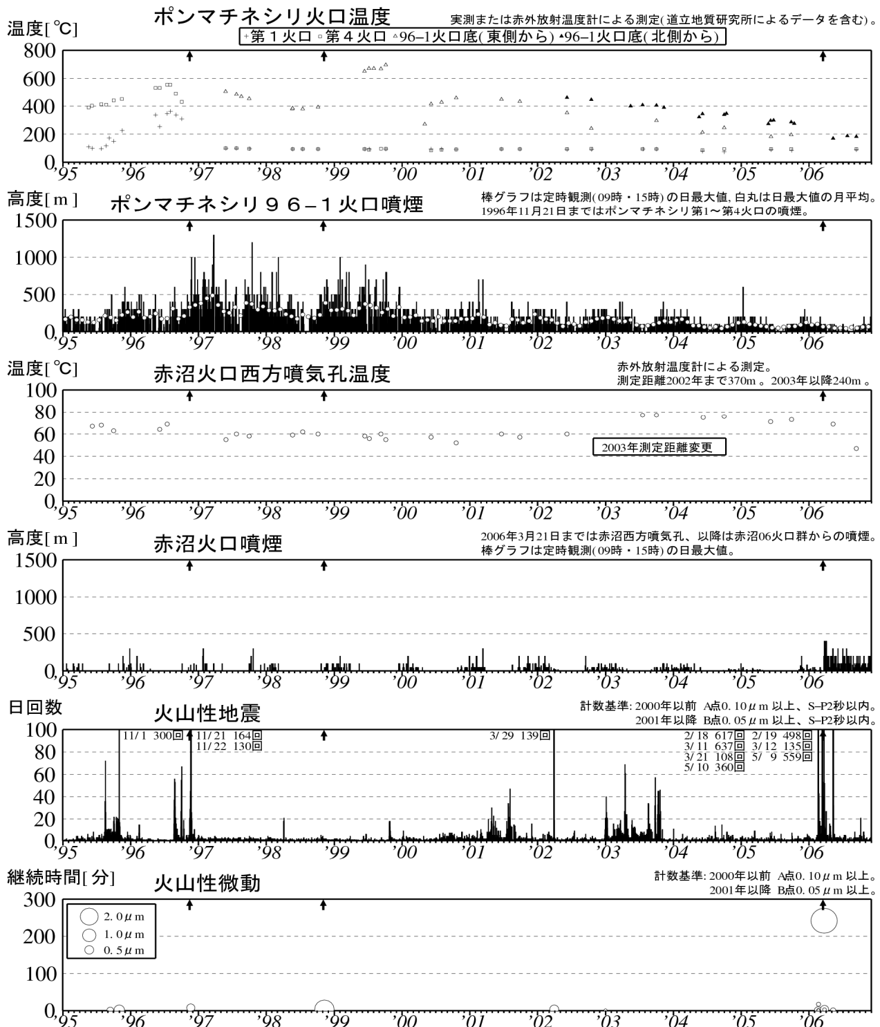
図2 雌阿寒岳 最近の火山活動経過図(1995年1月～2006年11月) ↑印は噴火 (1996年、1998年: ポンマチネシリ 96-1 火口からの噴火、2006年: 赤沼火口からの噴火)
