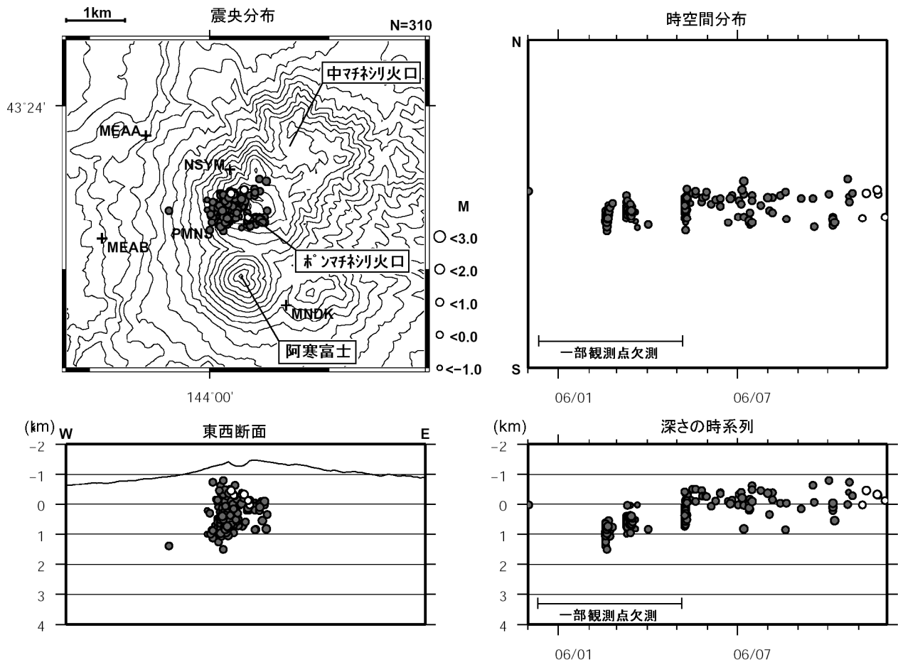
図 3 雌阿寒岳 震源分布図(2005 年 12 月～2006 年 11 月、+は地震観測点)
