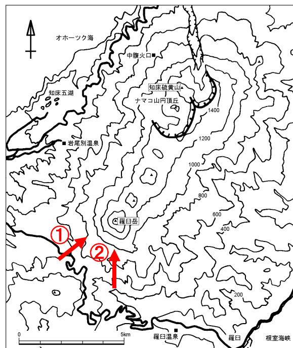
図 3 羅臼岳 火口周辺図
