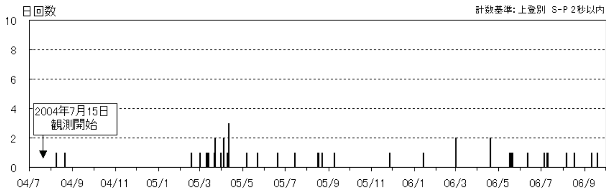
図1 倶多楽 日別地震回数（2004年7月15日～2006年9月30日）
