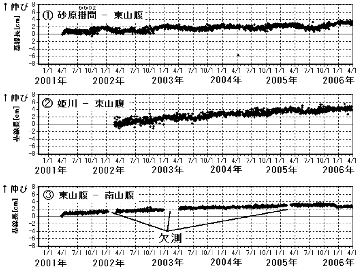
基線長変化 (2001 年 3 月 23 日～2006 年 3 月 31 日)
