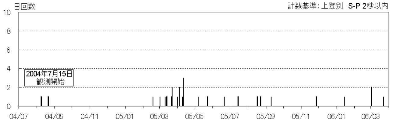
日別地震回数（2004 年 7 月 15 日～2006 年 3 月 31 日）
