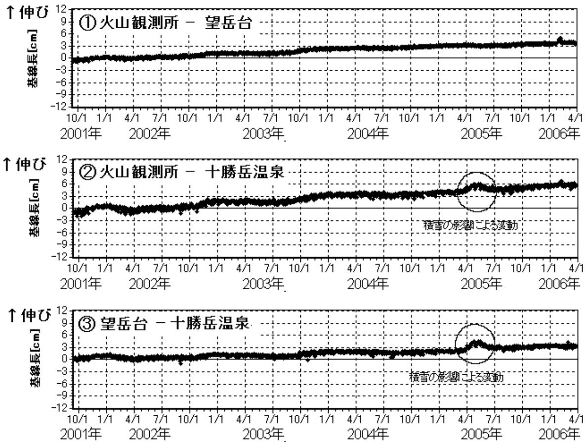
基線長変化（2001 年 9 月 13 日～2006 年 3 月 31 日）
