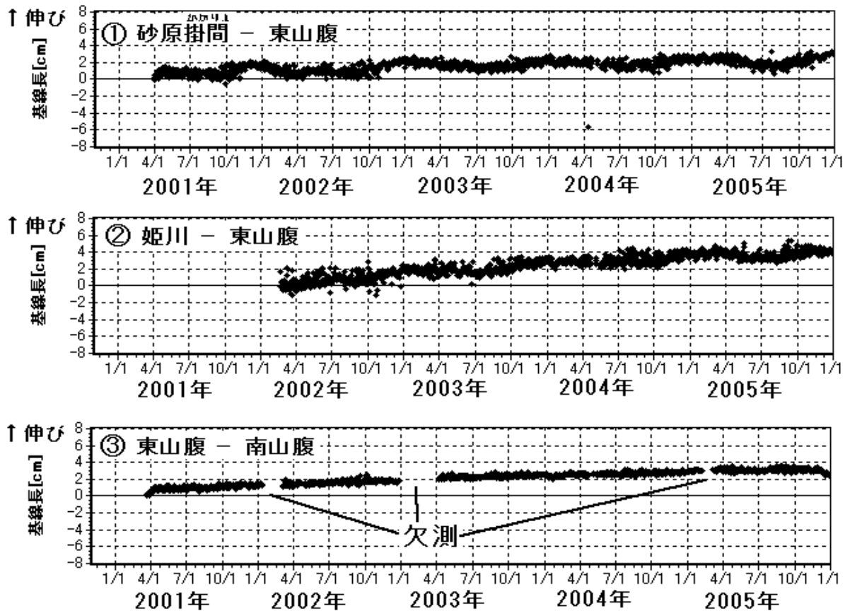
基線長変化（2001 年 3 月 23 日～2005 年 12 月 31 日）
