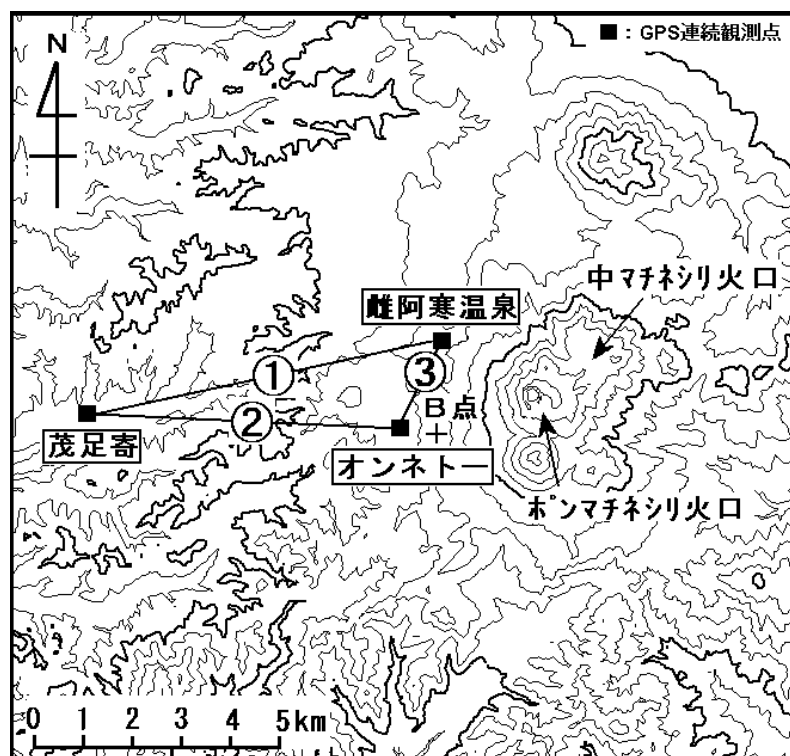
基線長変化（2001年9月19日～2005年6月30日）
