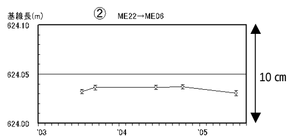
ポンマチネシリ火口周辺の基線長変化
