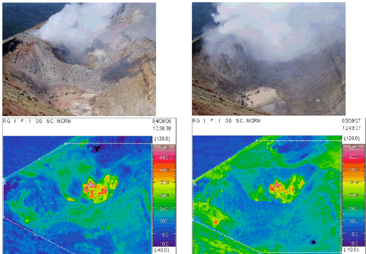
赤外熱映像装置による 96-1 火口及び第 1 火口の表面温度分布 （左：2004 年 6 月 6 日 右：2005 年 6 月 7 日）
