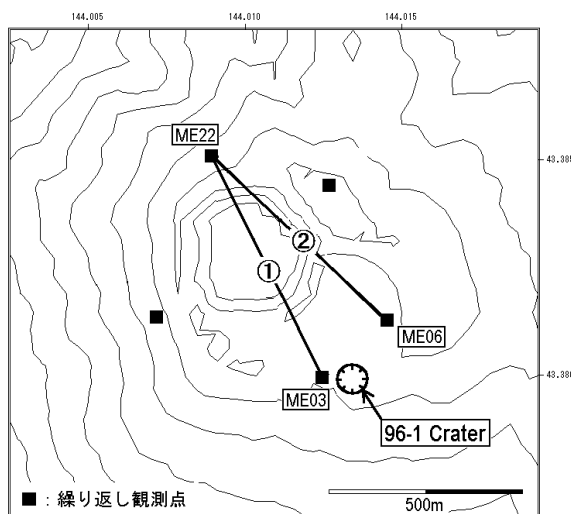
山頂 GPS 繰り返し観測位置
