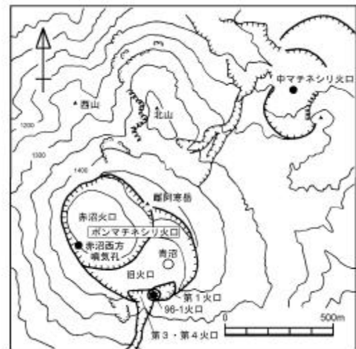
雌阿寒岳火口周辺図
