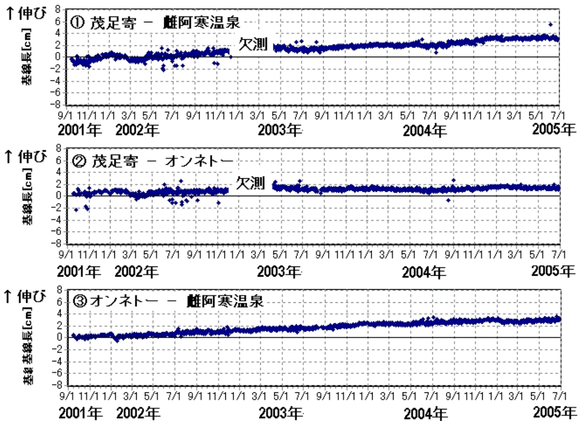
基線長変化（2001年9月19日～2005年6月30日）
