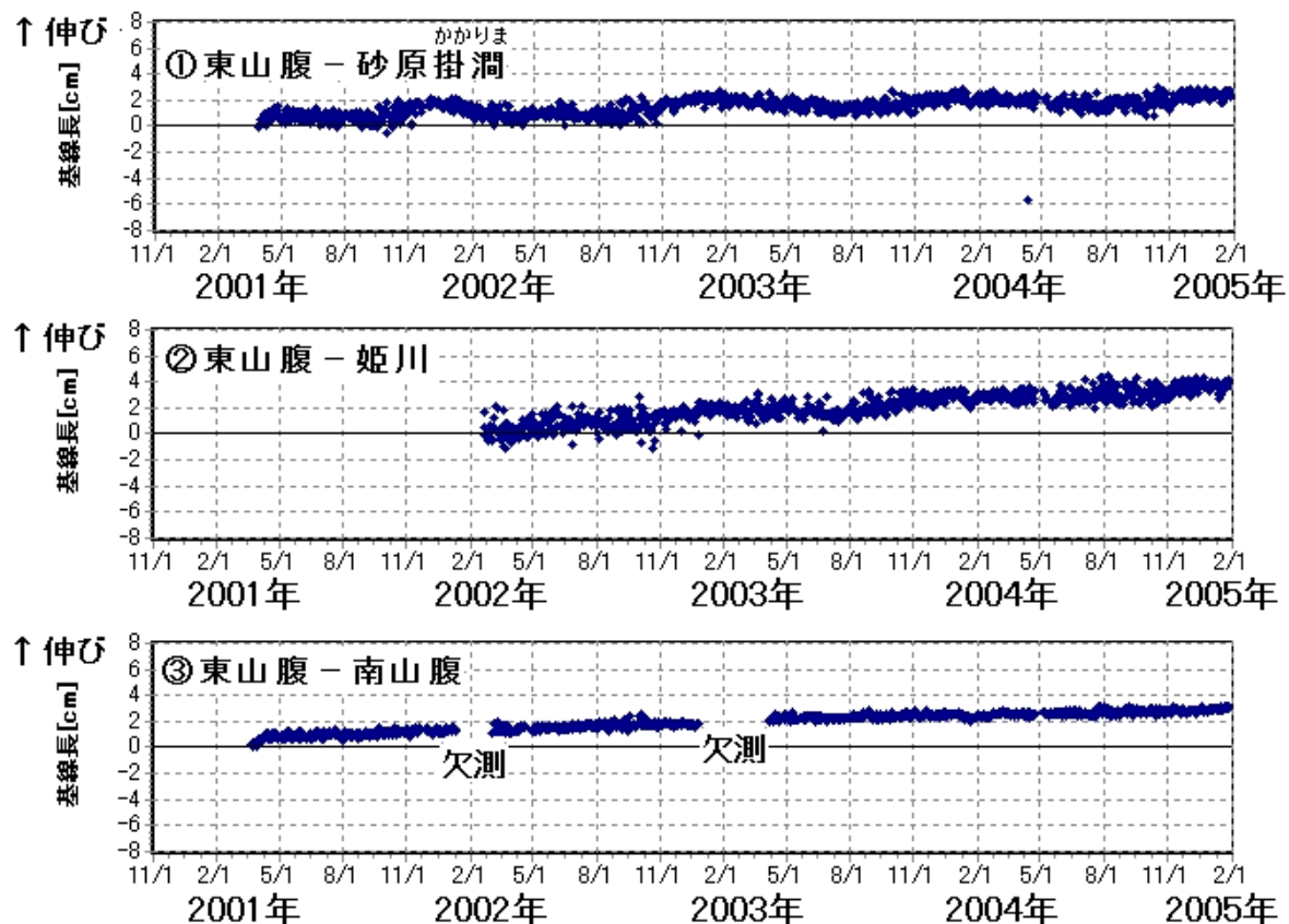
基線長変化（2001 年 3 月 23 日～2005 年 1 月 31 日）
