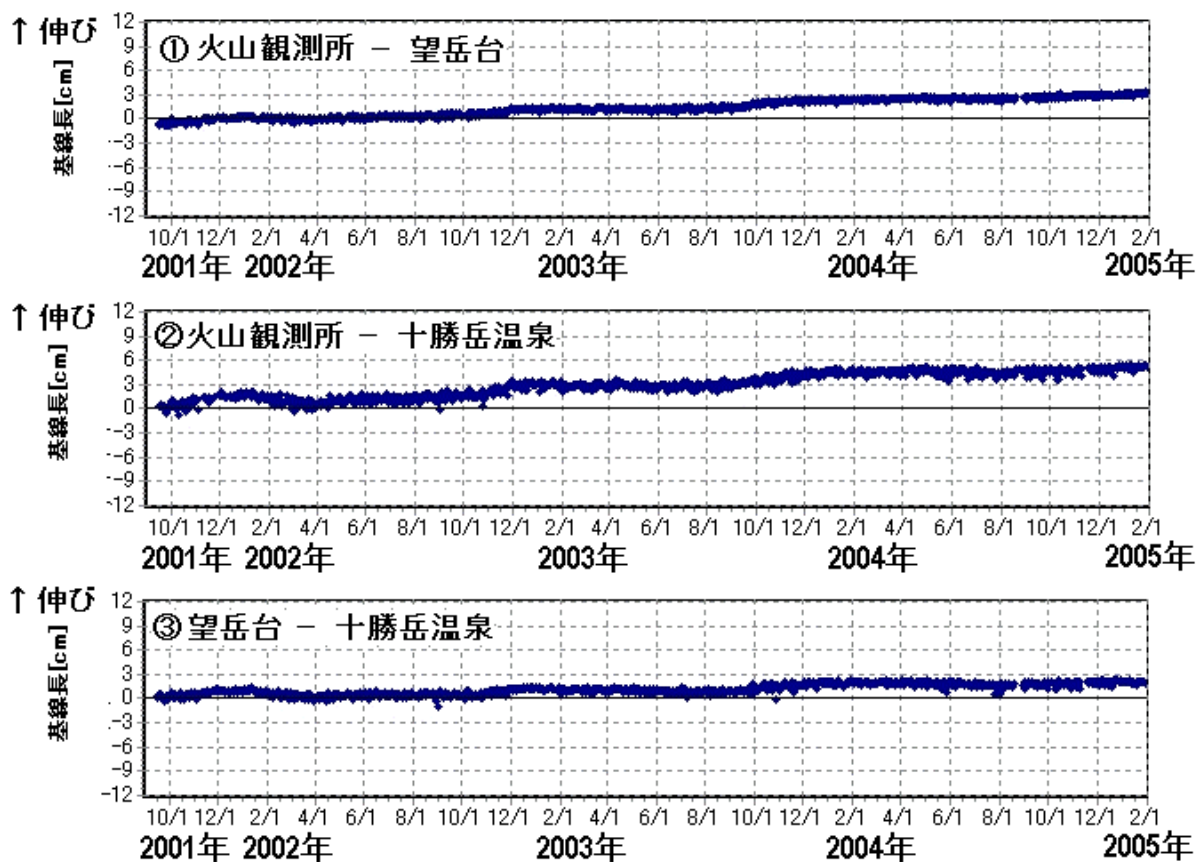
基線長変化（2001 年 9 月 13 日～2005 年 1 月 31 日）
