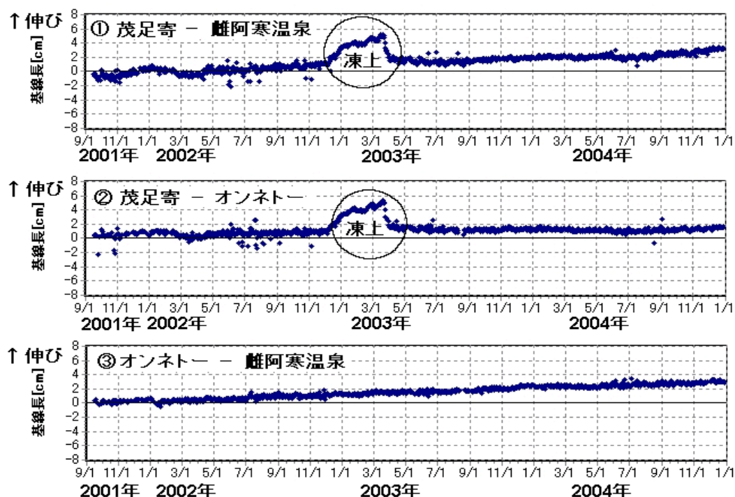
基線長変化（2001年9月19日～2004年12月31日）
