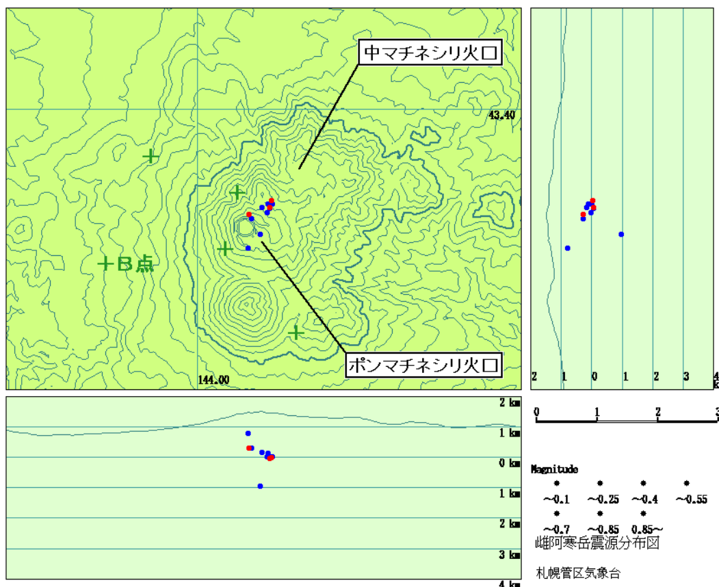
雌阿寒岳の震源分布図（丸印：震源、+印：地震観測点）
