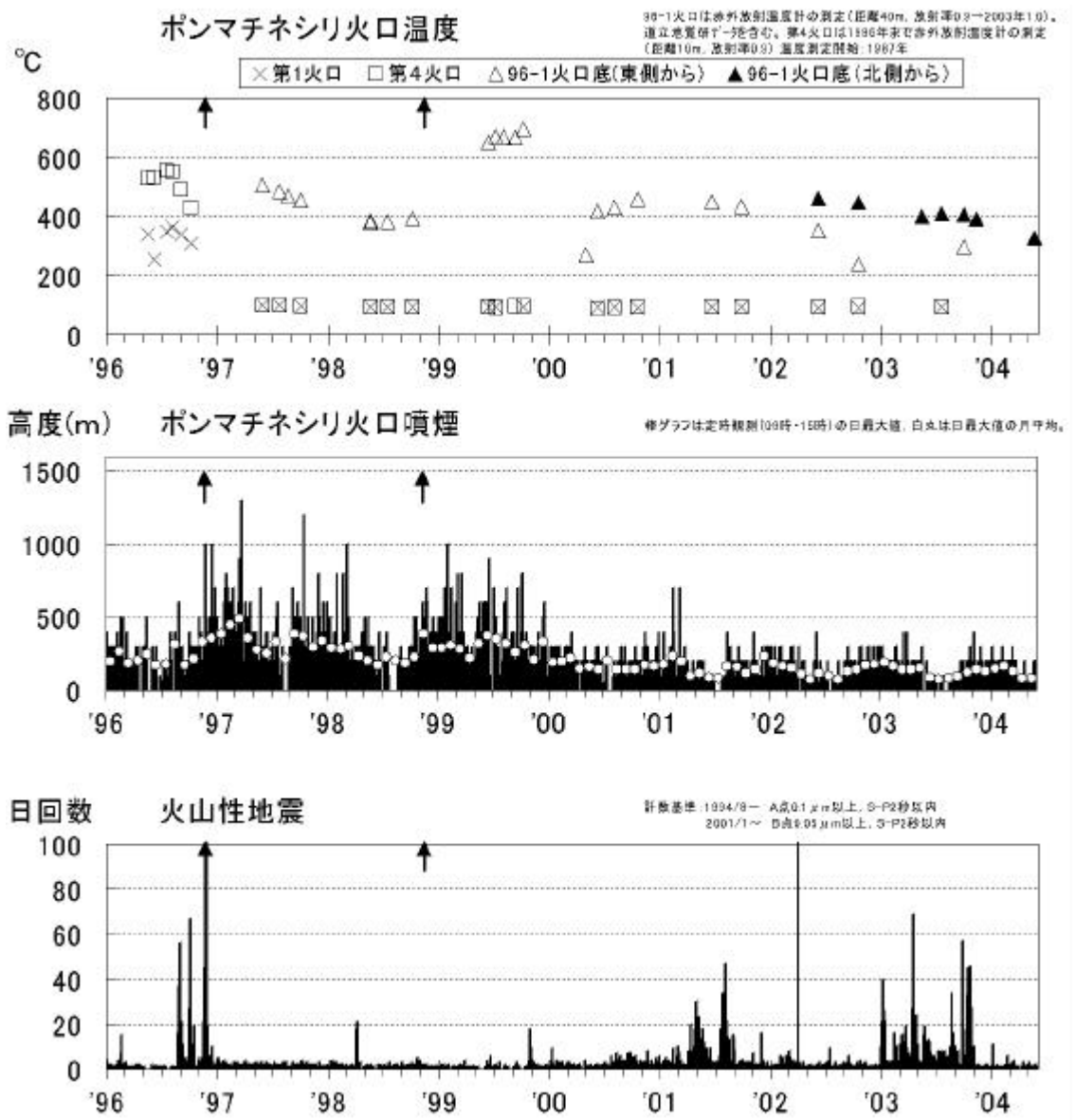
最近の火山活動経過図(1996年1月1日~2004年5月31日) 印は噴火
