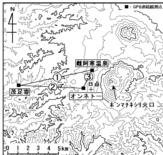
基線長変化(2001年9月19日~2004年5月31日)
