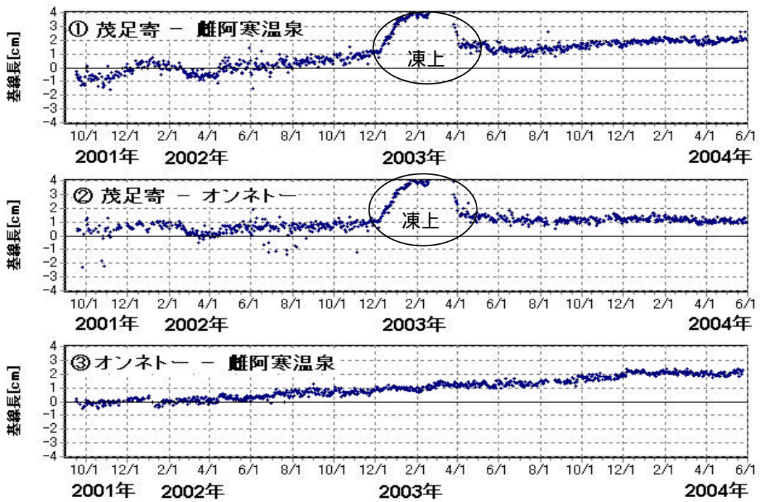
基線長変化(2001年9月19日~2004年5月31日)
