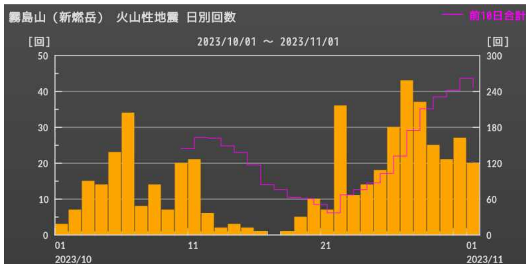
図6 霧島山（新燃岳） 火山性地震 日別回数 （2023年10月1日～11月1日（期間外））
