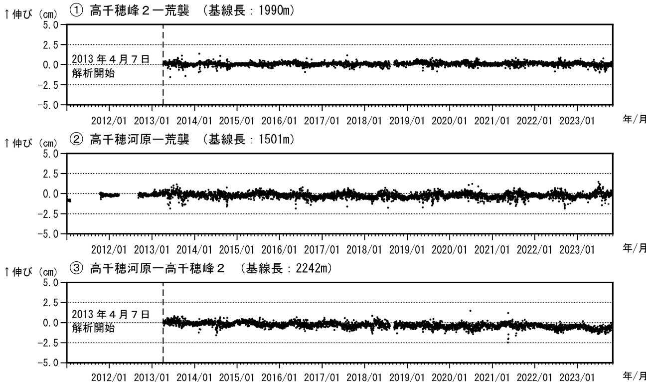
図6 霧島山（御鉢） GNSS 連続観測による基線長変化（2011年1月～2023年10月）
