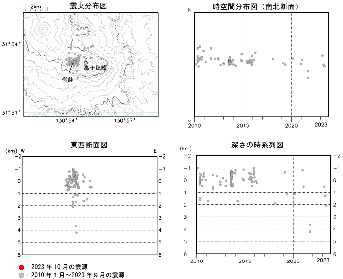
図4 霧島山（御鉢） 震源分布図（2010年1月～2023年10月）
