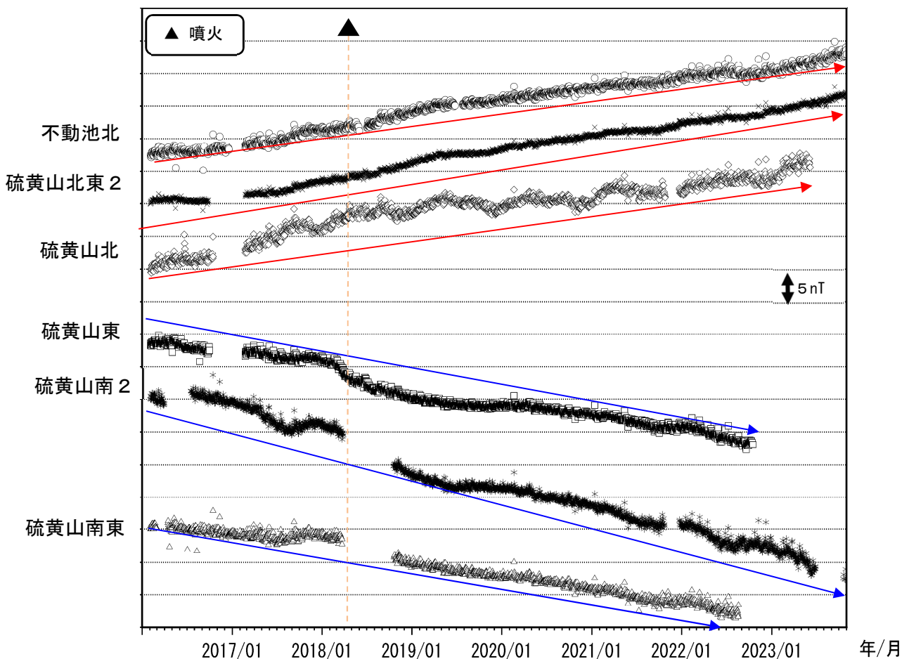
図 9-2 霧島山（えびの高原（硫黄山）周辺） 全磁力観測点で観測された全磁力変動（2016年1月～2023年10月）
