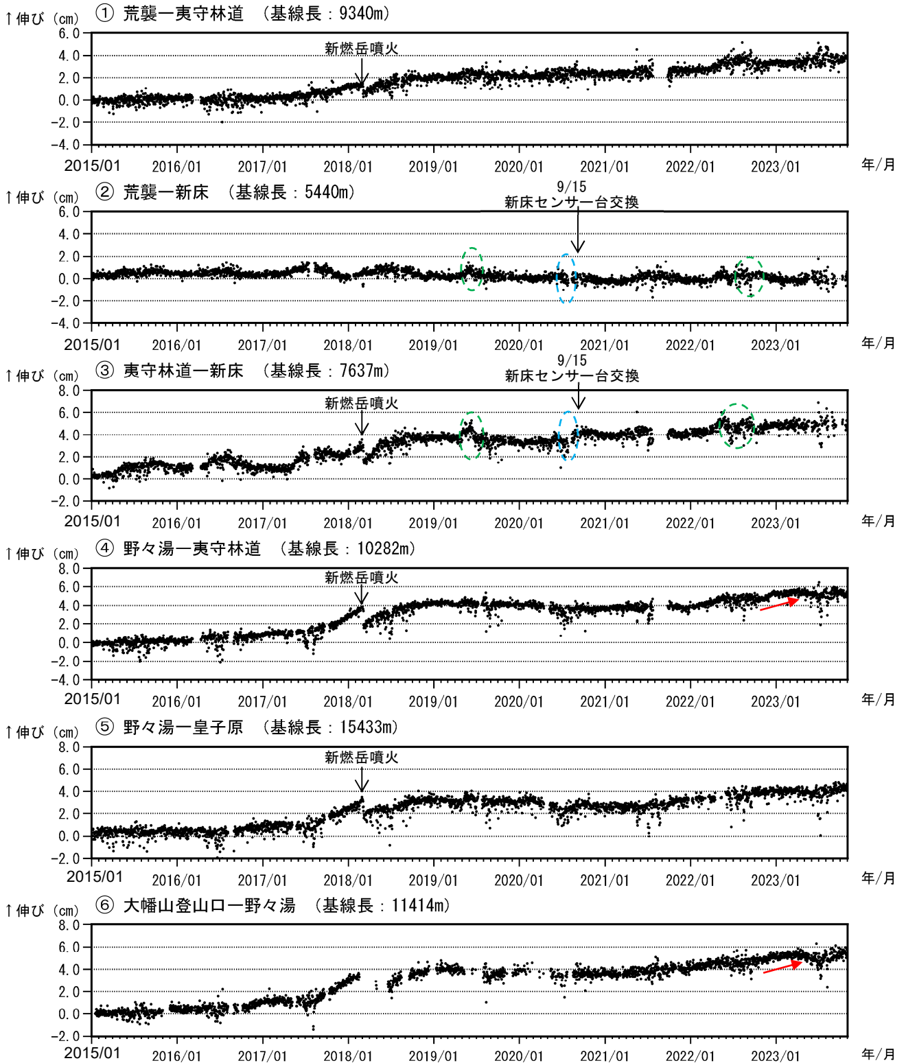
図9 霧島山（新燃岳） GNSS連続観測による基線長変化（2015年1月～2023年10月）
