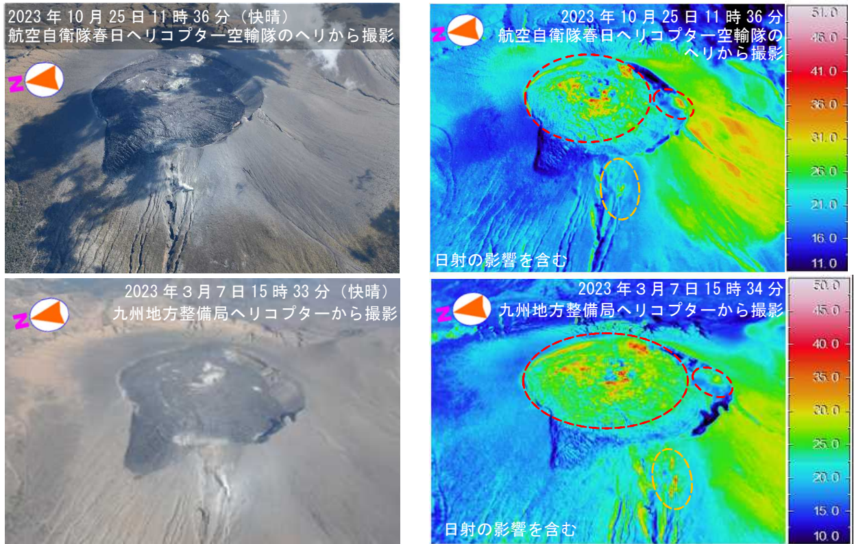
図3 霧島山（新燃岳） 新燃岳火口内及び西側割れ目の状況（上空から観測）
