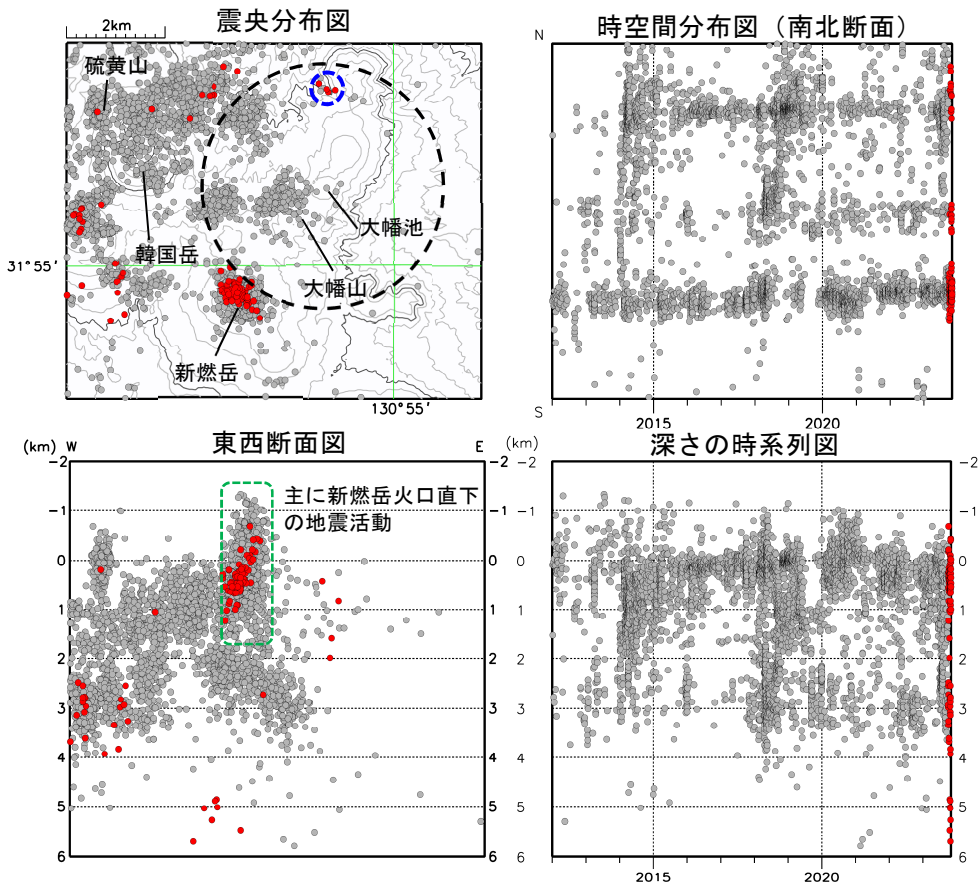
図5 霧島山（大幡池） 震源分布図（2012年1月～2023年10月）
