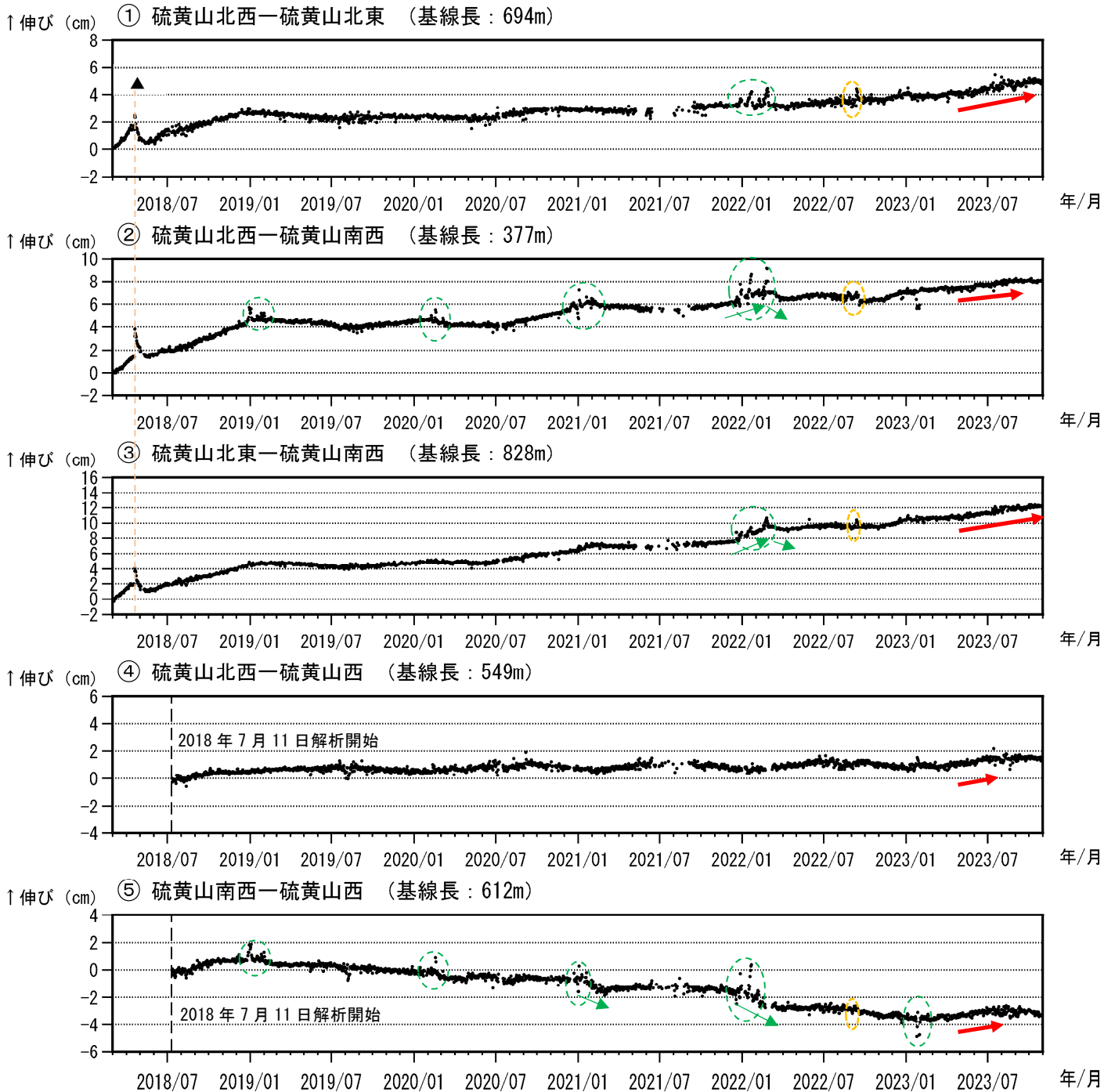
図8 霧島山（えびの高原（硫黄山）周辺） GNSS 連続観測による基線長変化 （2018年3月～2023年10月）
