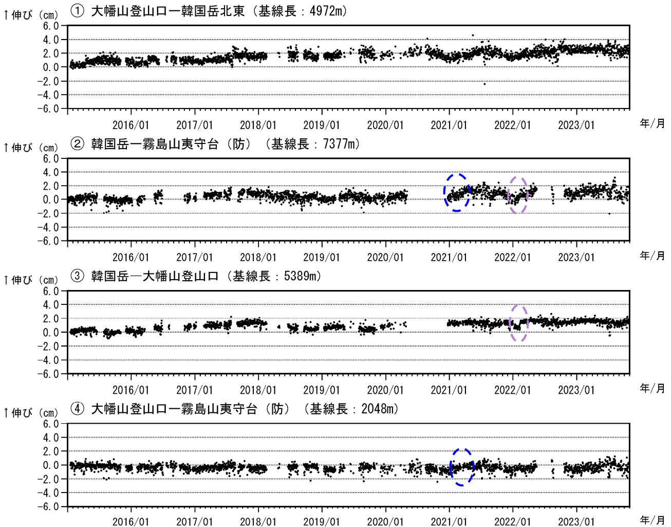
図6 霧島山(大幡池) GNSS連続観測による基線長変化(2015年1月~2023年10月)
