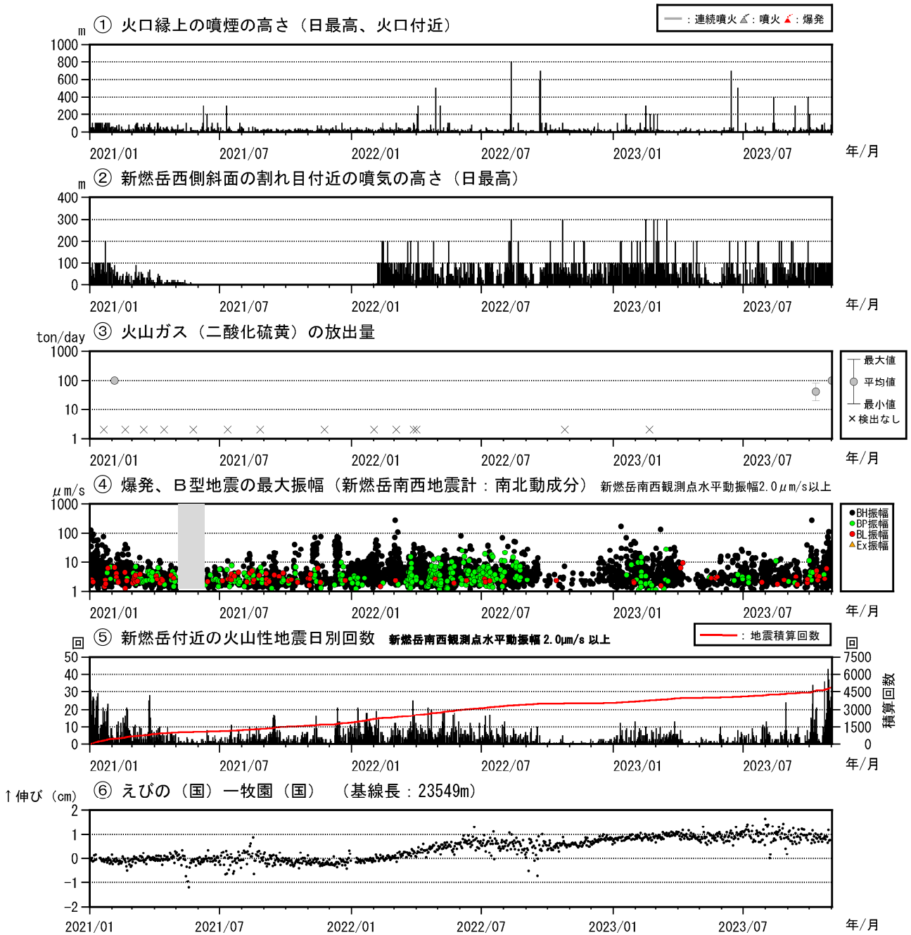
図7 霧島山（新燃岳） 火山活動経過図（2021年1月～2023年11月1日（期間外））
