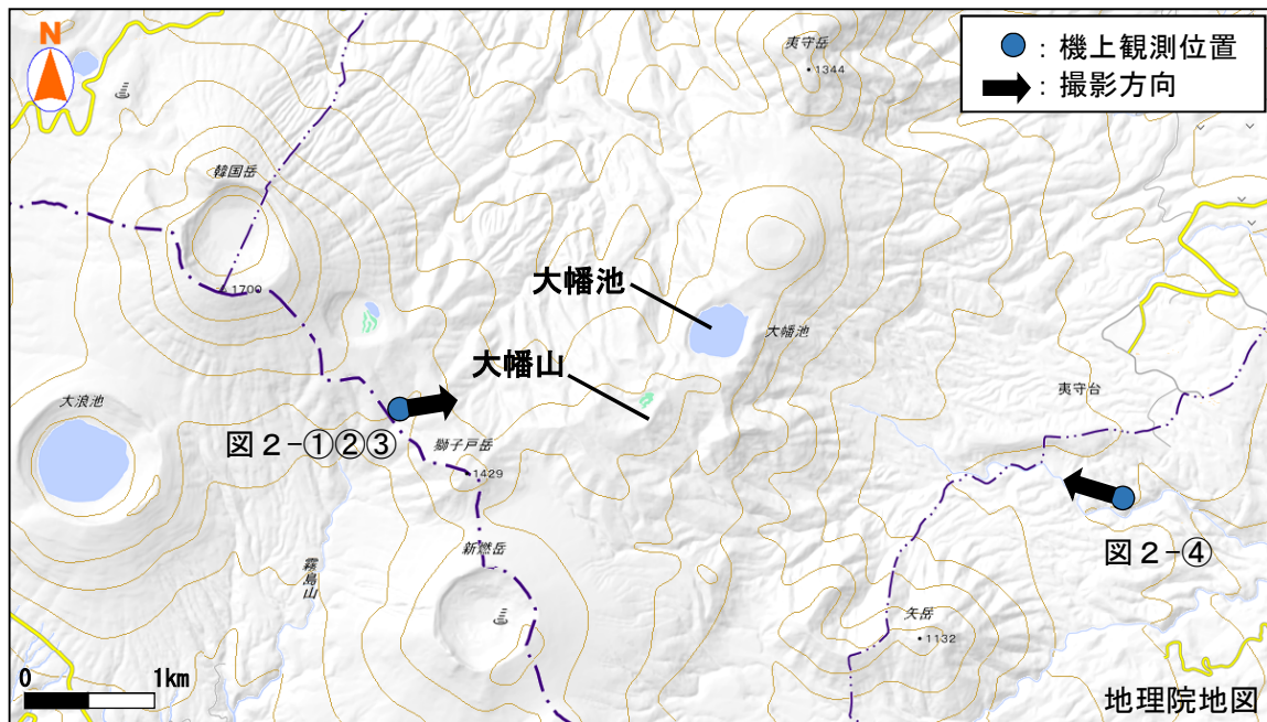
図3 霧島山（大幡池） 上空からの観測位置及び撮影方向
