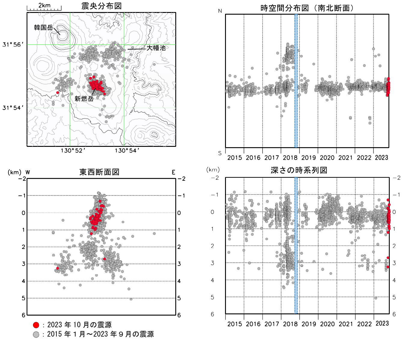
図8 霧島山（新燃岳） 震源分布図（2015年1月～2023年10月）
