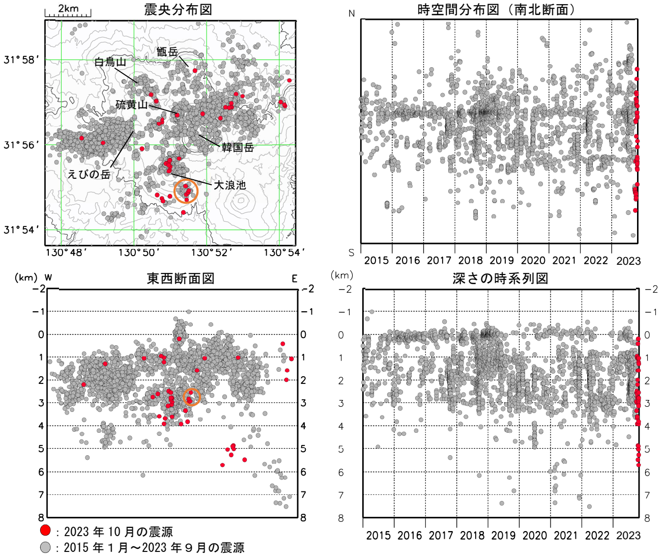
図 6 霧島山 (えびの高原 (硫黄山) 周辺) 震源分布図 (2015 年 1 月～2023 年 10 月)
