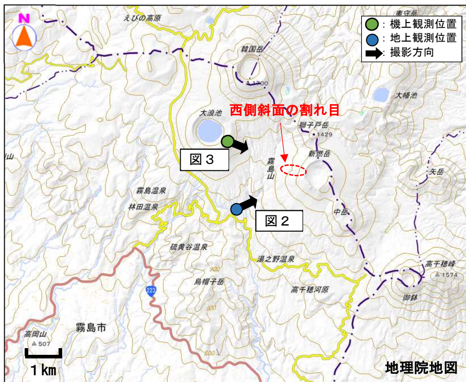
図4 霧島山（新燃岳） 図2・図3の観測位置及び撮影方向
