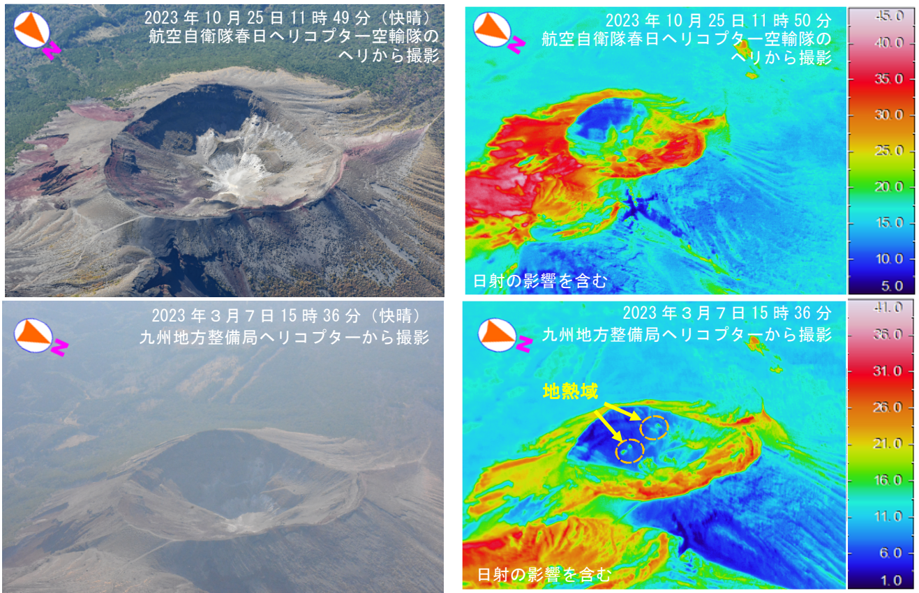
図2 霧島山（御鉢） 御鉢火口内及びその周辺の状況（上空から観測）
