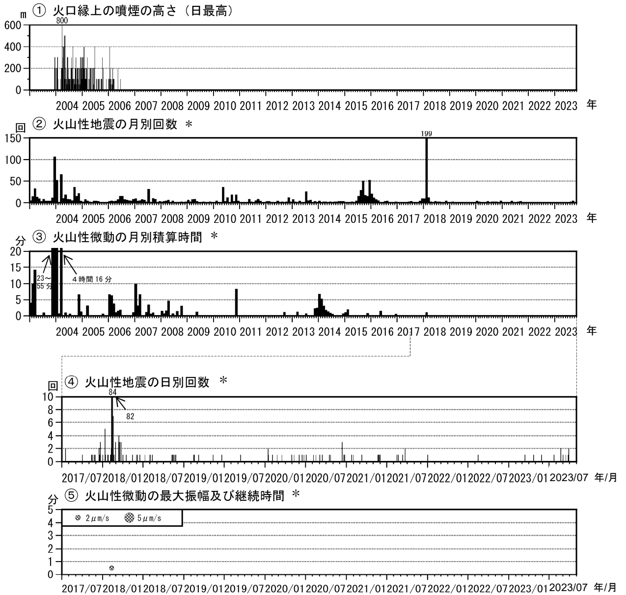
図5 霧島山（御鉢） 火山活動経過図（2003年1月～2023年10月）
