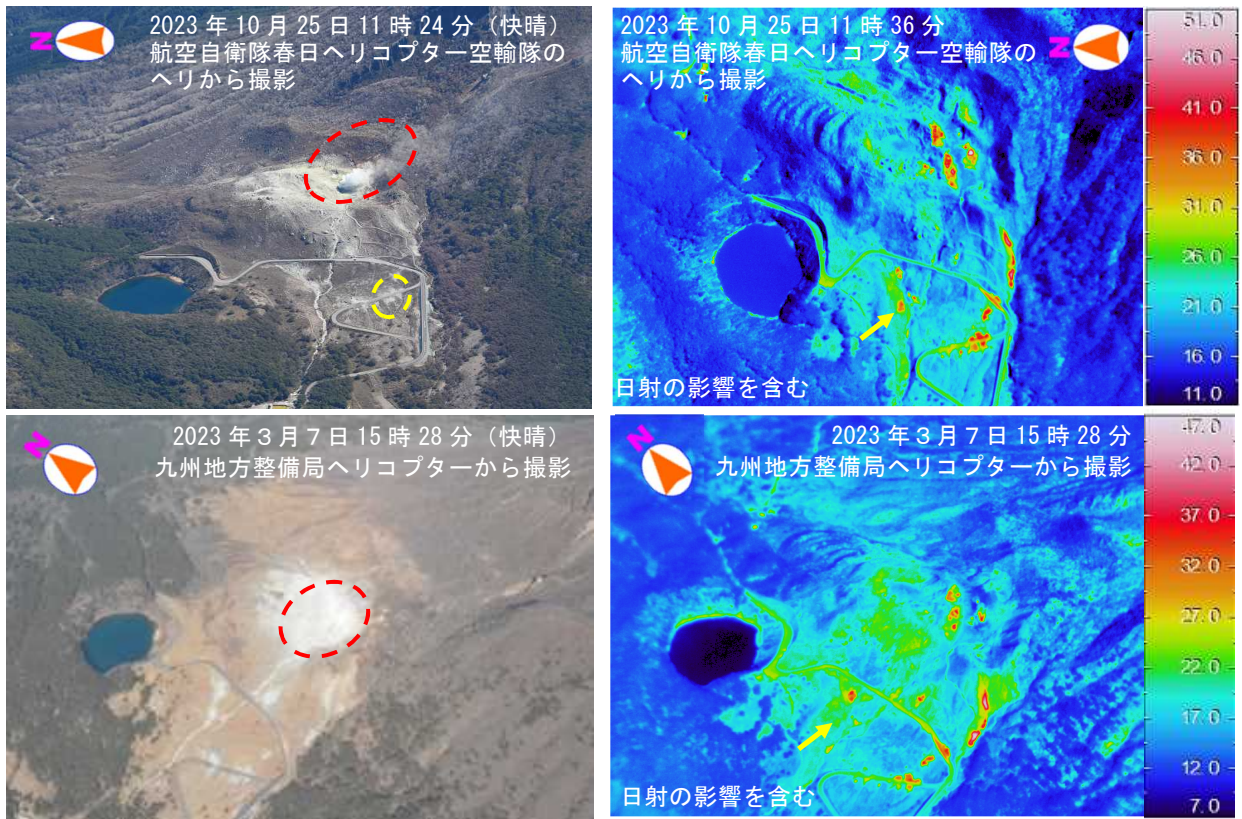
図3 霧島山（えびの高原（硫黄山）周辺） 硫黄山及びその周辺の状況（上空から観測）
