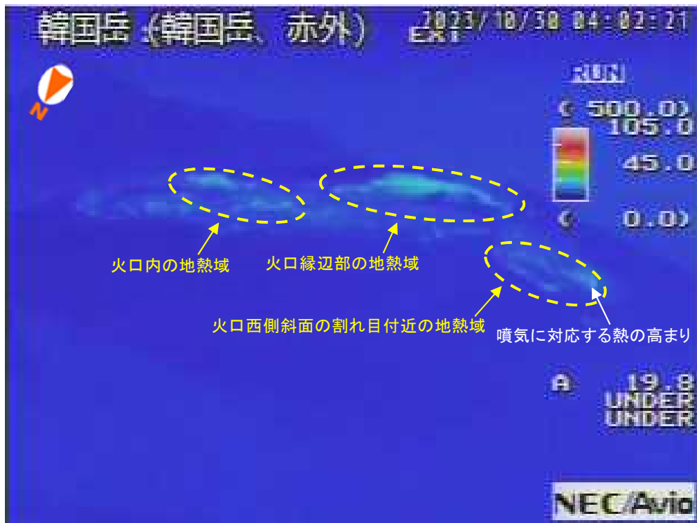
図1-2 霧島山（新燃岳）地熱域の状況（10月30日、韓国岳監視カメラ）
