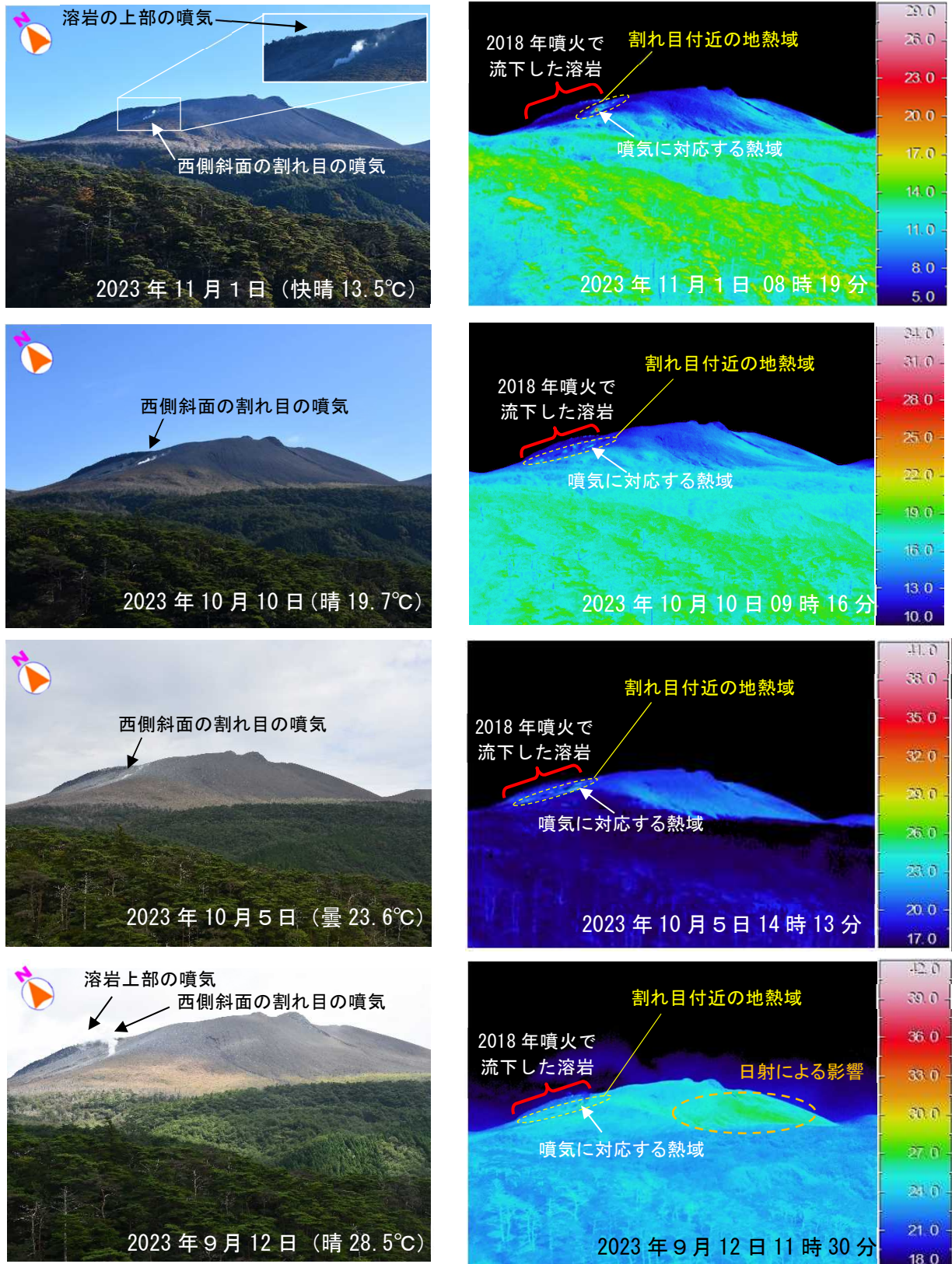
図2 霧島山（新燃岳） 新燃岳南西側の状況（新湯温泉付近（図4）から観測）
