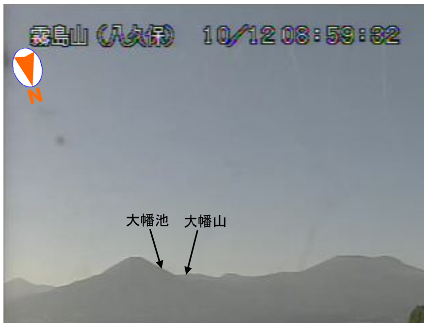
図1 霧島山（大幡池） 大幡池及び大幡山の状況（10月12日、八久保監視カメラ） 監視カメラによる観測では、噴煙は認められませんでした。
