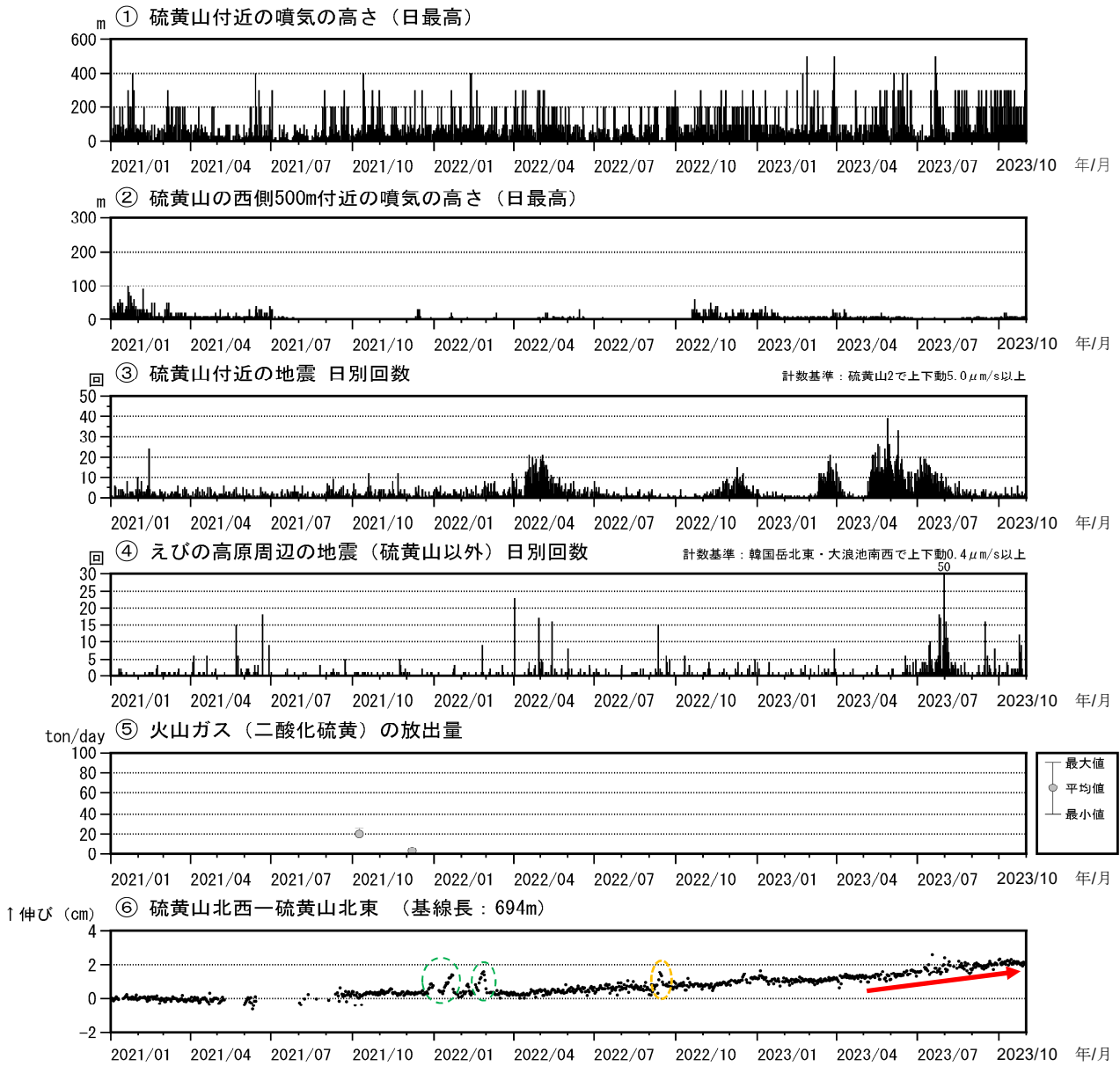
図5 霧島山（えびの高原（硫黄山）周辺）火山活動経過図（2021年1月～2023年10月）
