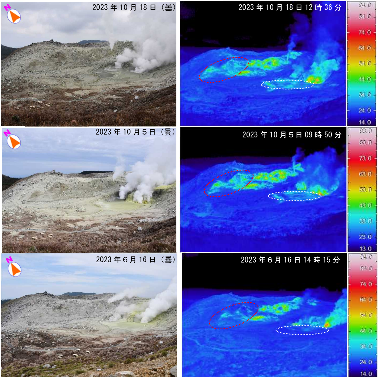
図2 霧島山（えびの高原（硫黄山）周辺） 硫黄山の南側の噴気及び地熱域の状況
