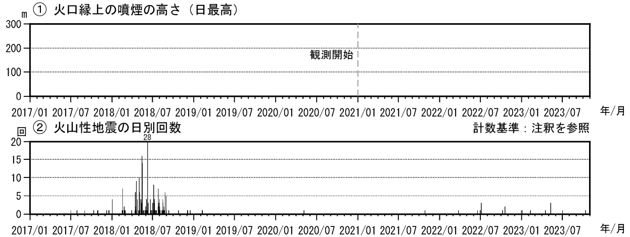
図4 霧島山（大幡池） 火山活動経過図（2017年1月～2023年10月）
