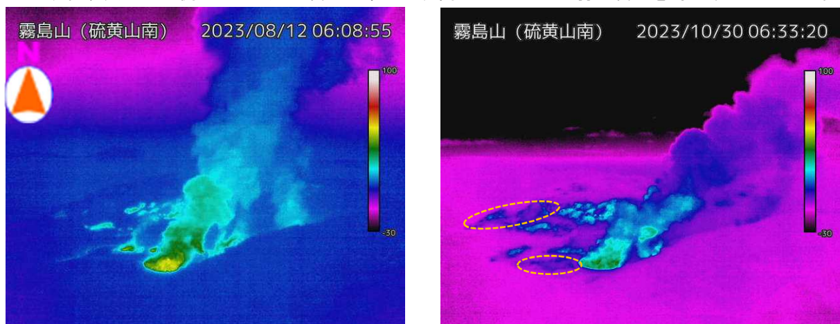
図1-2 霧島山（えびの高原（硫黄山）周辺） 硫黄山南側の状況 （10月30日、硫黄山南監視カメラ）
