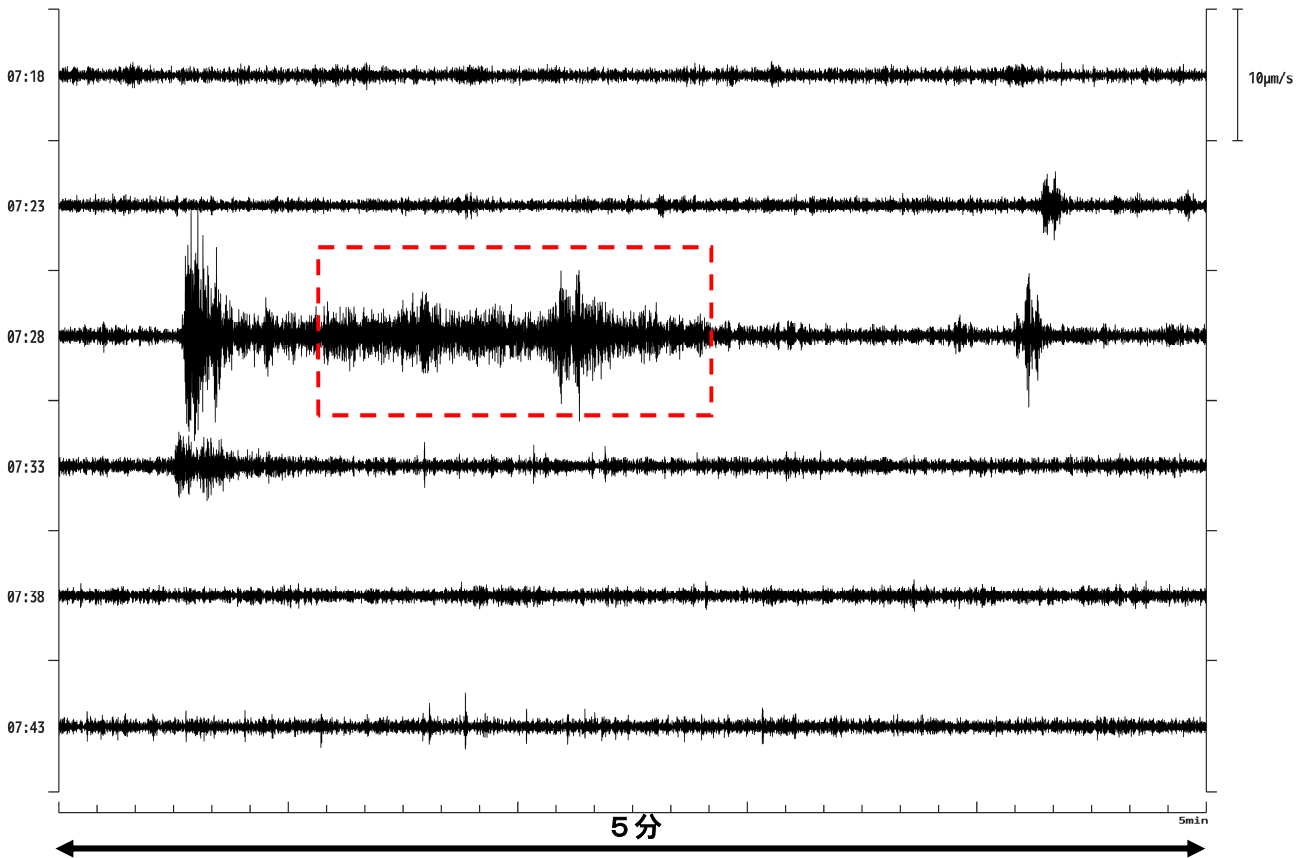
図5 霧島山（新燃岳） 10月7日07時28分に発生した火山性微動の状況 （2023年10月7日07時18分～47分、新燃岳南西地震計：南北動成分）
