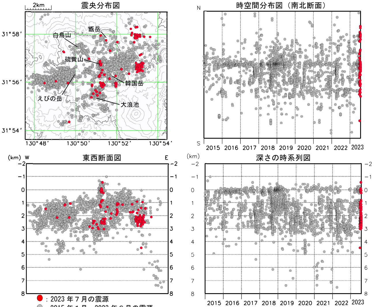
図6 霧島山（えびの高原（硫黄山）周辺） 震源分布図（2015年1月～2023年7月）
