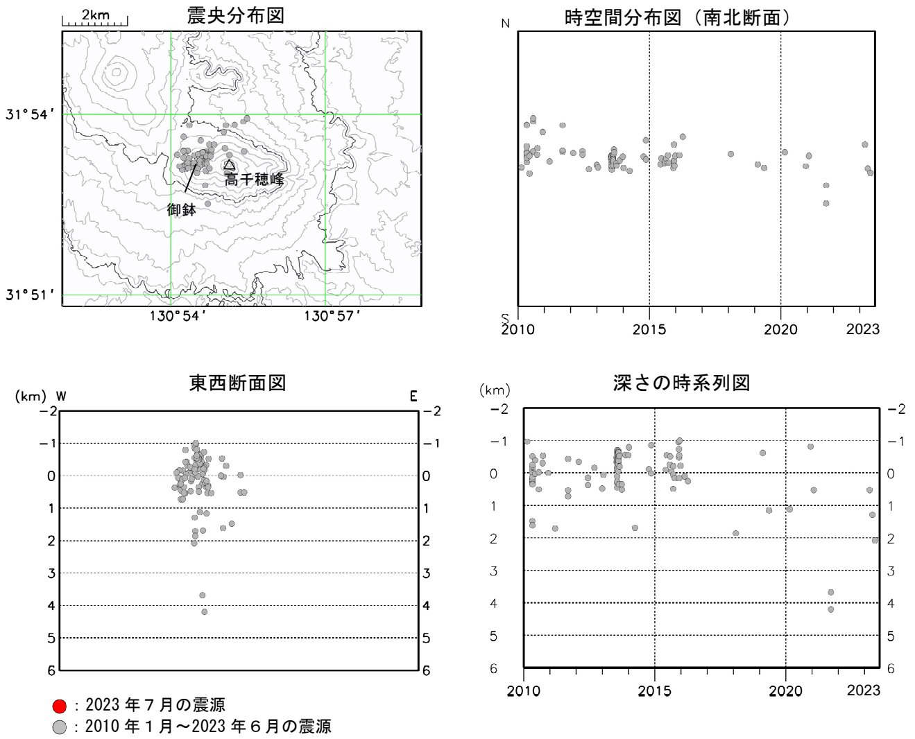
図2 霧島山（御鉢） 震源分布図（2010年1月～2023年7月）
