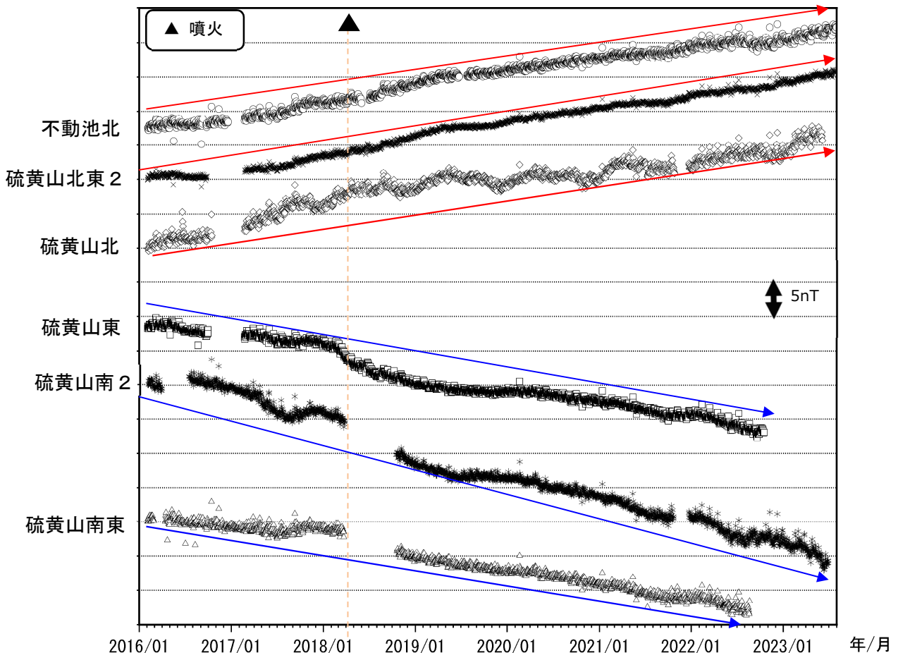
図 9-2 霧島山（えびの高原（硫黄山）周辺） 全磁力観測点で観測された全磁力変動 （2016年1月～2023年7月）
