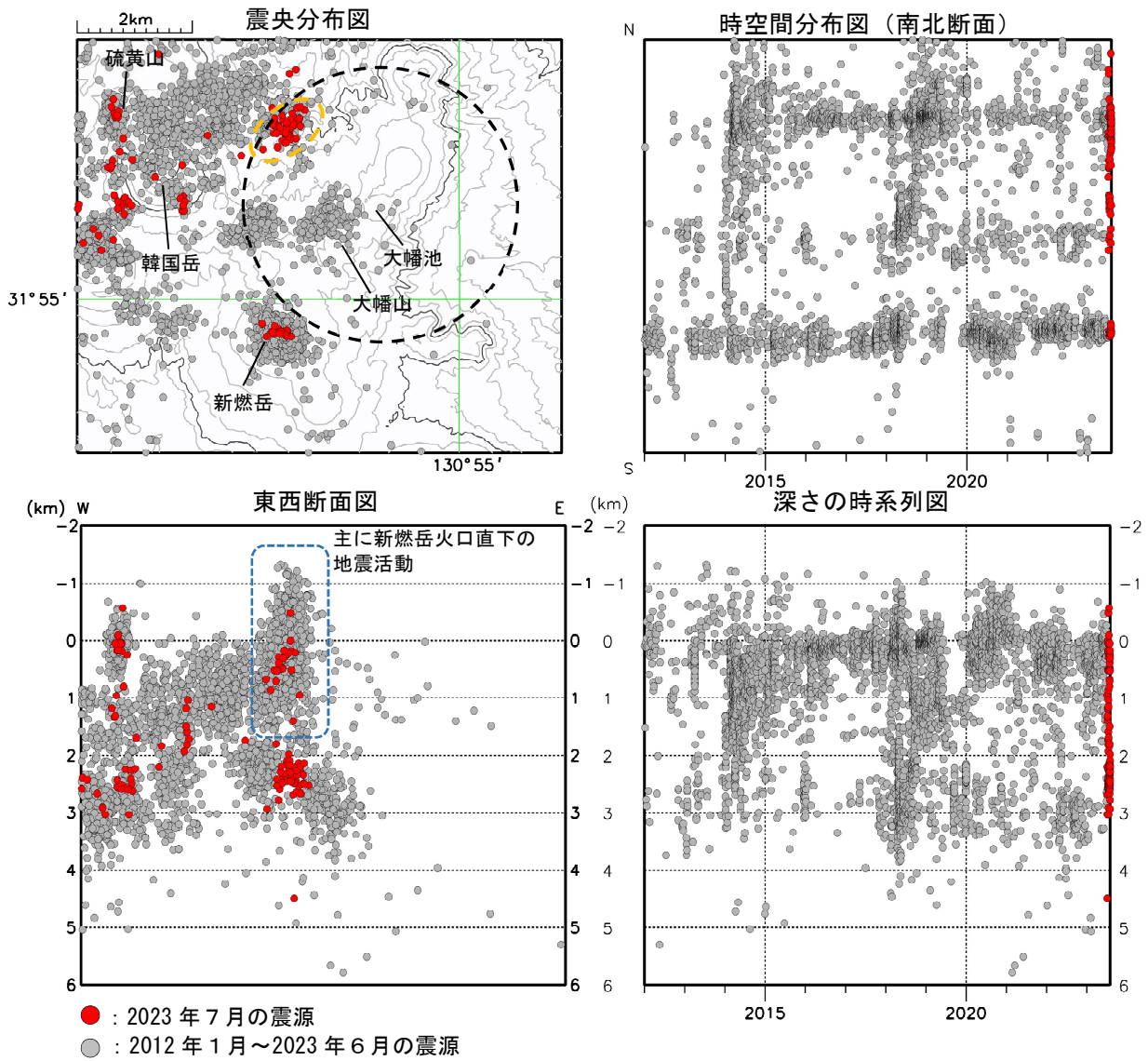
図3 霧島山（大幡池） 震源分布図（2012年1月～2023年7月）
