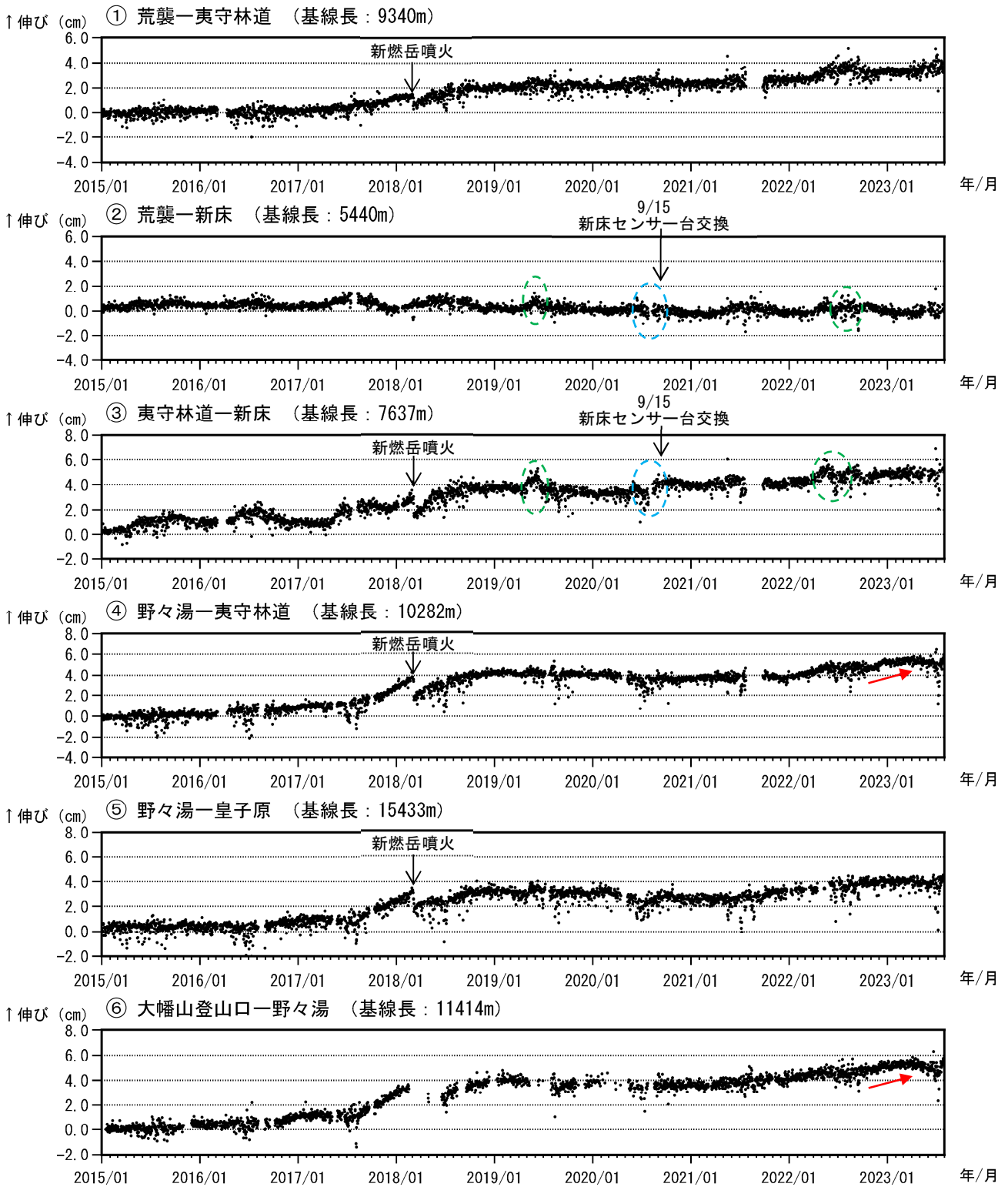
図4 霧島山（新燃岳） GNSS連続観測による基線長変化（2015年1月～2023年7月）
