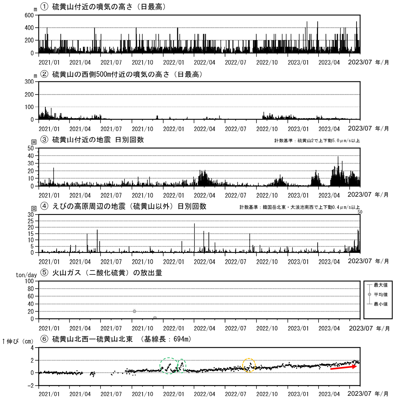
図5 霧島山（えびの高原（硫黄山）周辺） 火山活動経過図（2021年1月～2023年7月）
