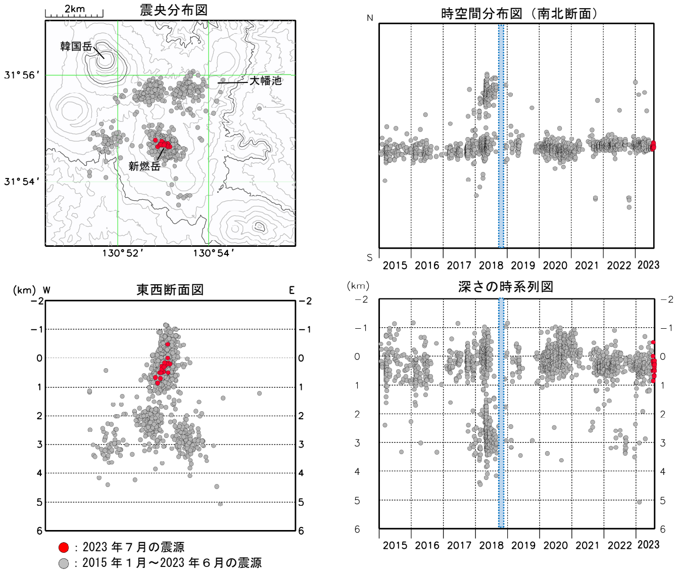
図3 霧島山（新燃岳） 震源分布図（2015年1月～2023年7月）
