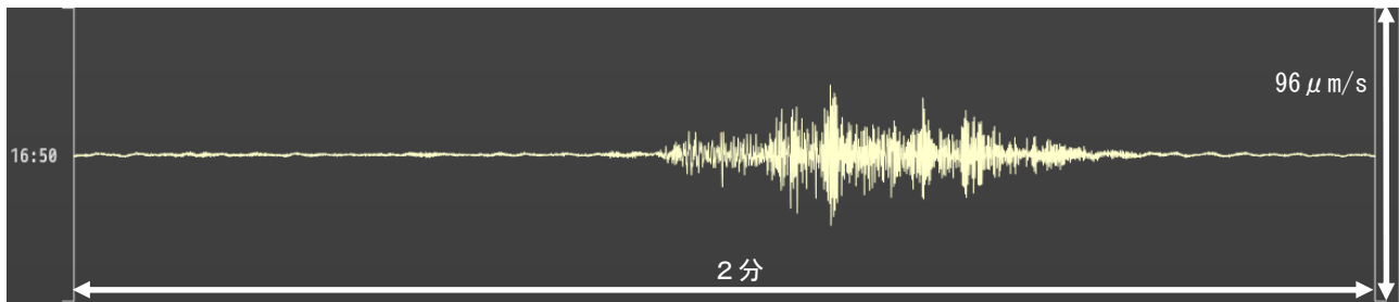
図1 霧島山（えびの高原（硫黄山）周辺）7月7日16時50分に発生した火山性微動 （硫黄山北東観測点上下動成分、16時50分～51分）
