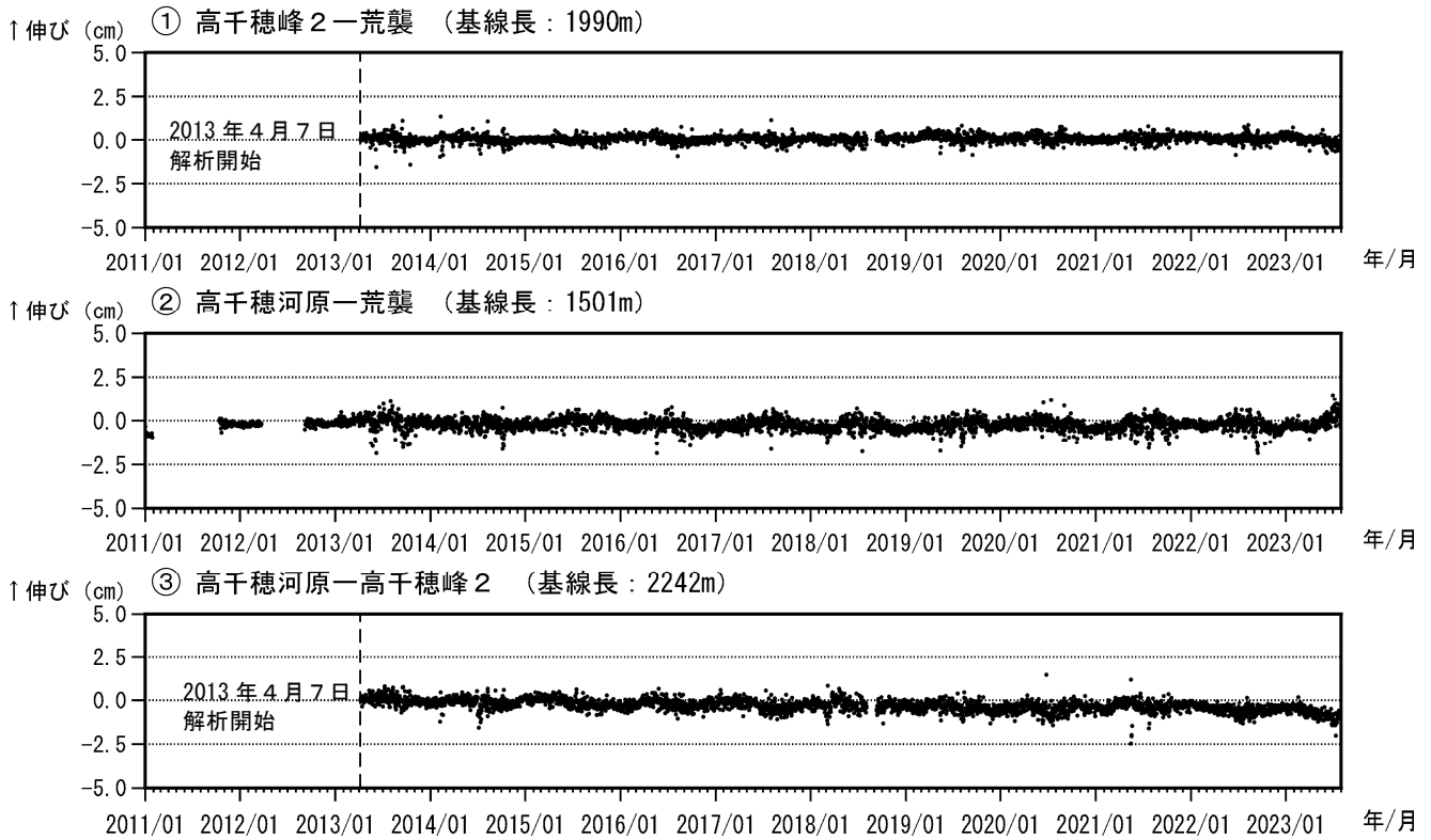
図4 霧島山（御鉢） GNSS連続観測による基線長変化（2011年1月～2023年7月）
