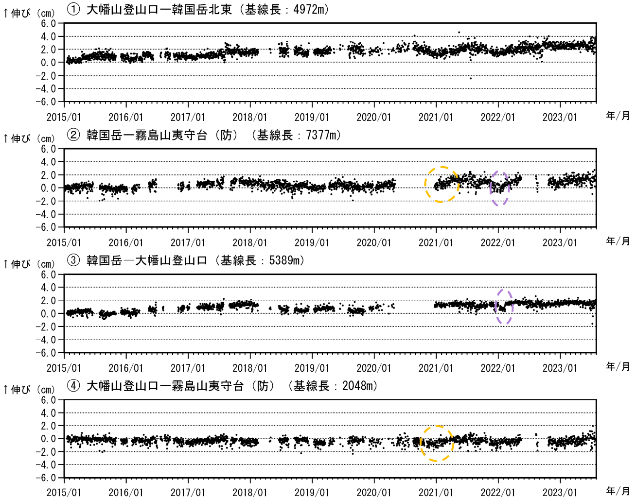
図4 霧島山（大幡池） GNSS 連続観測による基線長変化（2015年1月～2023年7月）
