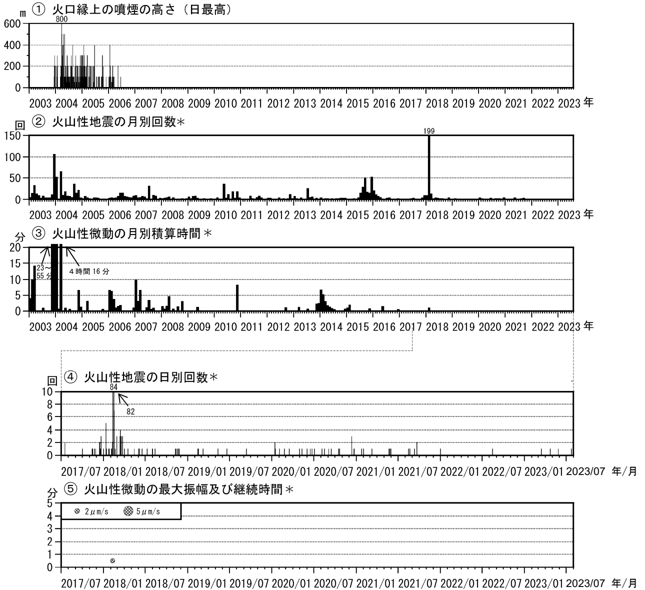
図3 霧島山（御鉢） 火山活動経過図（2003年1月～2023年7月）
