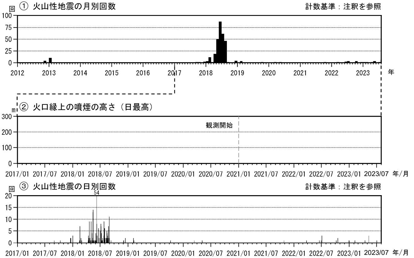
図2 霧島山（大幡池） 火山活動経過図（2012年1月～2023年7月）
