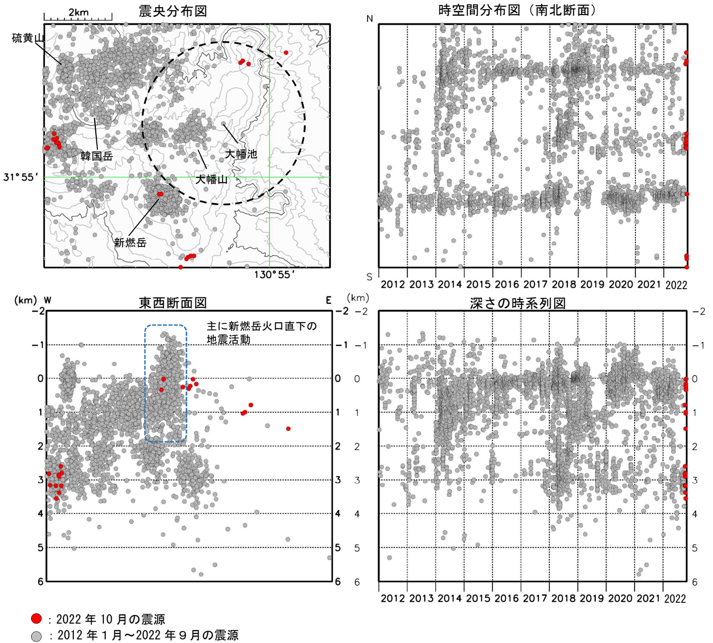
図6 霧島山（大幡池） 震源分布図（2012年1月～2022年10月）
