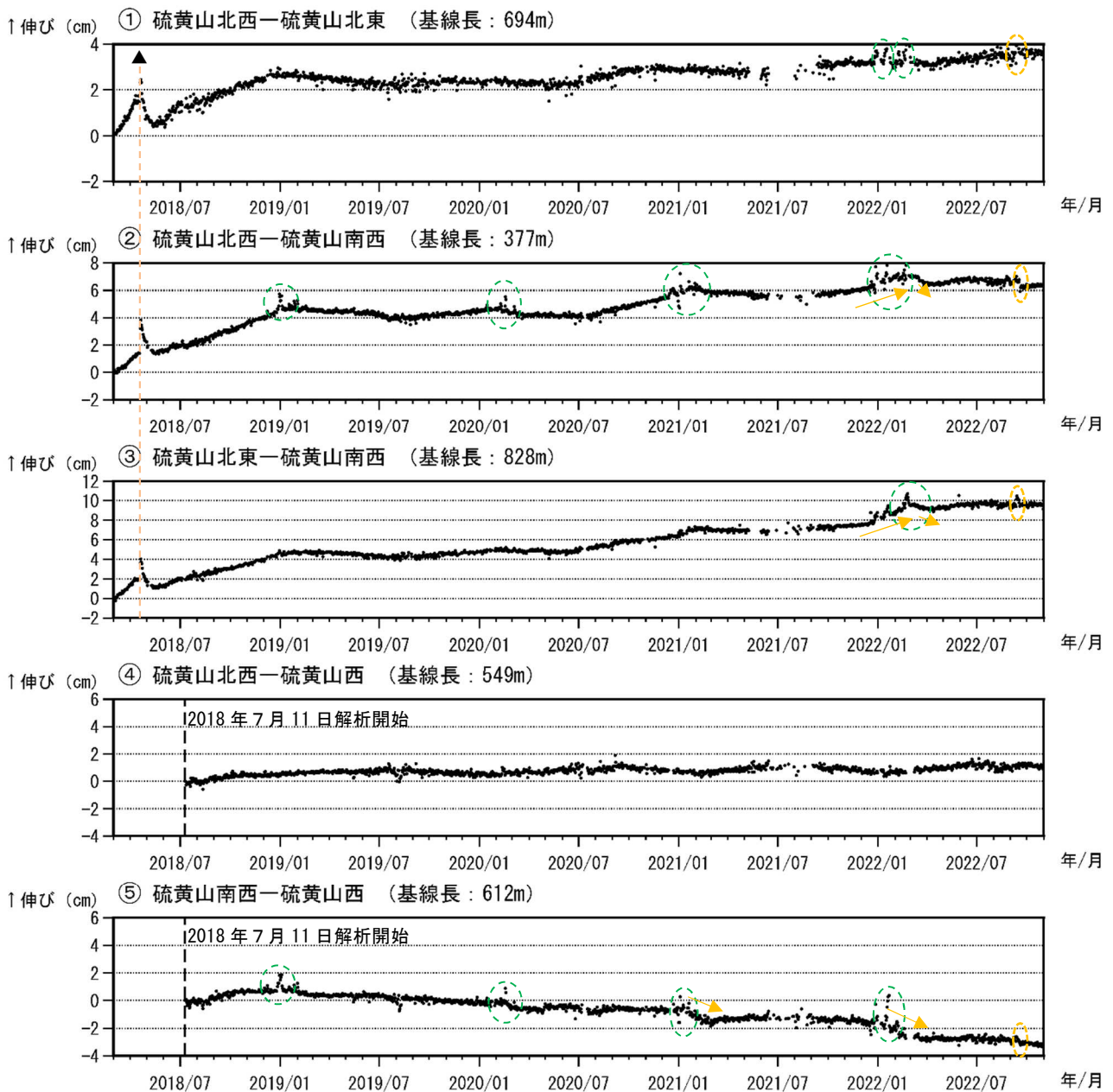
図8 霧島山（えびの高原（硫黄山）周辺） GNSS 連続観測による基線長変化 （2018年3月～2022年10月）
