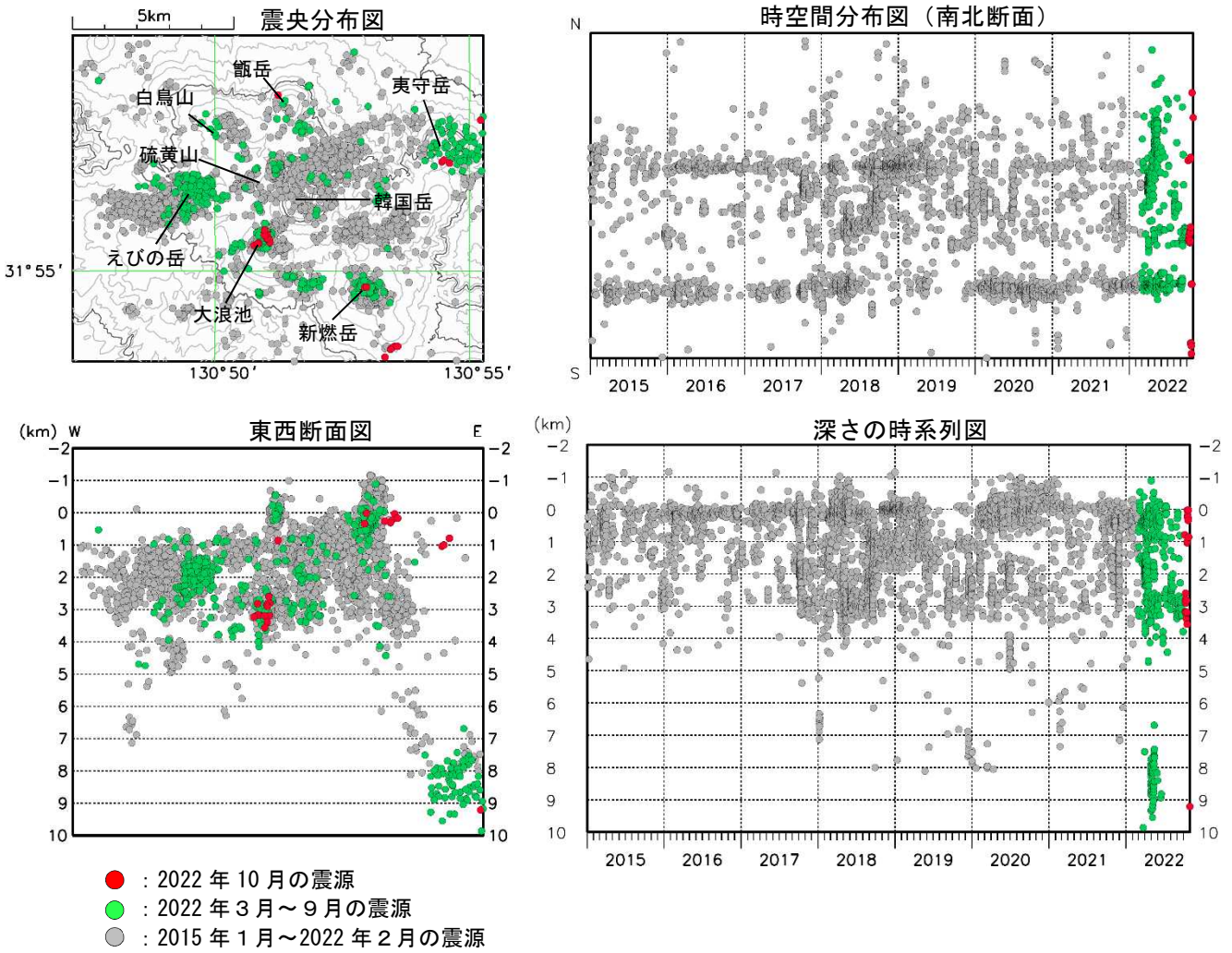
図 6-2 霧島山（新燃岳及びえびの高原（硫黄山）周辺） 震源分布図 （2015年1月～2022年10月）
