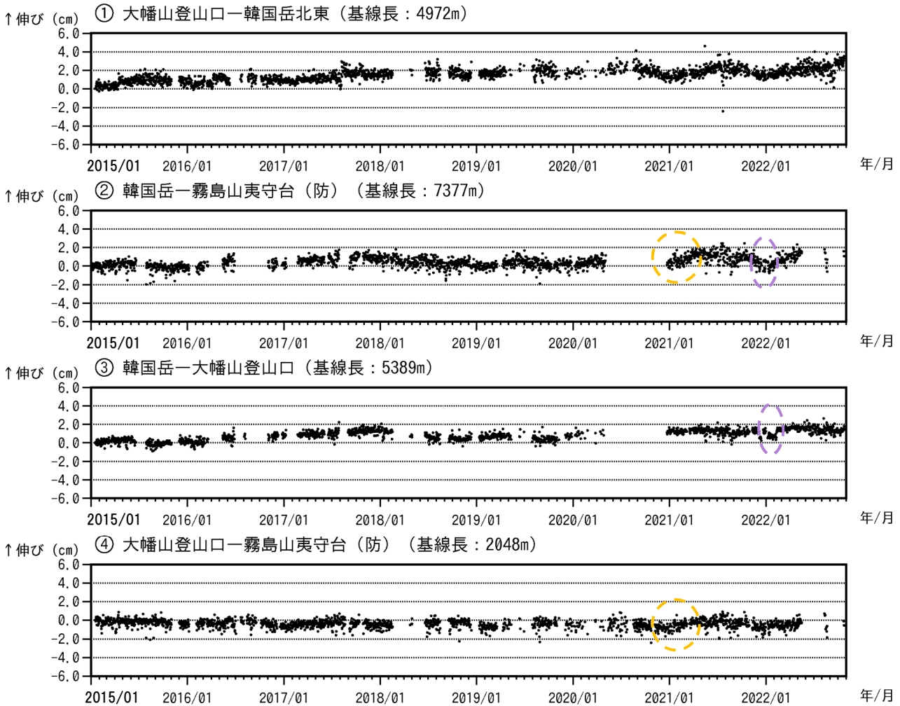
図7 霧島山 (大幡池) GNSS 連続観測による基線長変化 (2015年1月～2022年10月)
