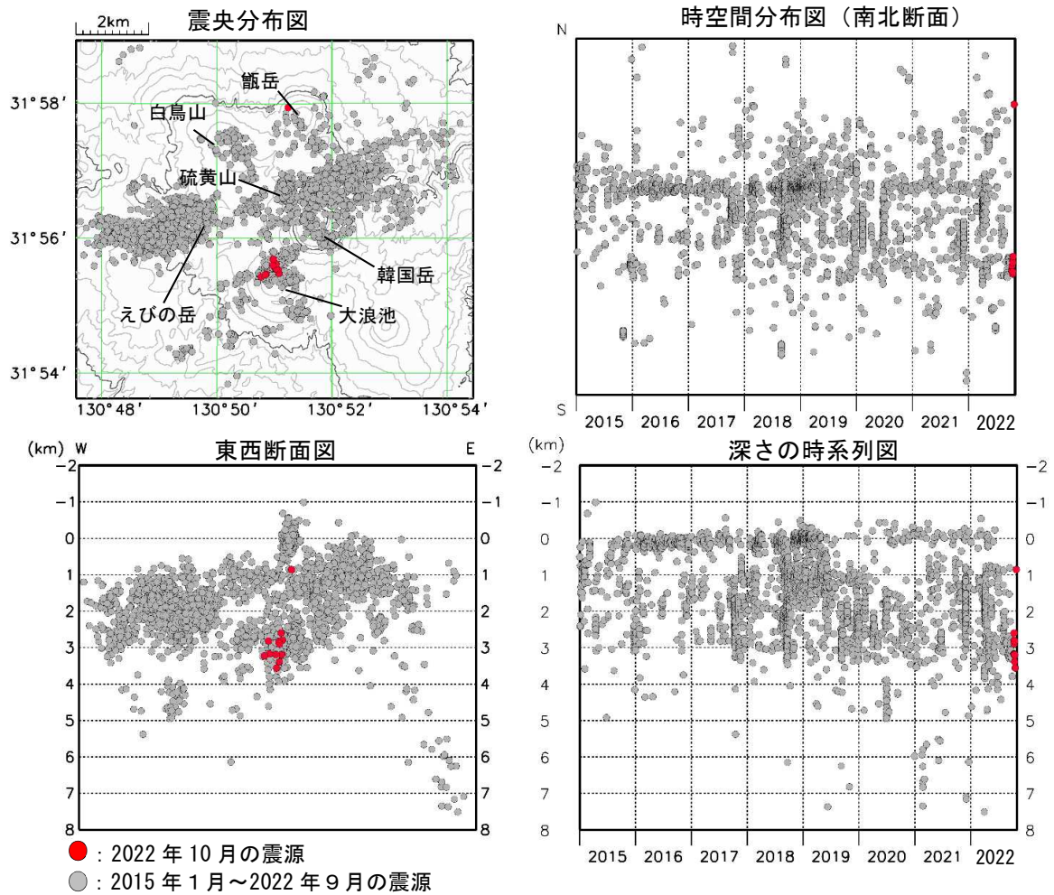
図6 霧島山（えびの高原（硫黄山）周辺） 震源分布図（2015年1月～2022年10月）
