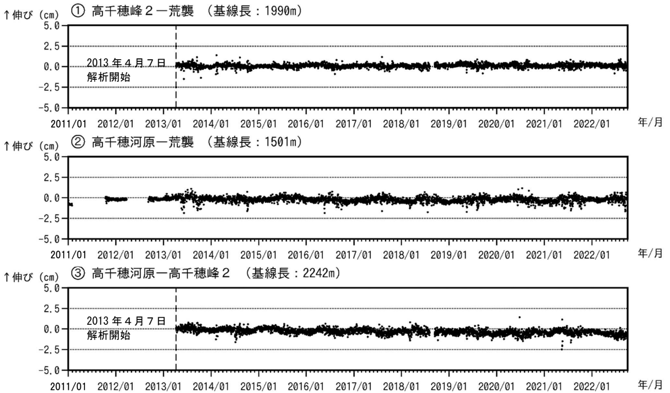
図6 霧島山（御鉢） GNSS 連続観測による基線長変化（2011年1月～2022年10月）
