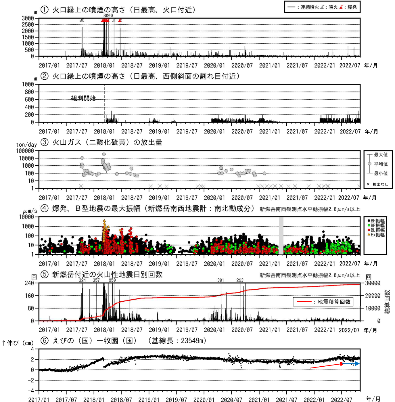
図5 霧島山（新燃岳） 火山活動経過図（2017年1月～2022年10月）
