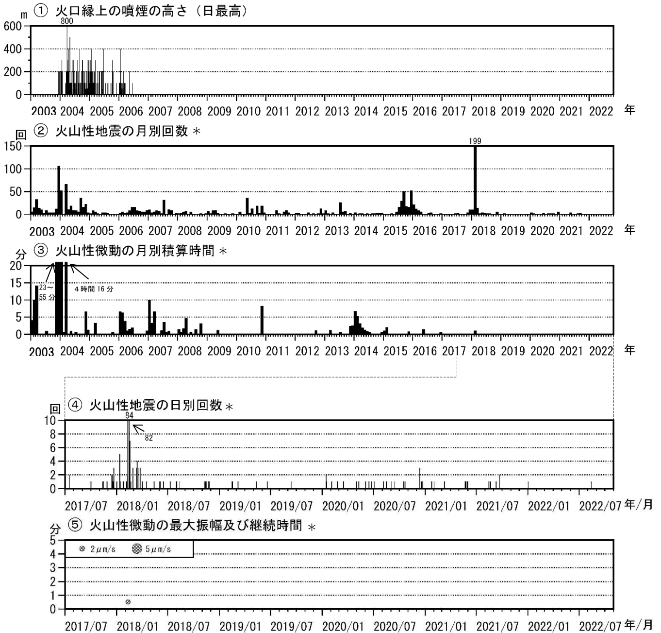
図4 霧島山（御鉢） 火山活動経過図（2003年1月～2022年10月）
