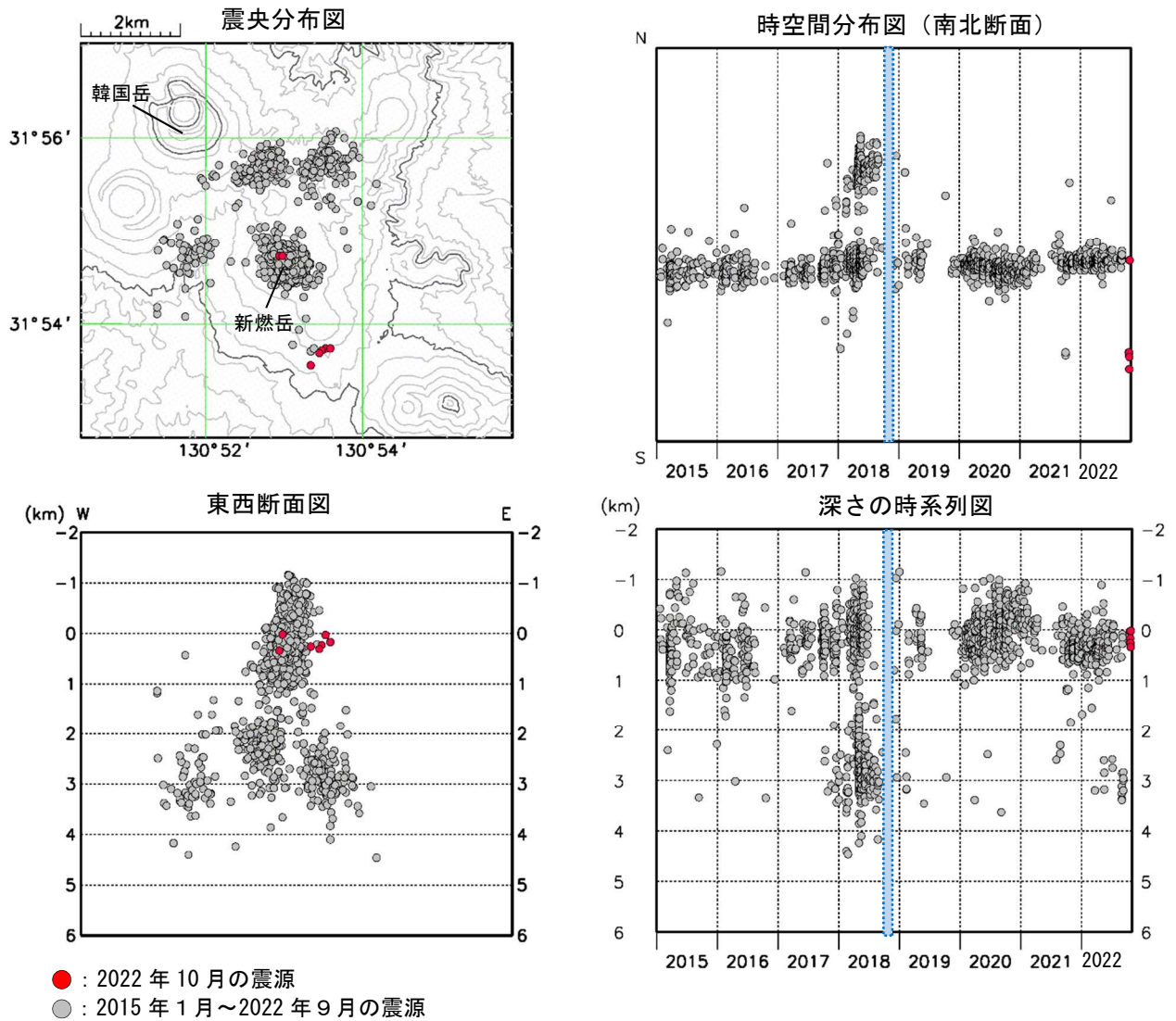
図 6-1 霧島山（新燃岳） 震源分布図（2015年1月～2022年10月）
