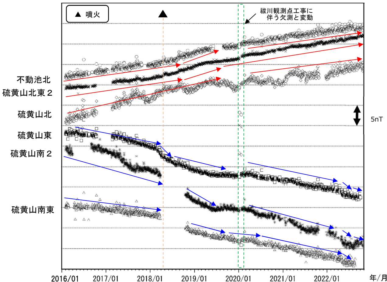
図 9-2 霧島山（えびの高原（硫黄山）周辺） 全磁力観測点で観測された全磁力変動（2016年1月～2022年10月）
