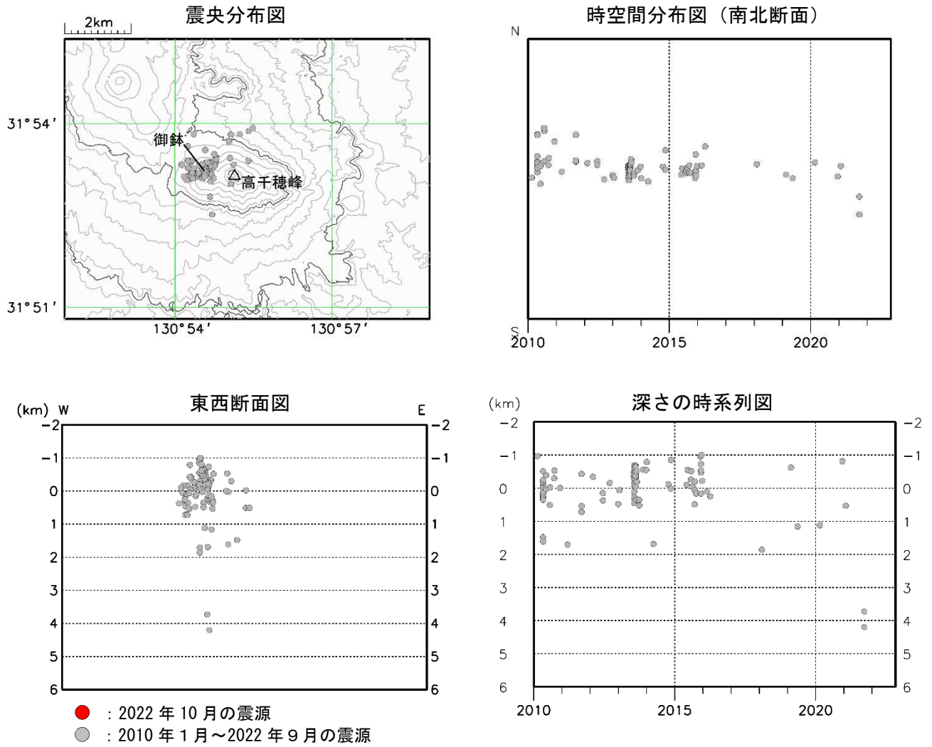
図5 霧島山（御鉢） 震源分布図（2010年1月～2022年10月）
