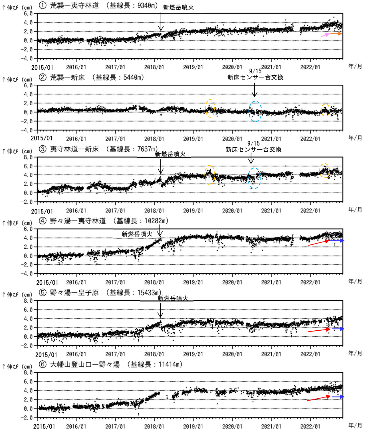
図7 霧島山（新燃岳） GNSS連続観測による基線長変化（2015年1月～2022年10月）
