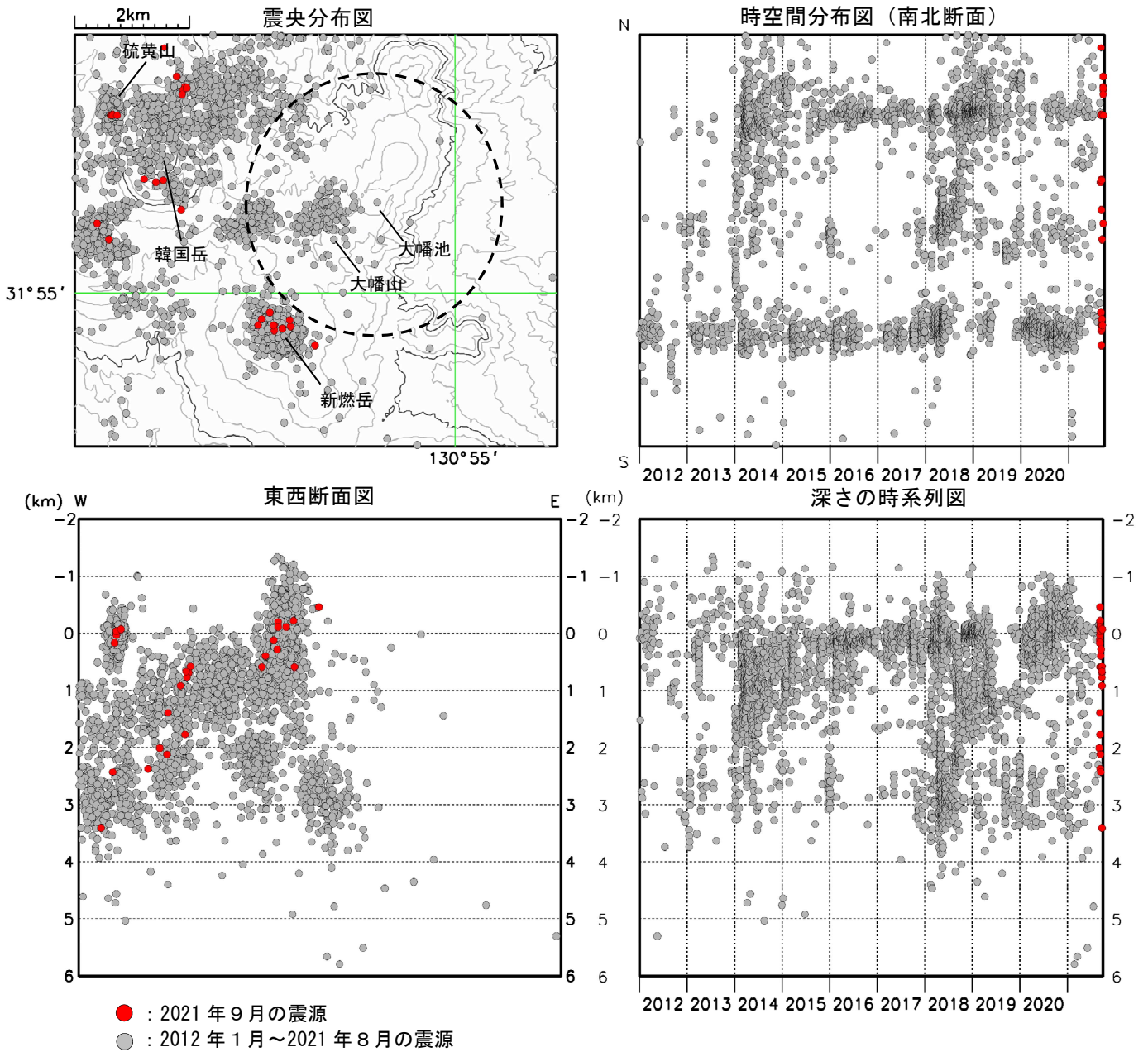
図3 霧島山（大幡池） 震源分布図（2012年1月～2021年9月）
