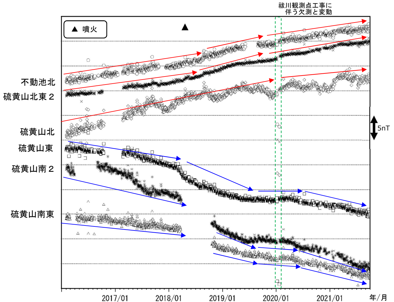
図 6-2 霧島山（えびの高原（硫黄山）周辺） 全磁力観測点で観測された全磁力変動（2016 年 1 月～2021 年 9 月）
