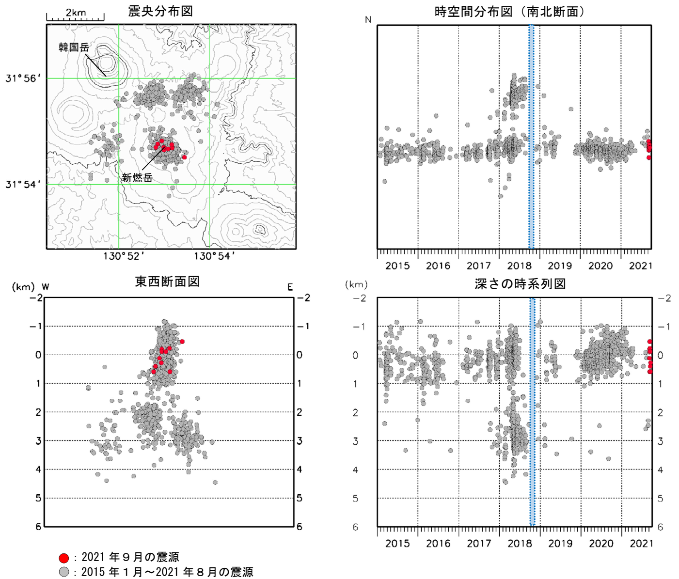
図3 霧島山（新燃岳）震源分布図（2015年1月～2021年9月）
