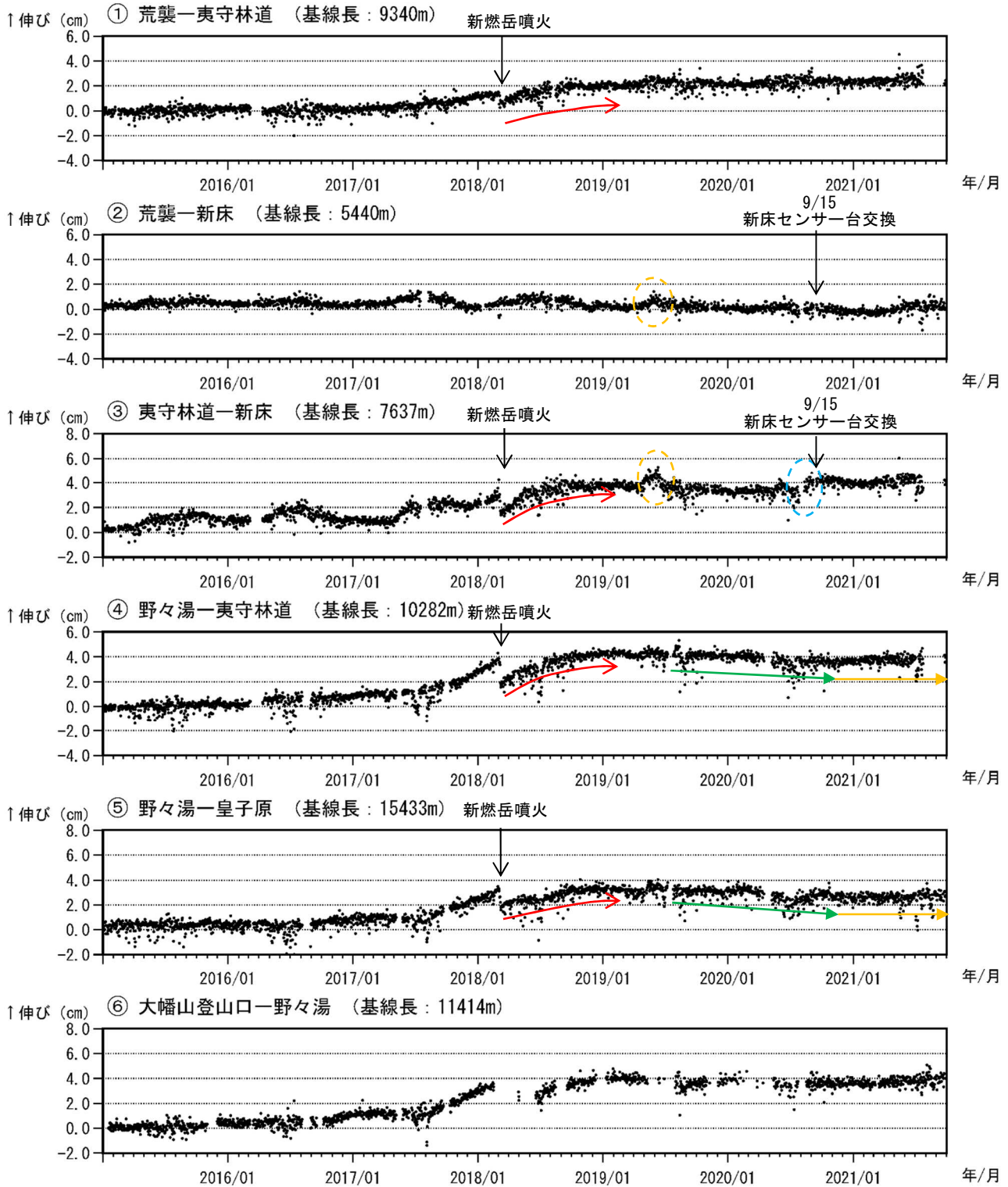
図4 霧島山（新燃岳） GNSS連続観測による基線長変化（2015年1月～2021年9月）
