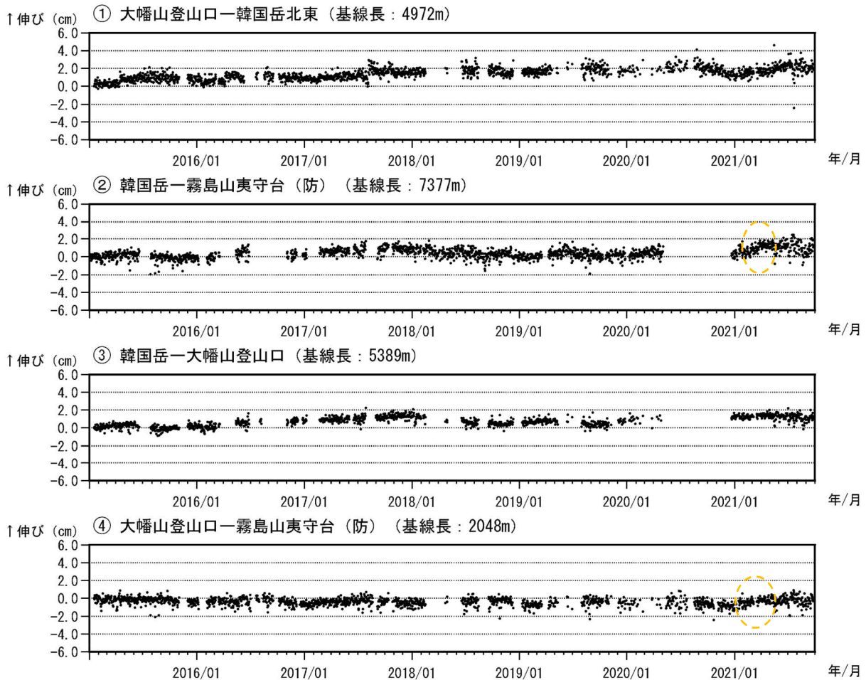
図4 霧島山（大幡池） GNSS 連続観測による基線長変化（2015年1月～2021年9月）
