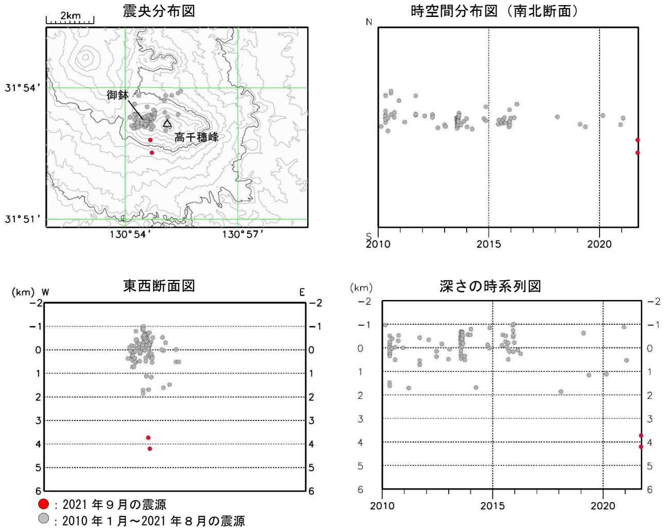
図3 霧島山（御鉢） 震源分布図（2010年1月～2021年9月）
