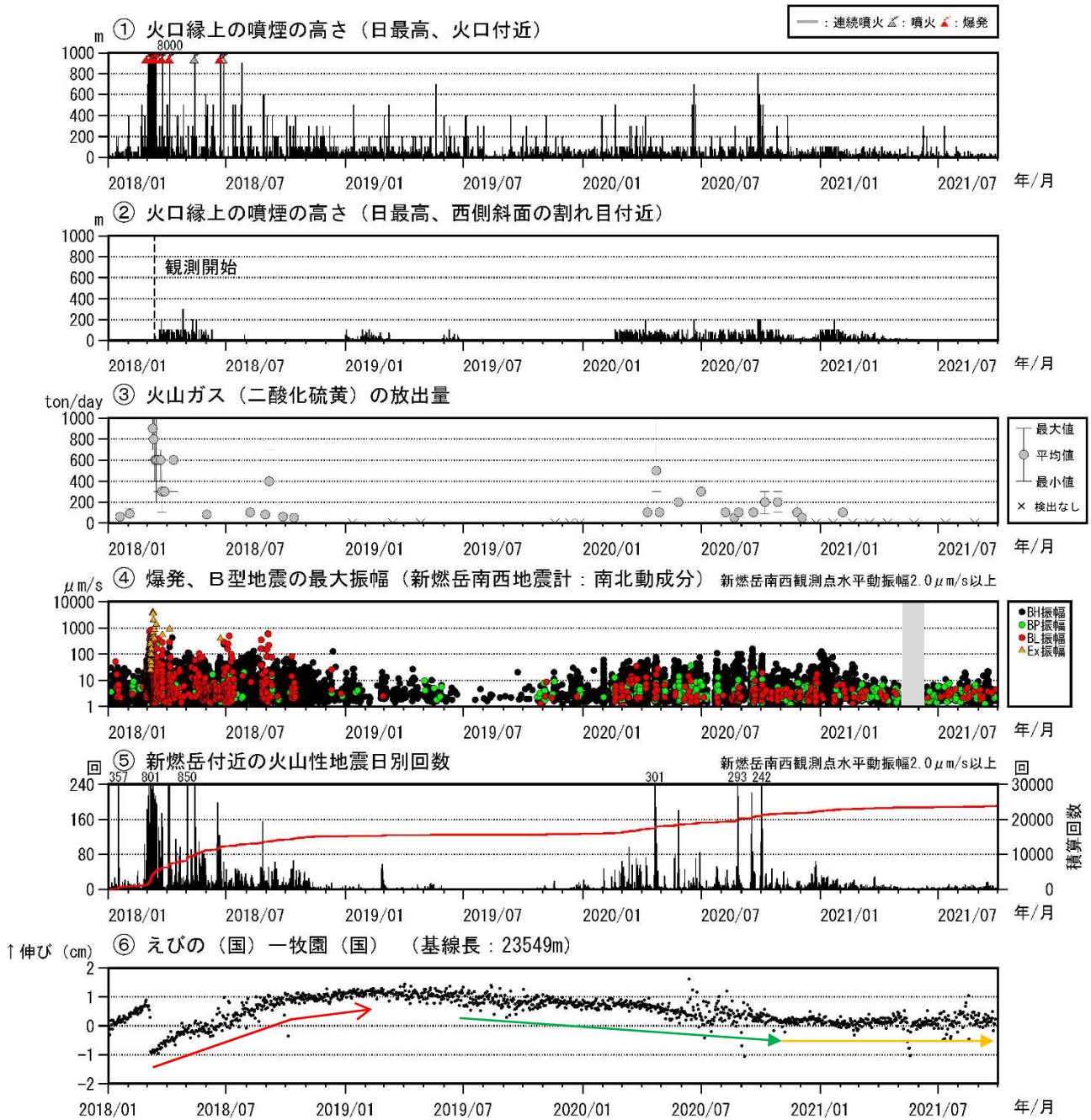
図2 霧島山（新燃岳） 火山活動経過図（2018年1月～2021年9月）
