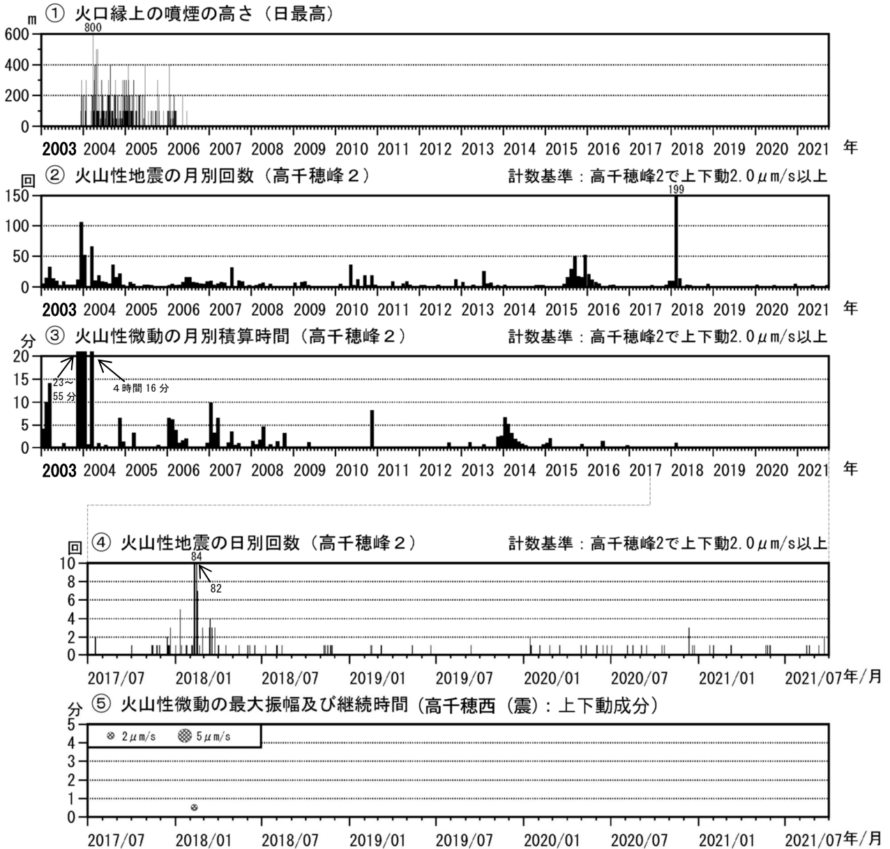
図2 霧島山（御鉢） 火山活動経過図（2003年1月～2021年9月）
