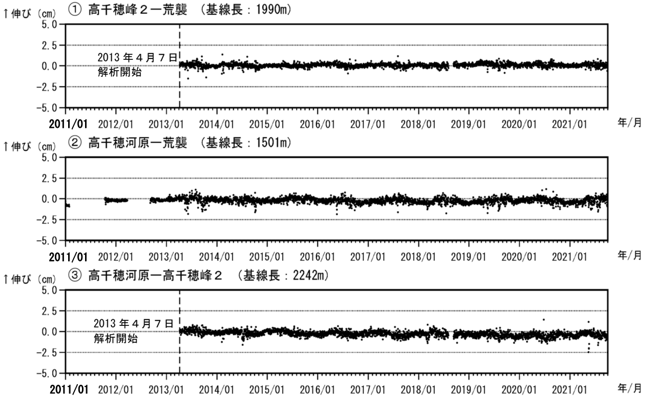
図4 霧島山（御鉢） GNSS 連続観測による基線長変化（2011年1月～2021年9月）
