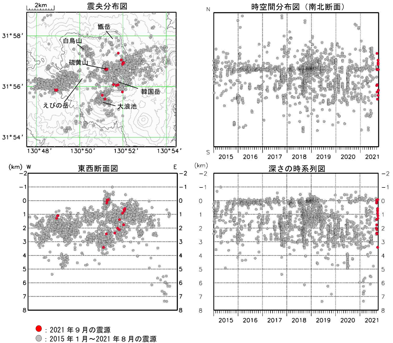
図2 霧島山（えびの高原（硫黄山）周辺） 震源分布図（2015年1月～2021年9月）
