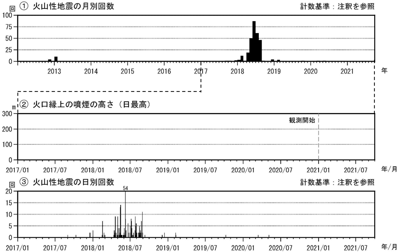
図2 霧島山（大幡池） 火山活動経過図（2012年1月～2021年9月）
