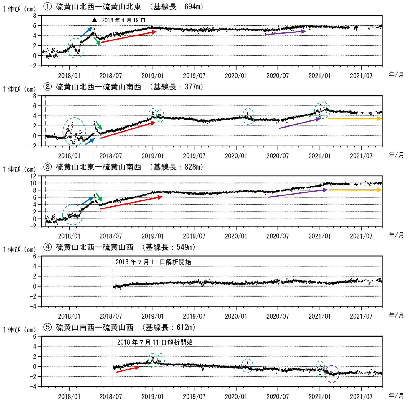
図4 霧島山（えびの高原（硫黄山）周辺） GNSS 連続観測による基線長変化 （2017年9月～2021年9月）
