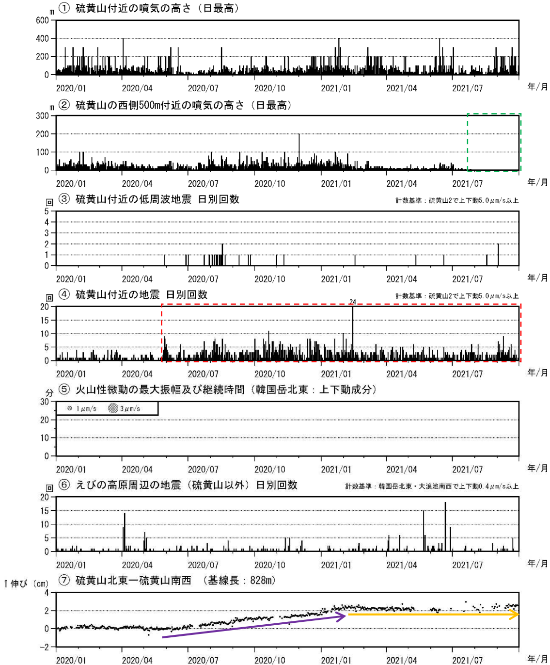
図3 霧島山（えびの高原（硫黄山）周辺）火山活動経過図（2020年1月～2021年9月）
