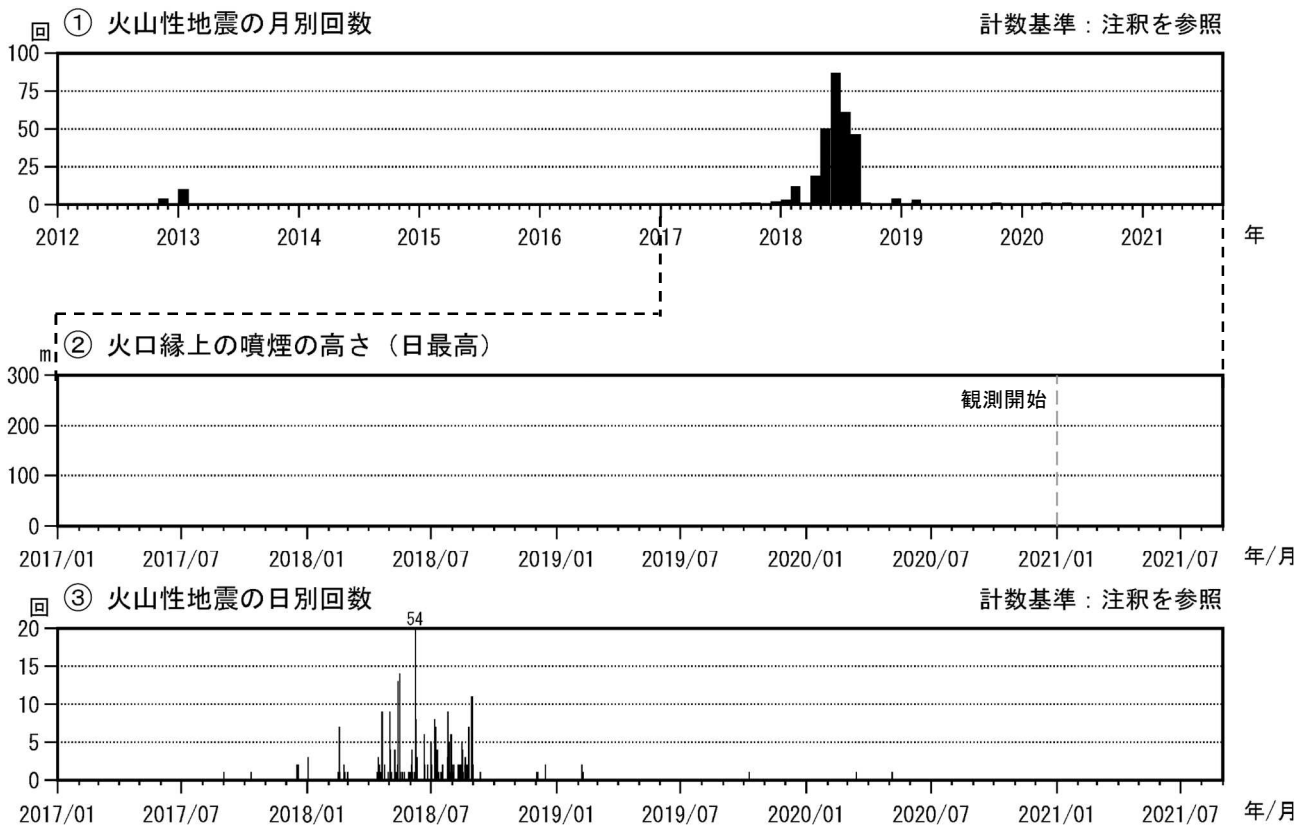
図2 霧島山（大幡池） 火山活動経過図（2012年1月～2021年8月）
