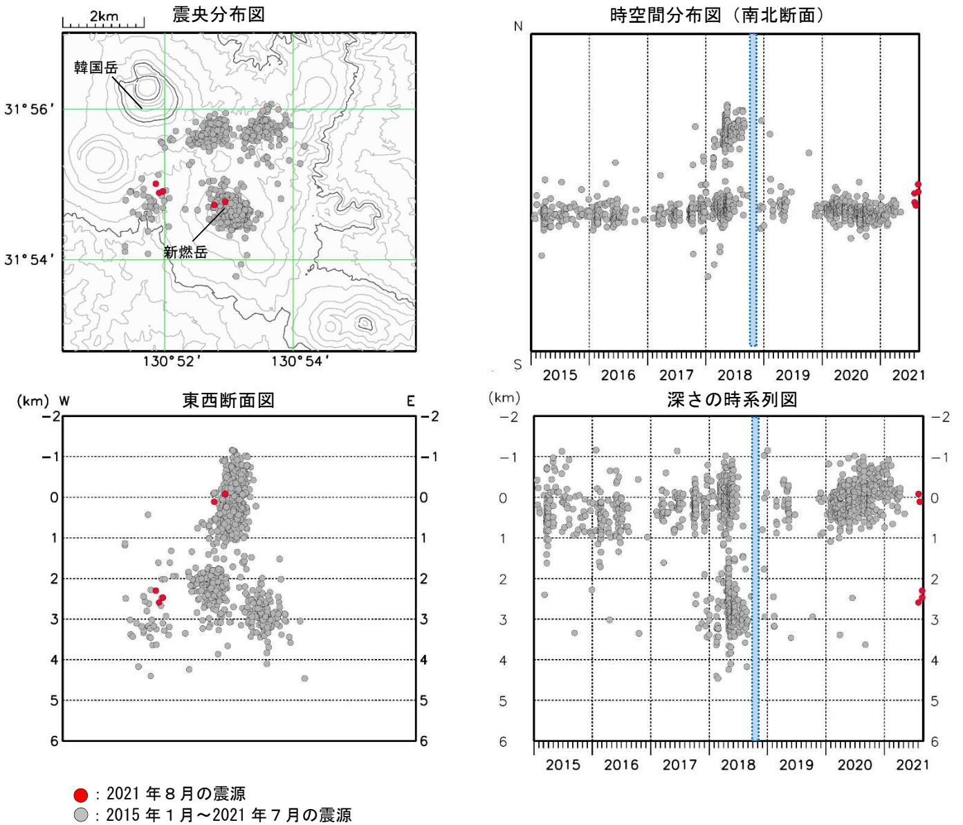
図3 霧島山（新燃岳） 震源分布図（2015年1月～2021年8月）
