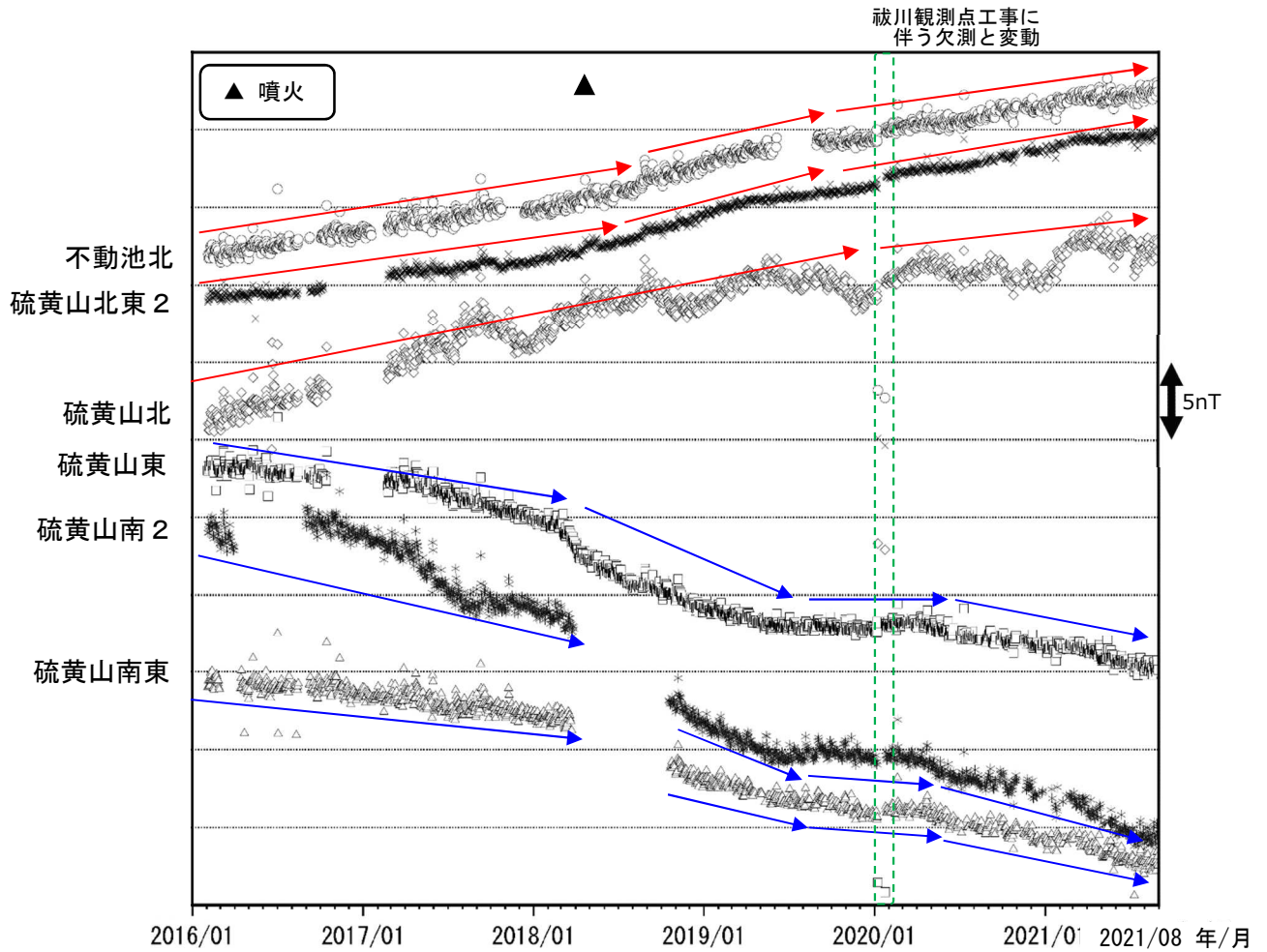
図 8-2 霧島山（えびの高原（硫黄山）周辺） 全磁力観測点で観測された全磁力変動（2016年1月～2021年8月）
