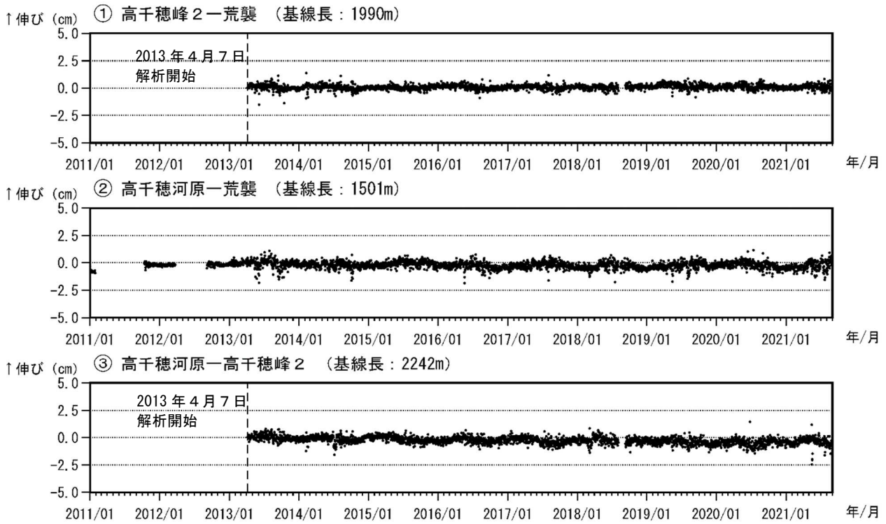
図4 霧島山（御鉢） GNSS 連続観測による基線長変化（2011年1月～2021年8月）
