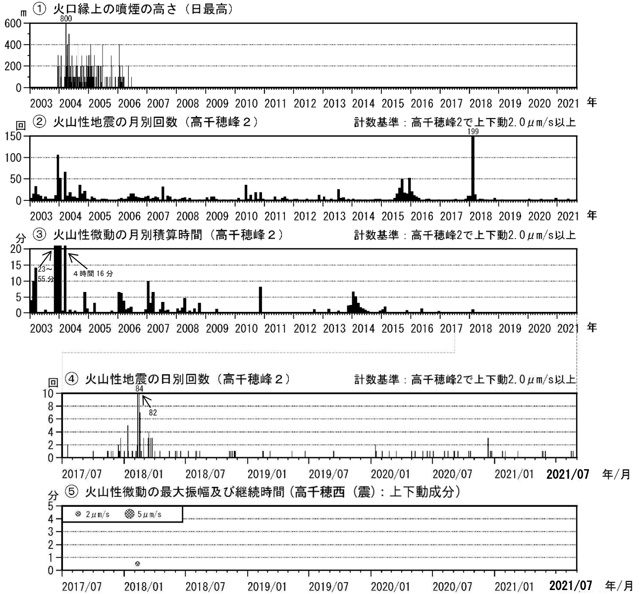
図2 霧島山（御鉢） 火山活動経過図（2003年1月～2021年8月）
