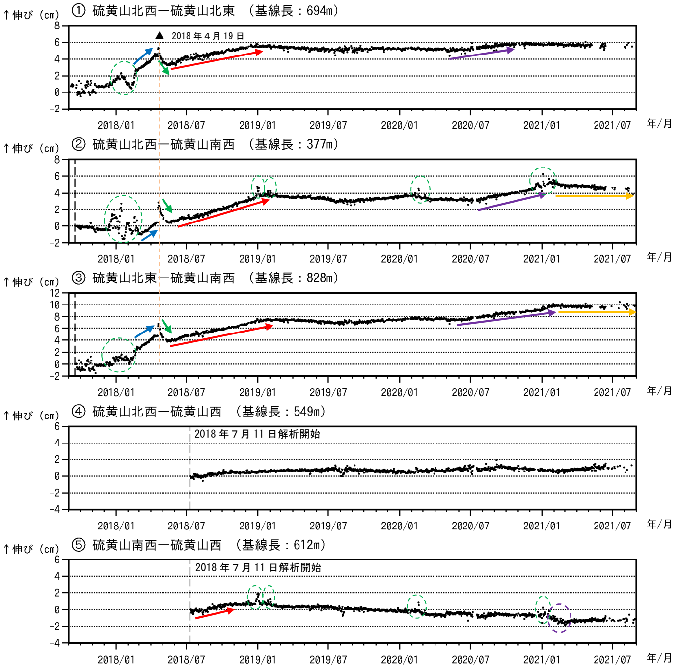
図6 霧島山（えびの高原（硫黄山）周辺） GNSS連続観測による基線長変化 （2017年9月～2021年8月）
