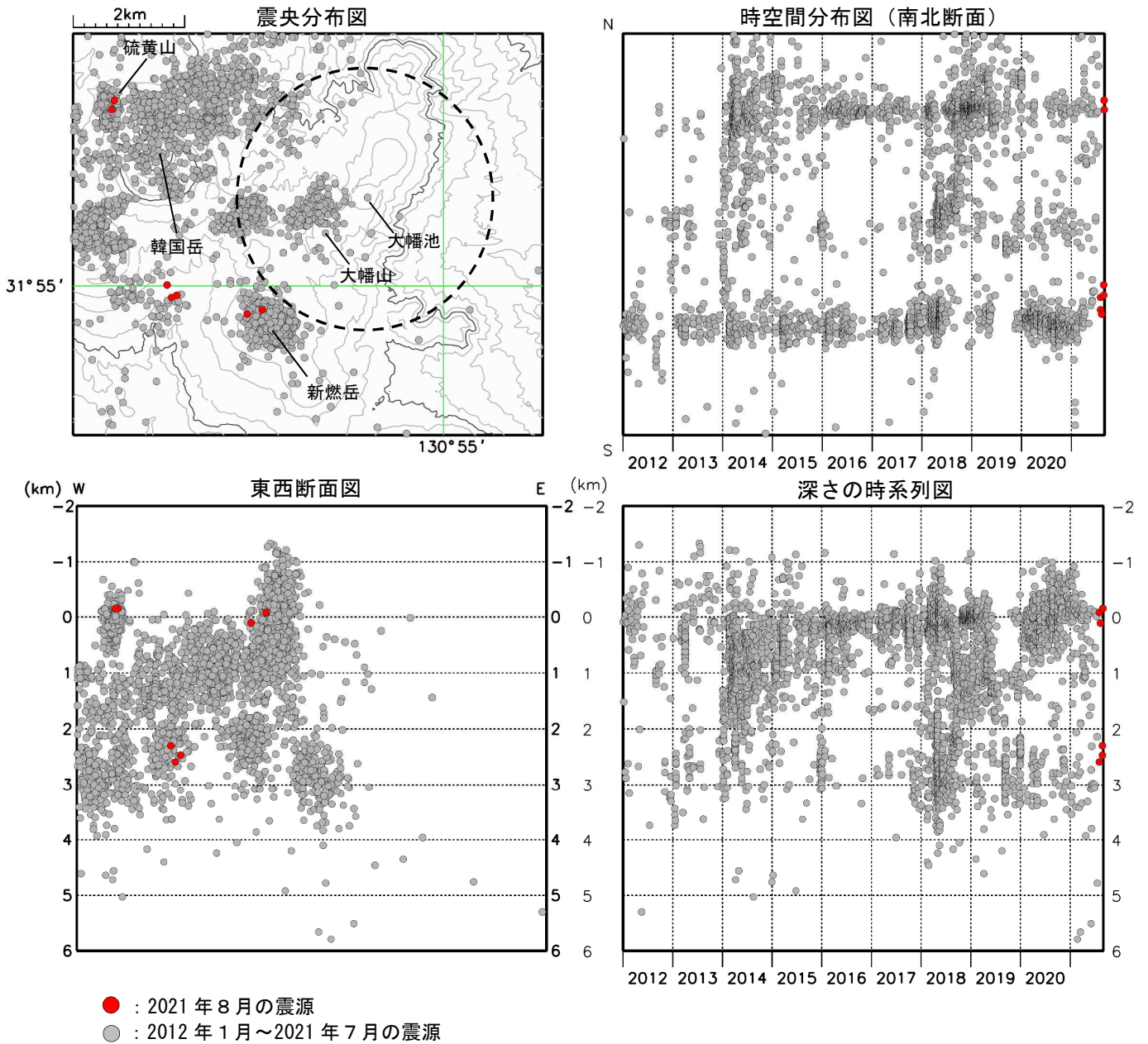
図3 霧島山（大幡池） 震源分布図（2012年1月～2021年8月）
