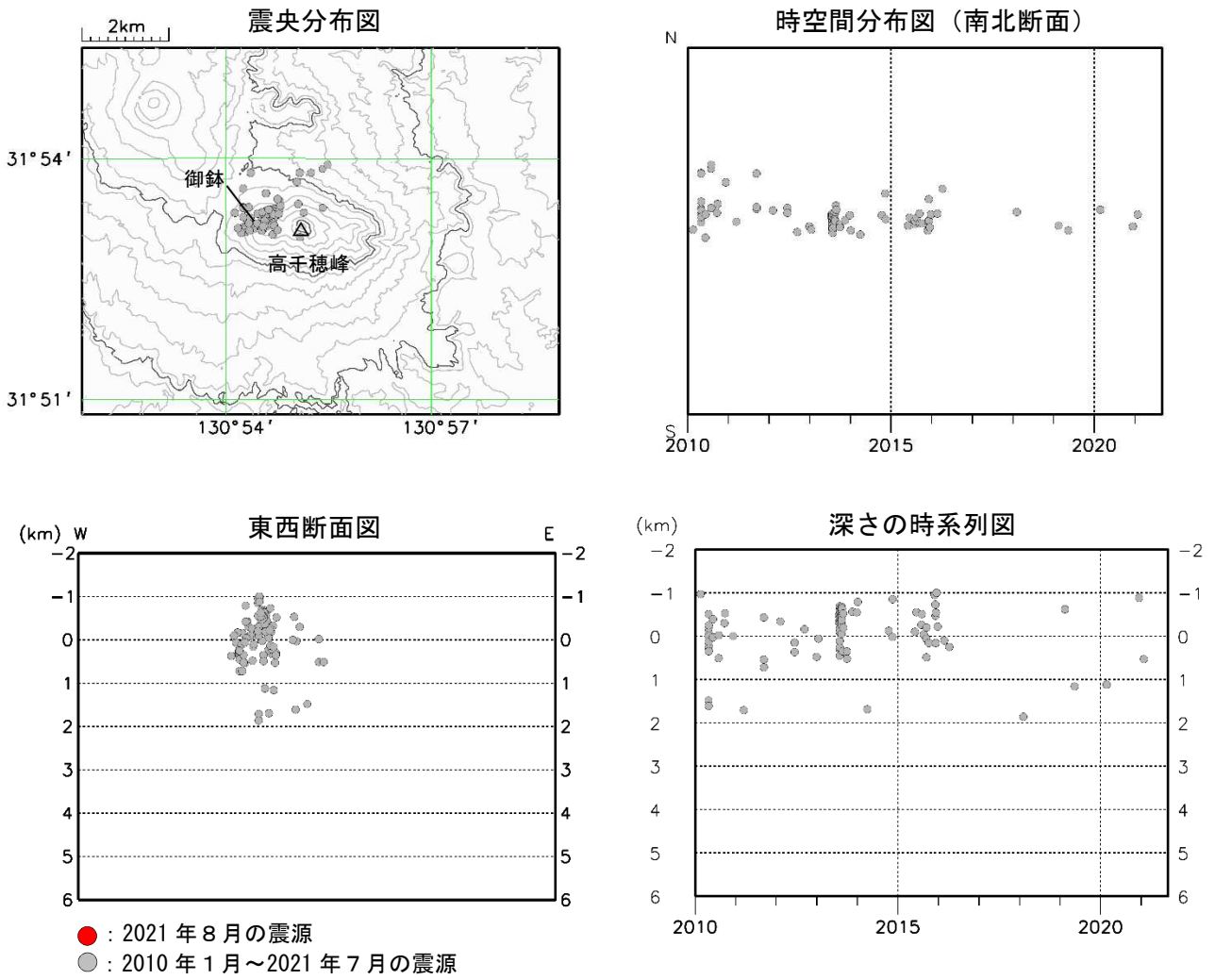
図3 霧島山（御鉢） 震源分布図（2010年1月～2021年8月）
