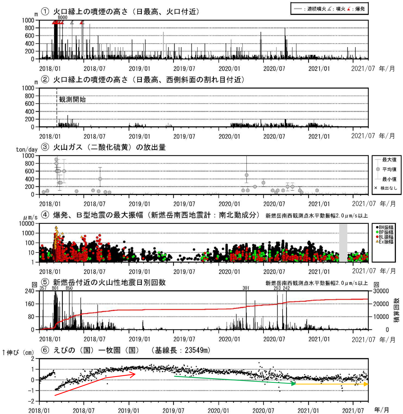
図2 霧島山（新燃岳） 火山活動経過図（2018年1月～2021年8月）
