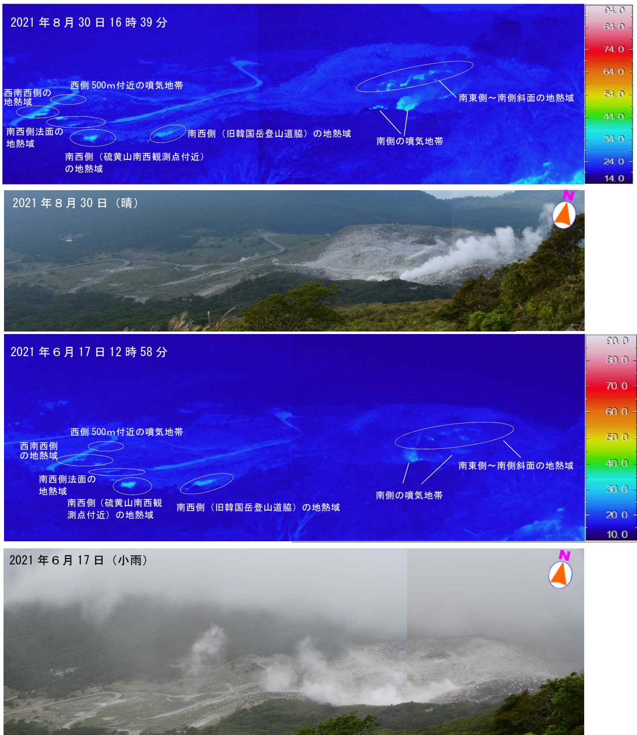
図2 霧島山（えびの高原（硫黄山）周辺） 硫黄山の火口及びその周辺の状況 （韓国岳4合目（図3参照）からの観測）
