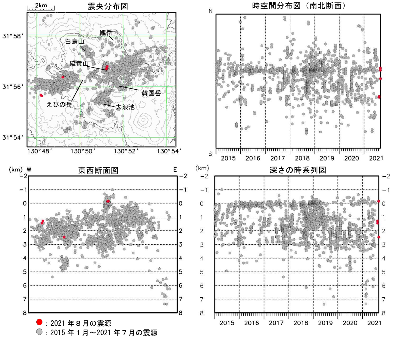
図4 霧島山（えびの高原（硫黄山）周辺） 震源分布図（2015年1月～2021年8月）
