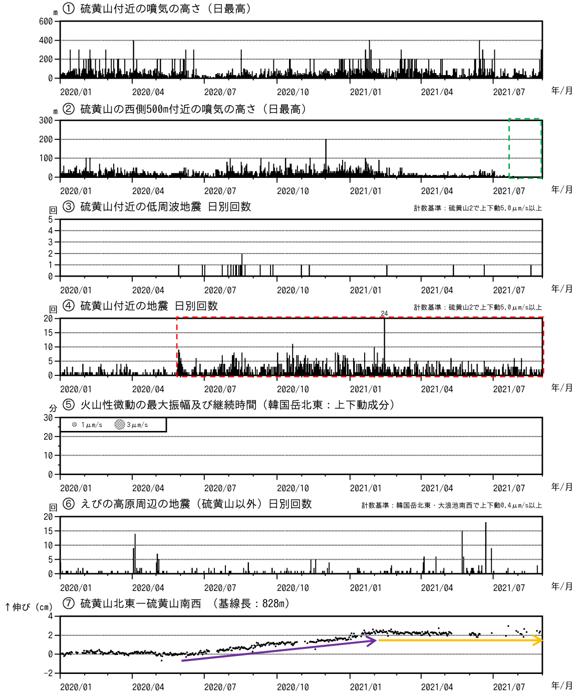
図5 霧島山（えびの高原（硫黄山）周辺）火山活動経過図（2020年1月～2021年8月）
