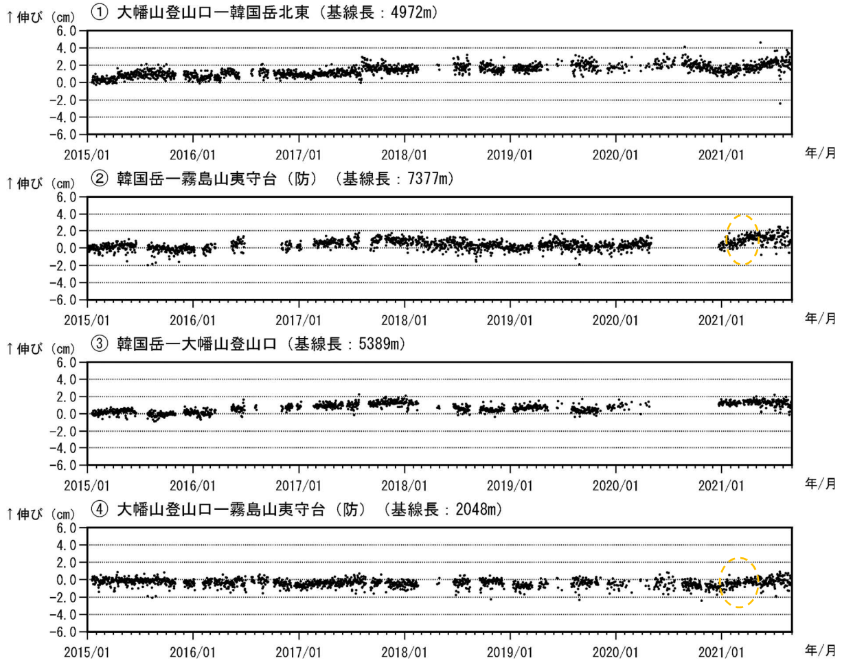
図4 霧島山（大幡池） GNSS 連続観測による基線長変化（2015年1月～2021年8月）
