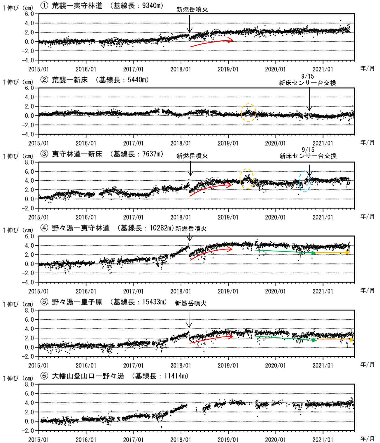
図4 霧島山（新燃岳） GNSS連続観測による基線長変化（2015年1月～2021年8月）
