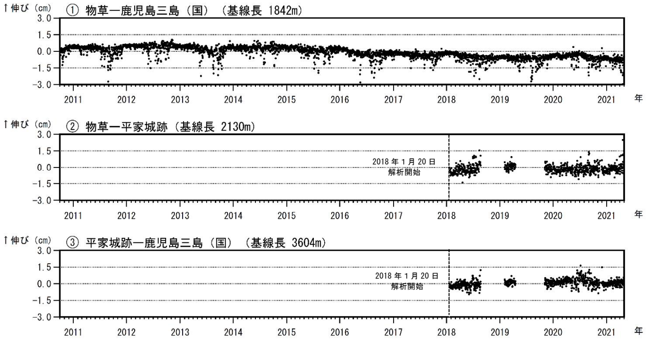
図6 薩摩硫黄島 GNSS連続観測による基線長変化 (2010年10月～2021年4月)
