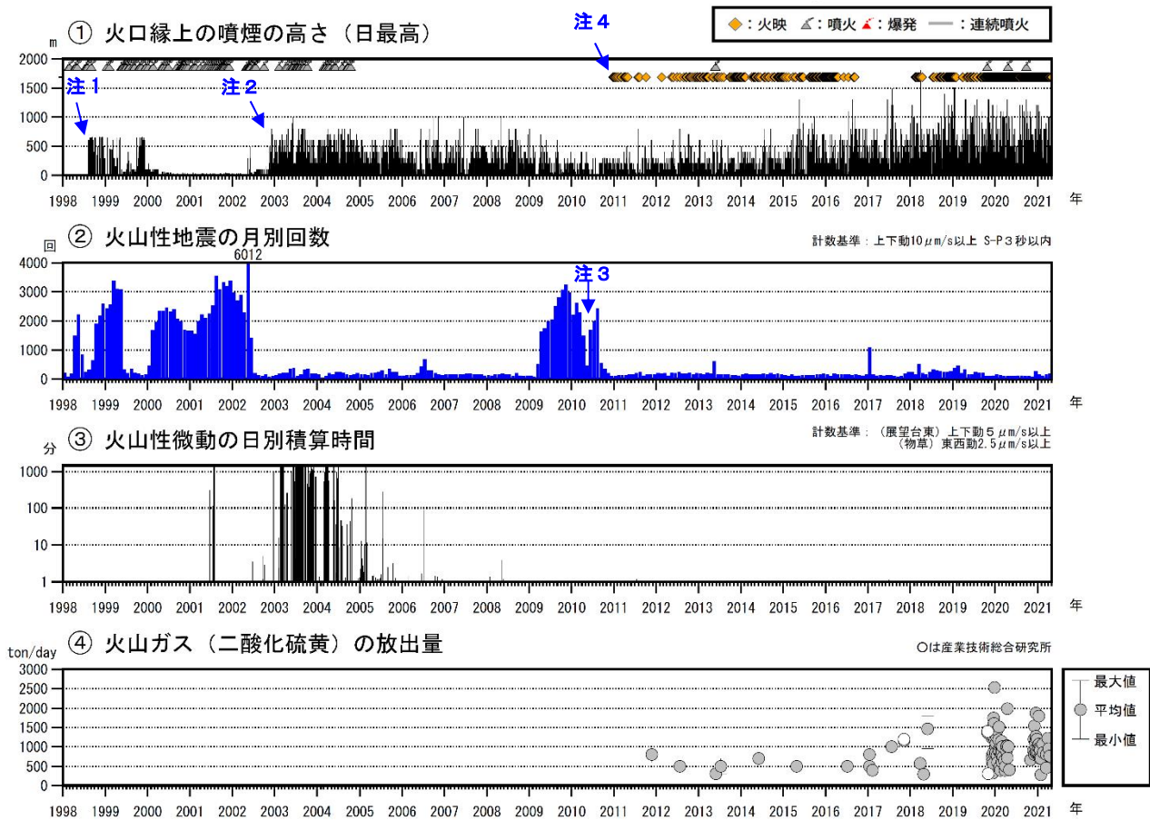
図3 薩摩硫黄島 火山活動経過図（1998年1月～2021年4月）
