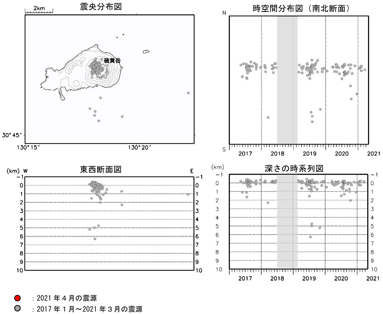
図5 薩摩硫黄島 火山性地震の震源分布図（2017年1月～2021年4月）
