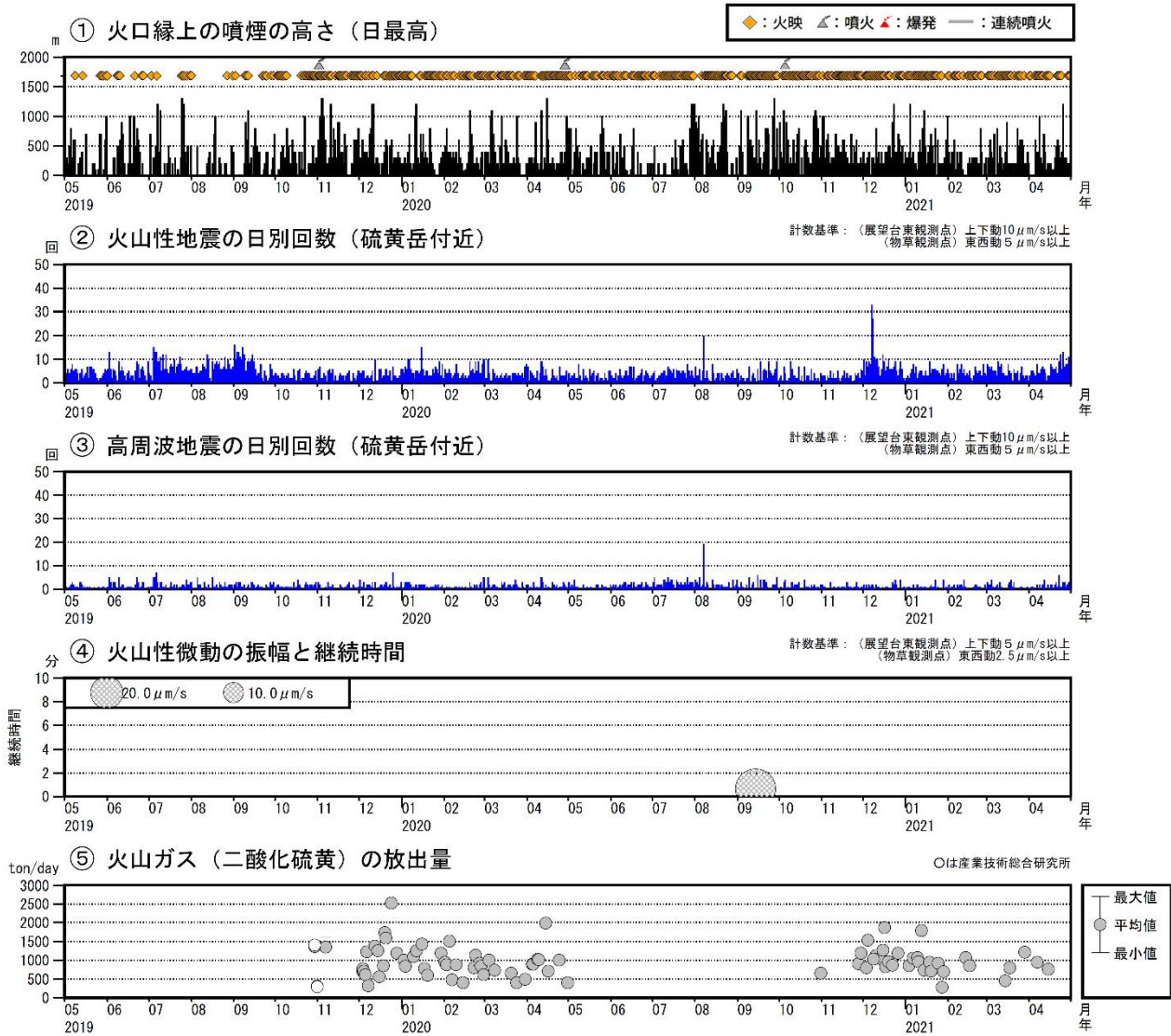
図4 薩摩硫黄島 火山活動経過図（2019年5月～2021年4月）
