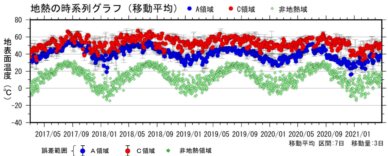
図2-2 九重山 星生山北尾根の赤外熱映像装置による日別最高温度（2017年3月～2021年4月）
