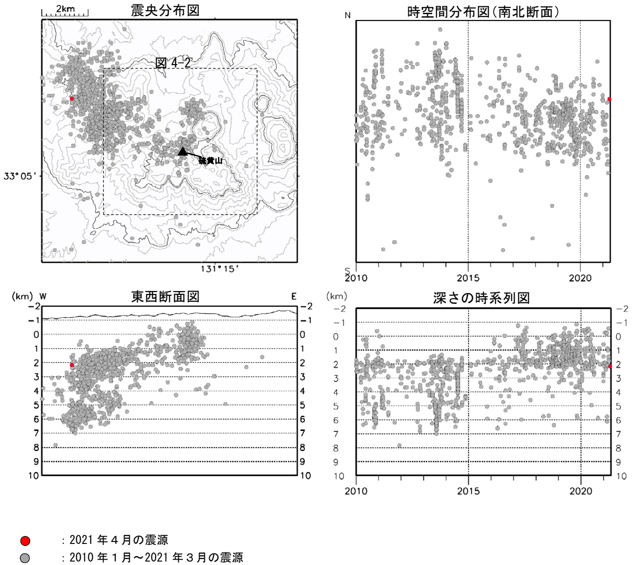
図 4-1 九重山 震源分布図（広域）（2010年1月～2021年4月）
