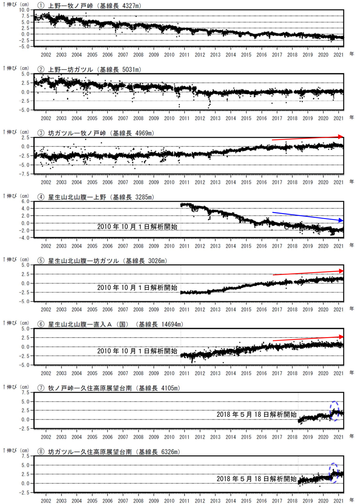
図6 九重山 GNSS連続観測による基線長変化（2001年4月～2021年4月）
