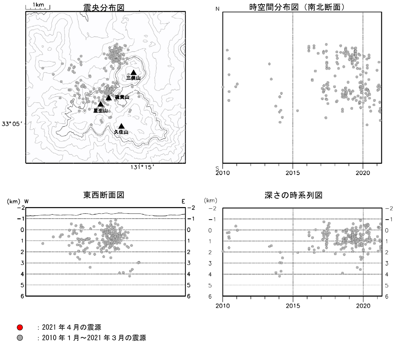
図 4-2 九重山 震源分布図（硫黄山付近）（2010年1月～2021年4月）
