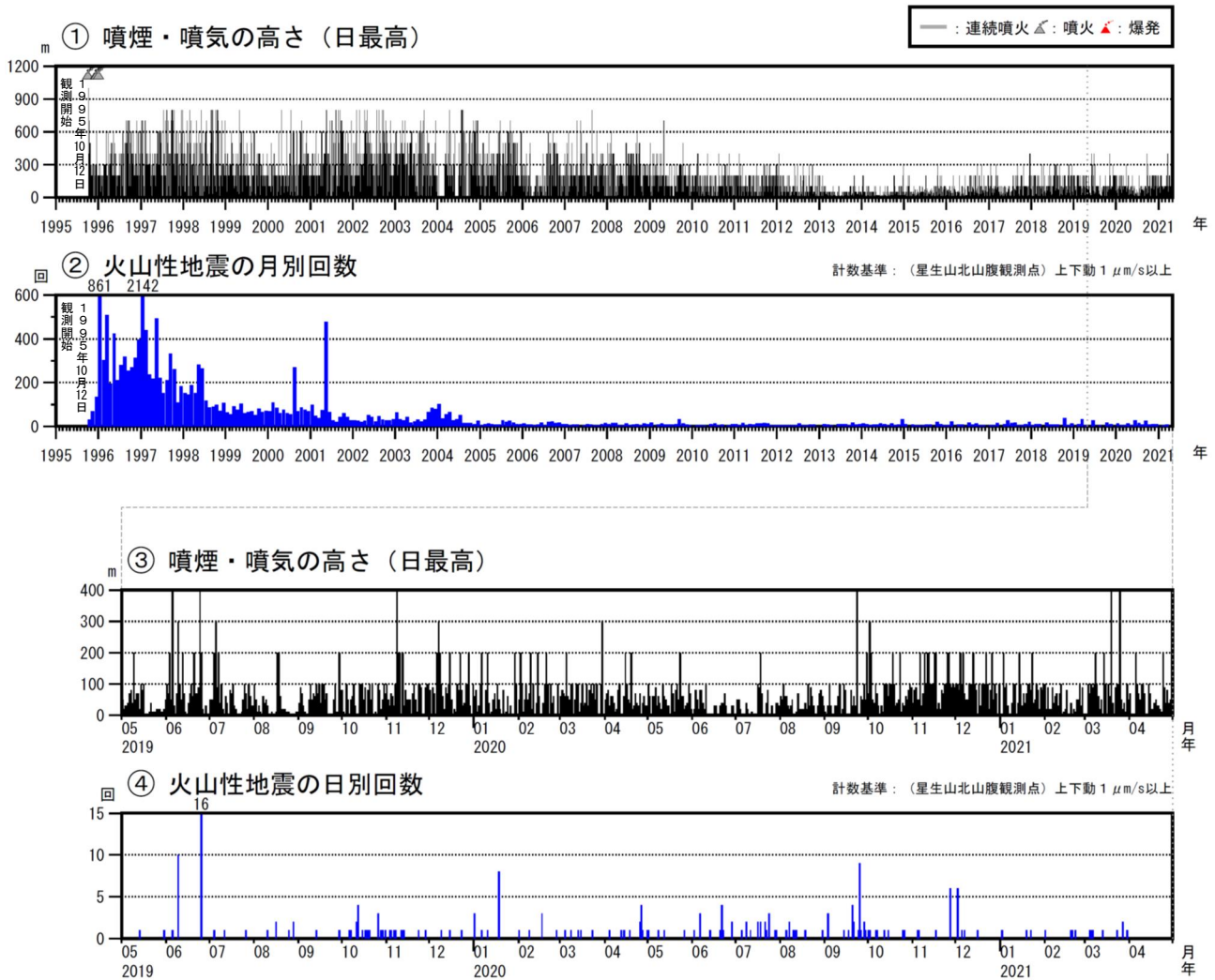
図3 九重山 火山活動経過図（1995年1月～2021年4月）
