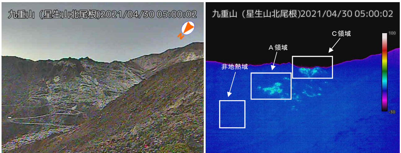
図2-1 九重山 硫黄山の噴気および地熱域の状況（4月30日 星生山北尾根監視カメラ）
