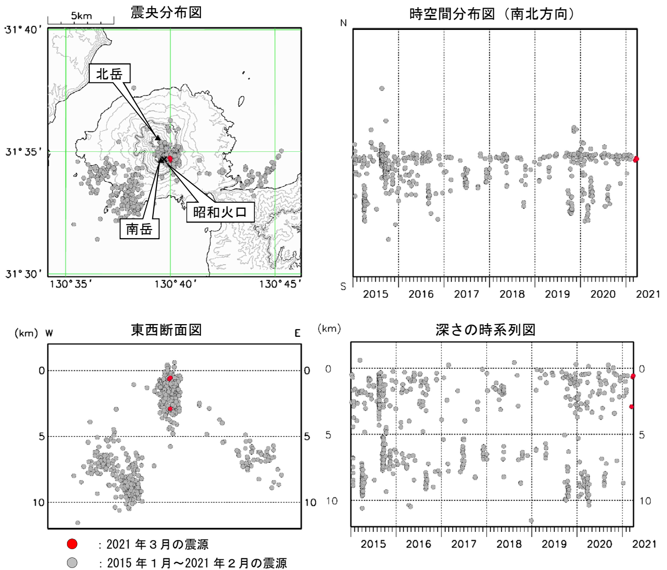
図4 桜島 震源分布図（2015年1月～2021年3月）
