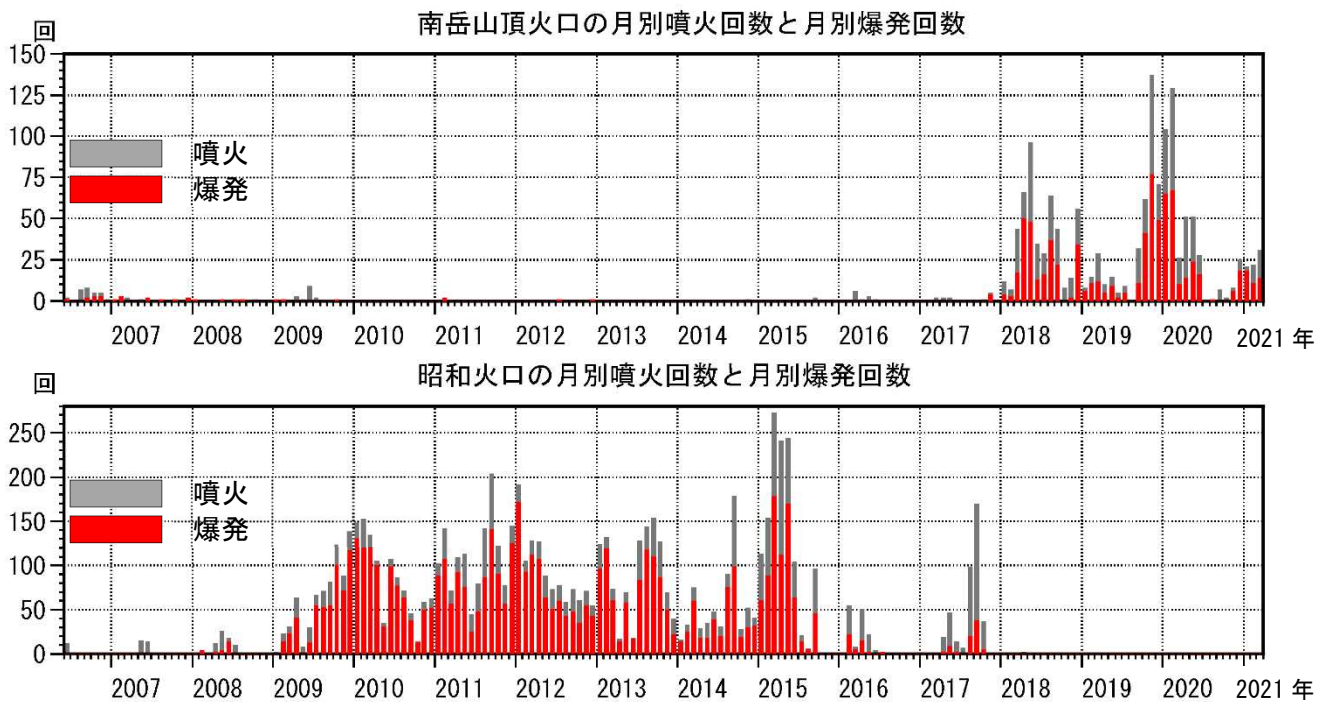
図 5-2 桜島 南岳山頂火口（上図）と昭和火口（下図）の月別噴火回数と月別爆発回数 （2006年6月～2021年3月）
