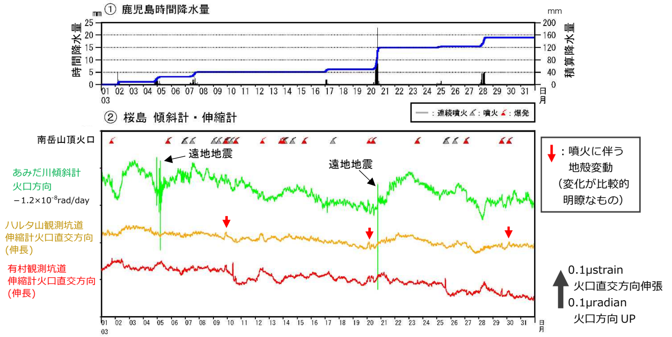
図7 桜島 傾斜計及び伸縮計による地殻変動の状況（2021年3月）
