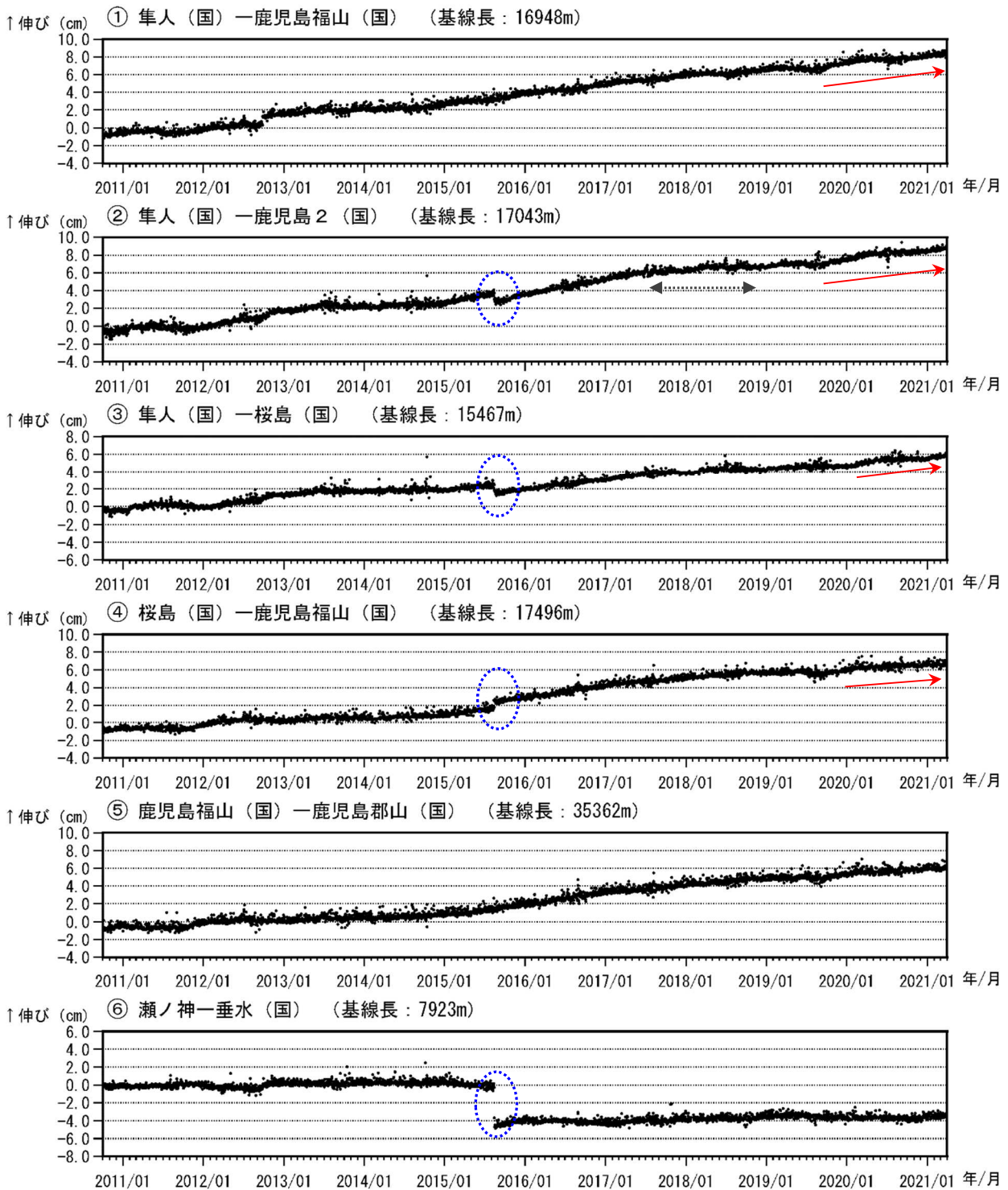
図 8-1 桜島 GNSS 連続観測による基線長変化（2010 年 10 月～2021 年 3 月）
