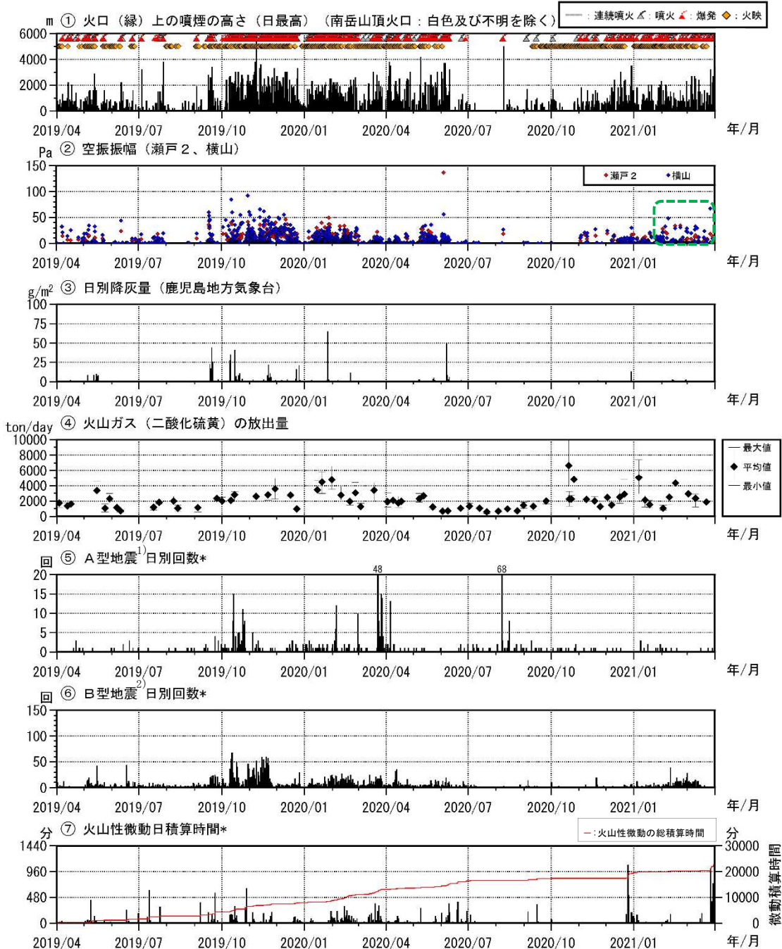
図6 桜島 最近2年間の活動経過図（2019年4月～2021年3月）
