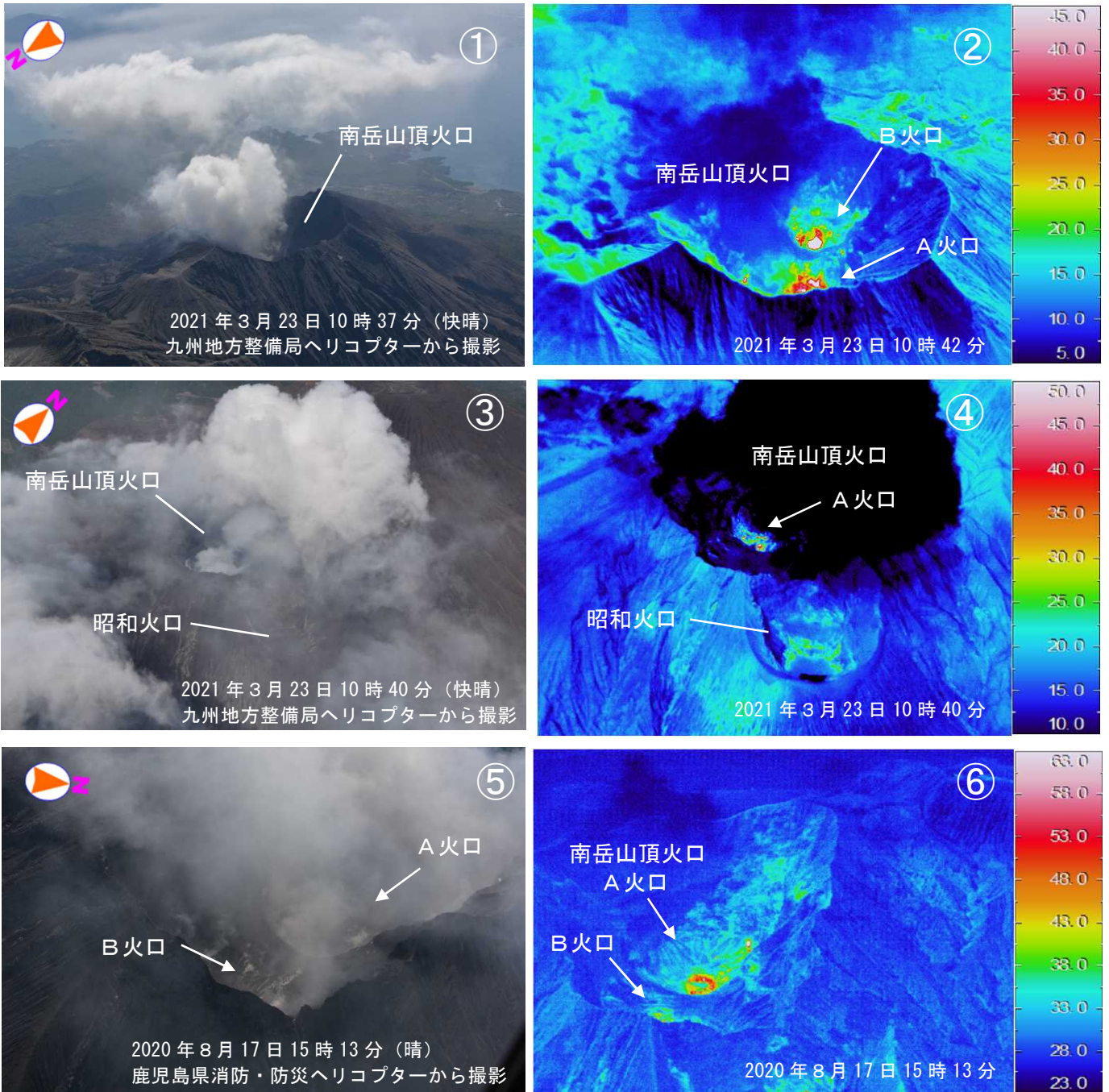
図2 桜島 上空から観測した南岳山頂火口及び昭和火口の状況
