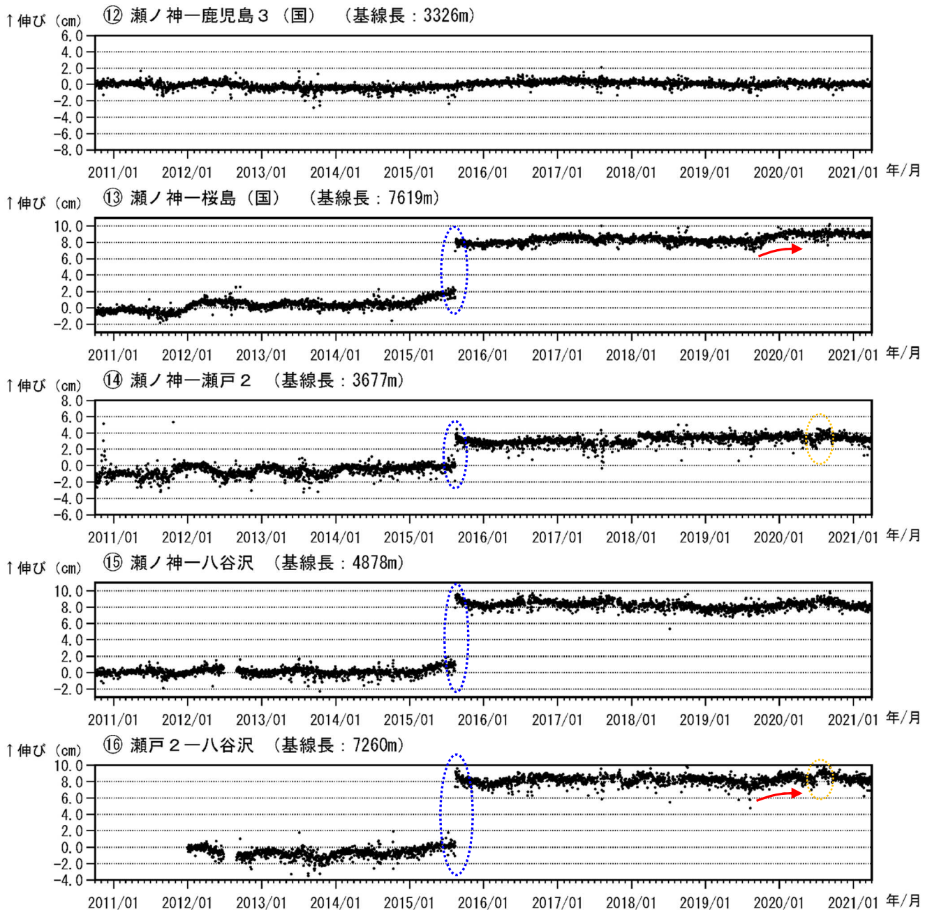
図 8-3 桜島 GNSS 連続観測による基線長変化（2010 年 10 月～2021 年 3 月）
