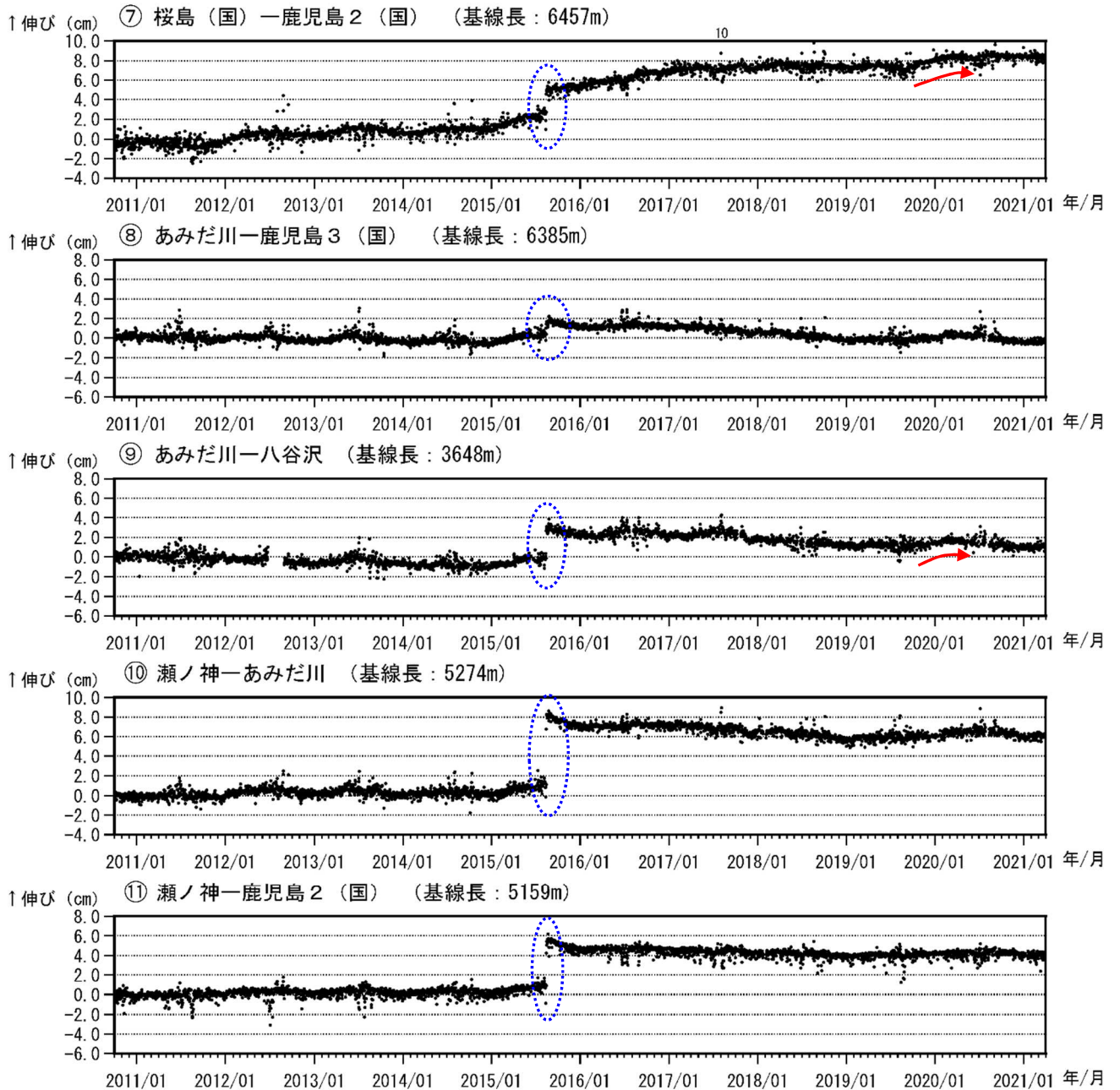
図8-2 桜島 GNSS 連続観測による基線長変化（2010年10月～2021年3月）
