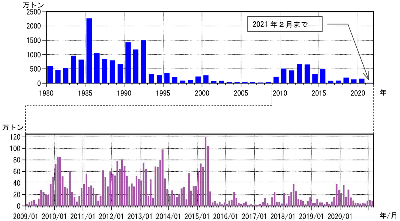
図10 桜島 鹿児島県が実施している降灰の観測データから推定した火山灰の総噴出量 (上段：1980年1月～2021年2月の年別値、下段：2009年1月～2021年2月の月別値)
