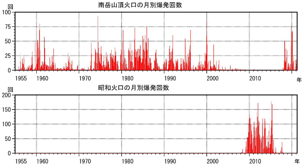
図 5-1 桜島 南岳山頂火口（上図）と昭和火口（下図）の月別爆発回数 （1955年1月～2021年3月）
