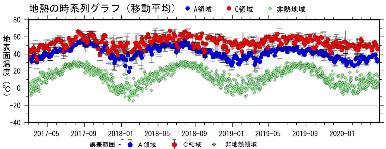
図2-2 九重山 星生山北尾根の赤外熱映像装置による日別最高温度（2017年4月～2020年4月） A領域、C領域ともに非地熱領域と比べて地表面温度が高い状態が続いています。
