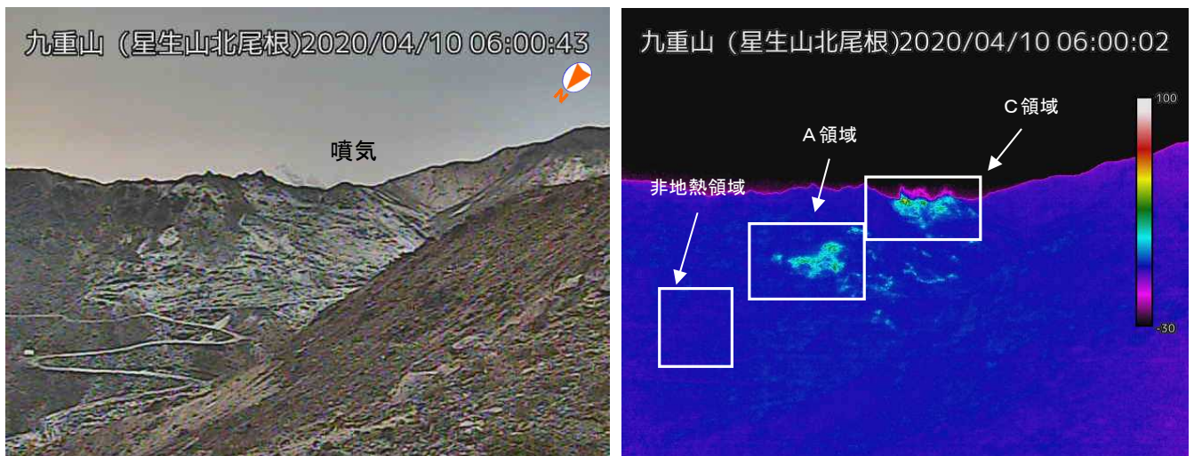
図2-1 九重山 噴気および地熱域の状況 （4月10日 星生山北尾根高感度カメラ（左）及び赤外熱映像装置による（右））
