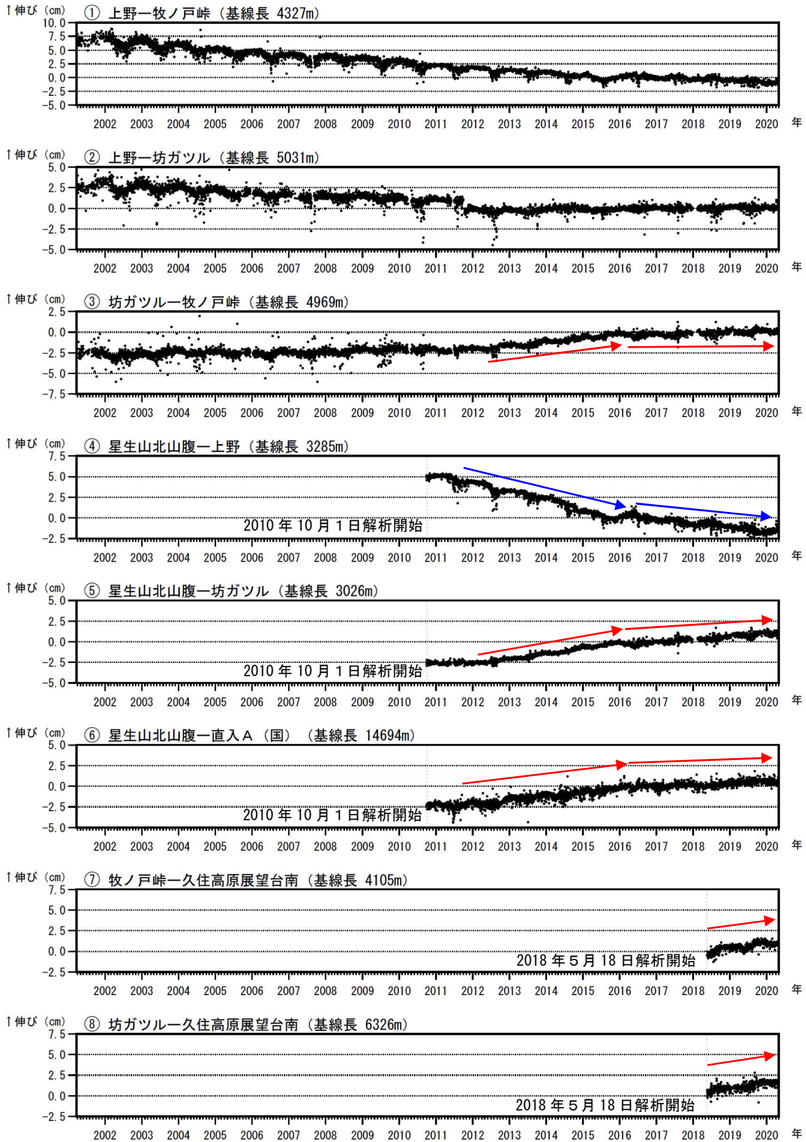
図8 九重山 GNSS連続観測による基線長変化（2001年4月～2020年4月）
