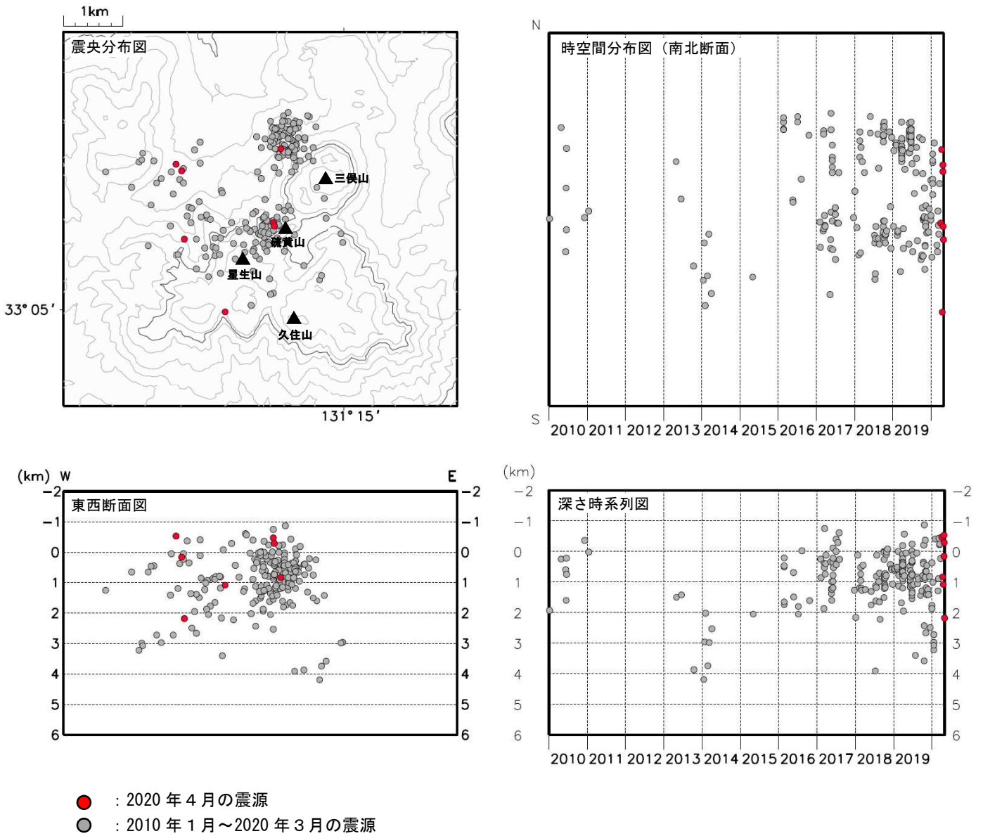
図 4-2 九重山 震源分布図（硫黄山付近の火山性地震）（2010年1月～2020年4月）
