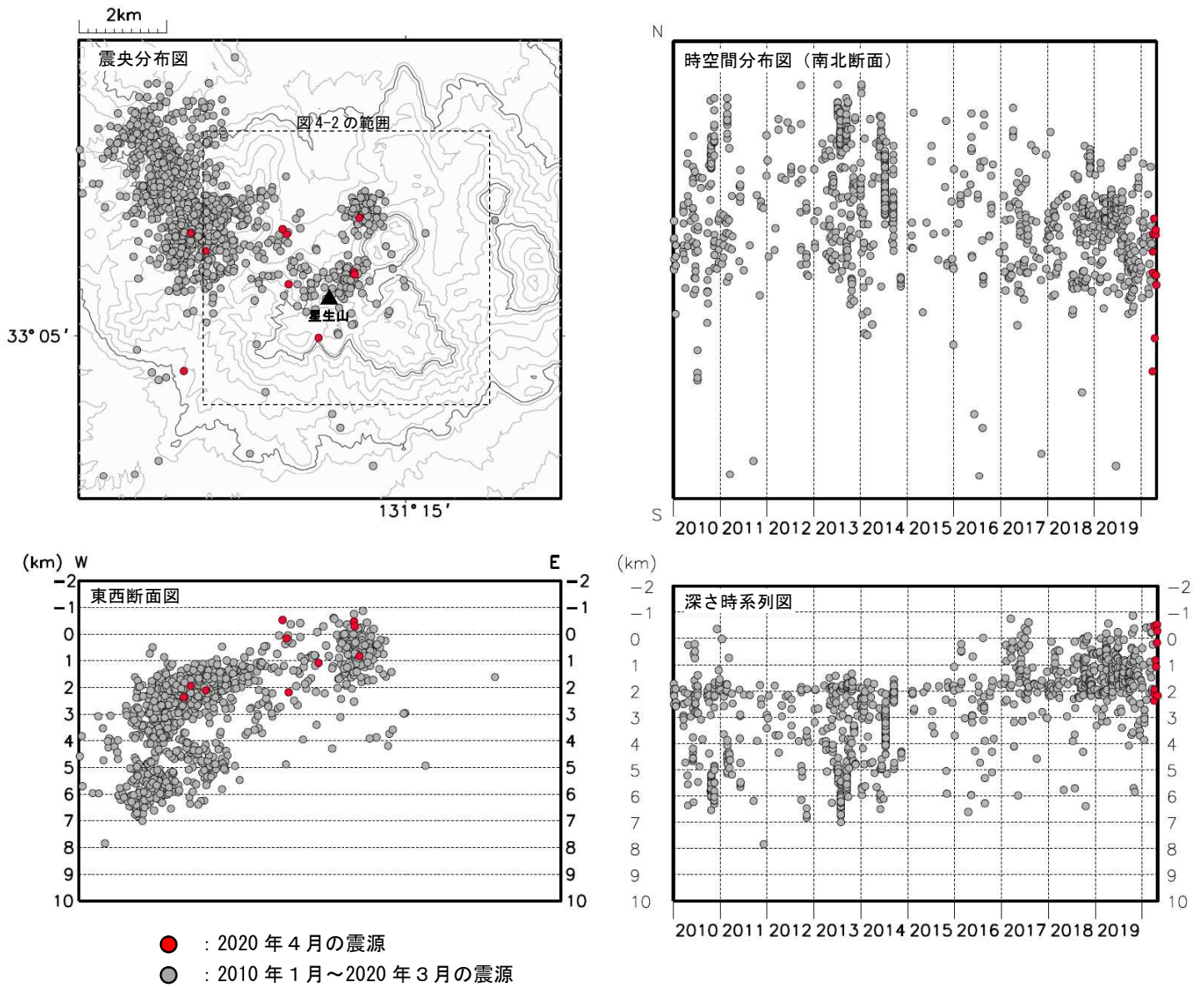
図4-1 九重山 震源分布図（広域）（2010年1月～2020年4月）
