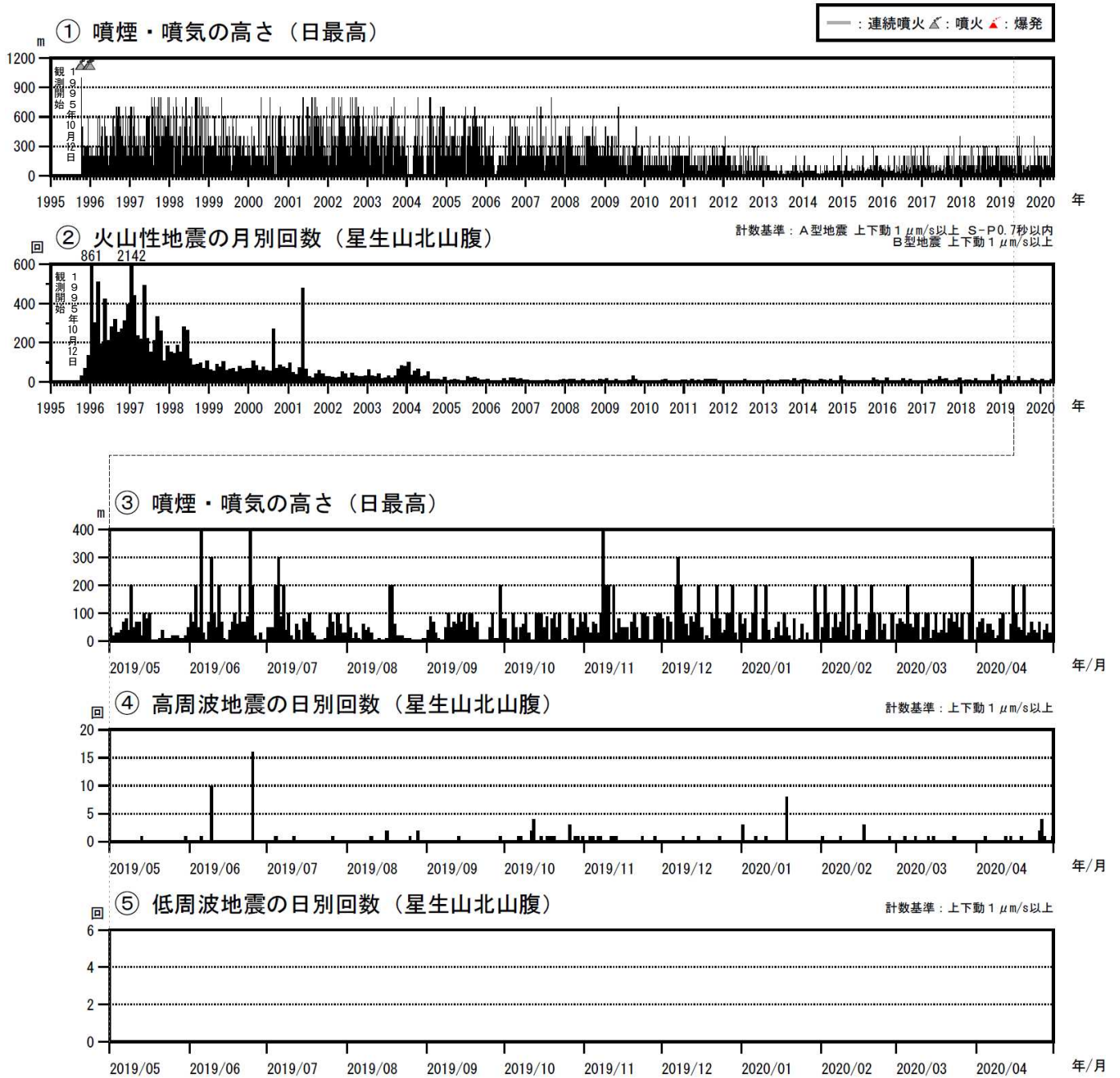
図3 九重山 火山活動経過図（1995年1月～2020年4月）
