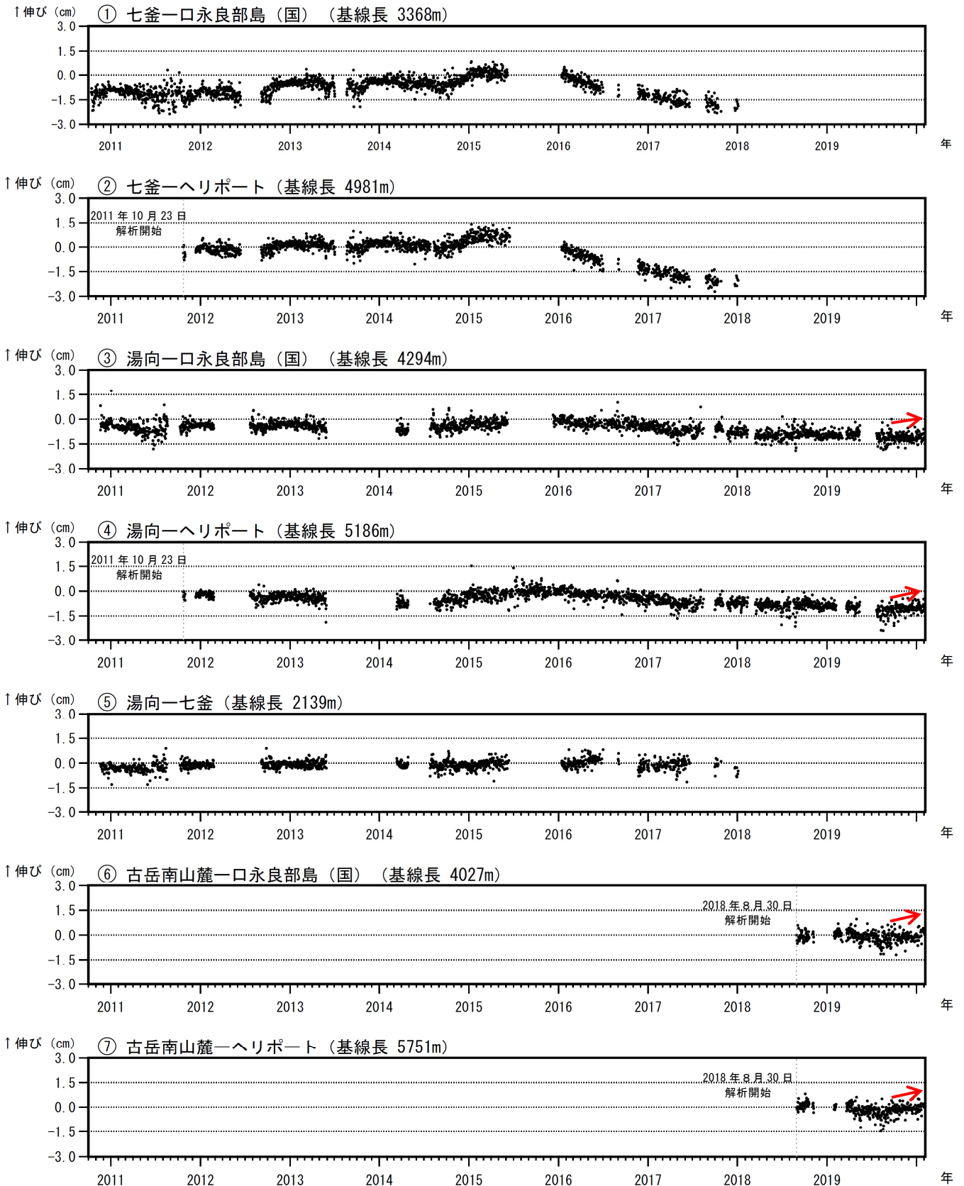
図 24 口永良部島 GNSS 連続観測による基線長変化（2010 年 10 月～2020 年 2 月 3 日）
