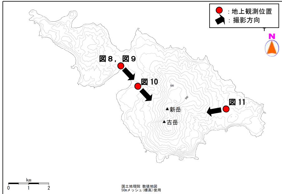
図7 口永良部島 現地調査観測位置及び撮影方向
