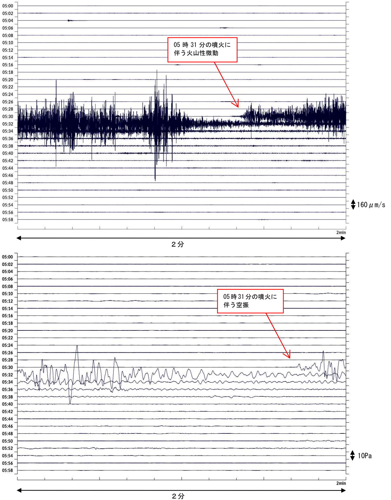
図 21 口永良部島 地震波形及び空振波形
