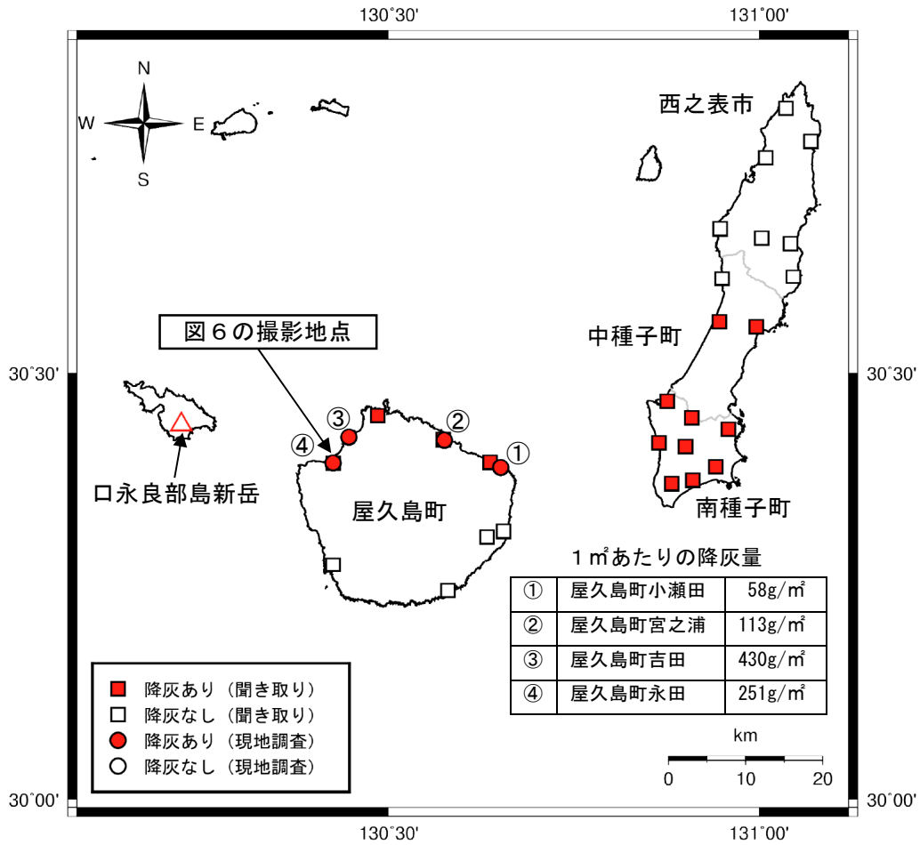
図5 口永良部島 降灰分布図及び降灰量
