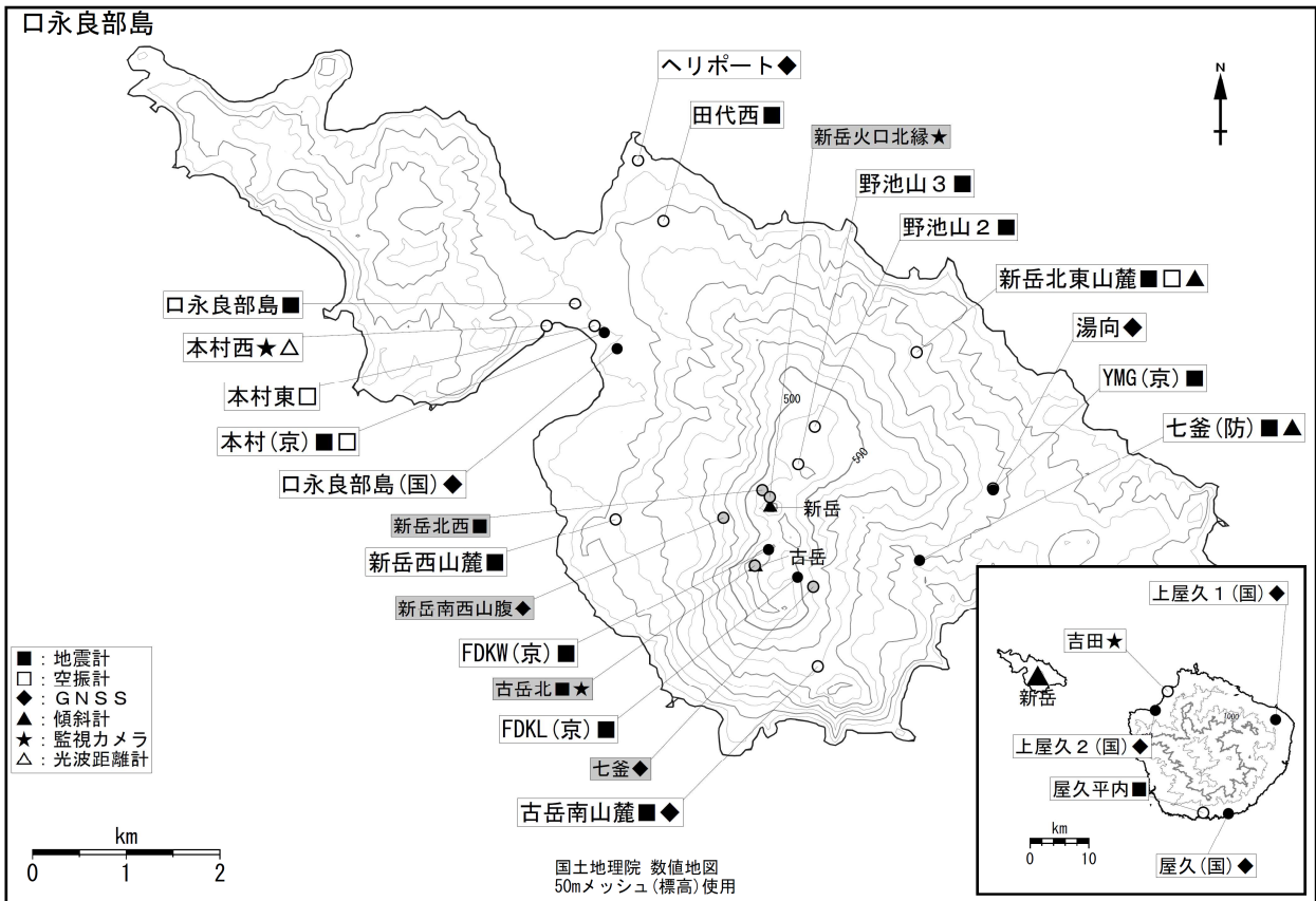
図 26 口永良部島 観測点配置図
