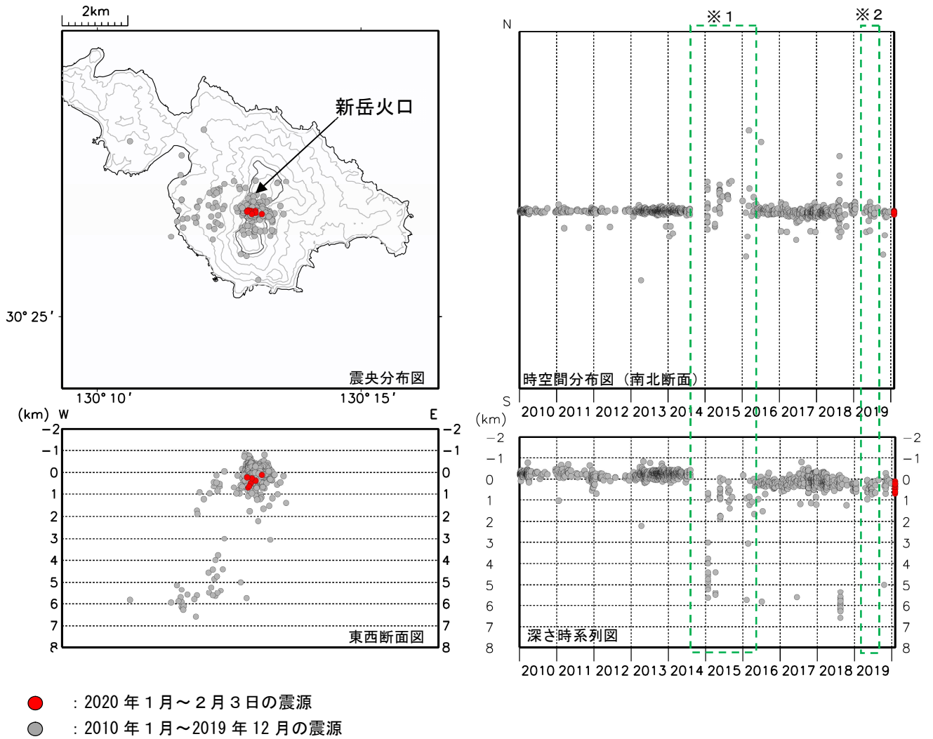
図18 口永良部島 震源分布図（2010年1月～2020年2月3日）
