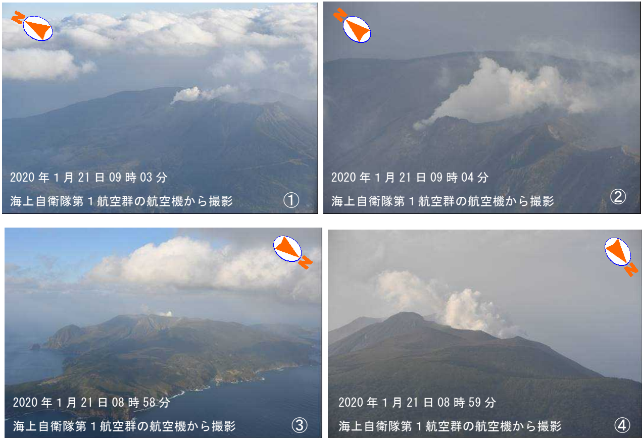
図12 口永良部島 上空から観測した新岳火口の状況（1月21日）
