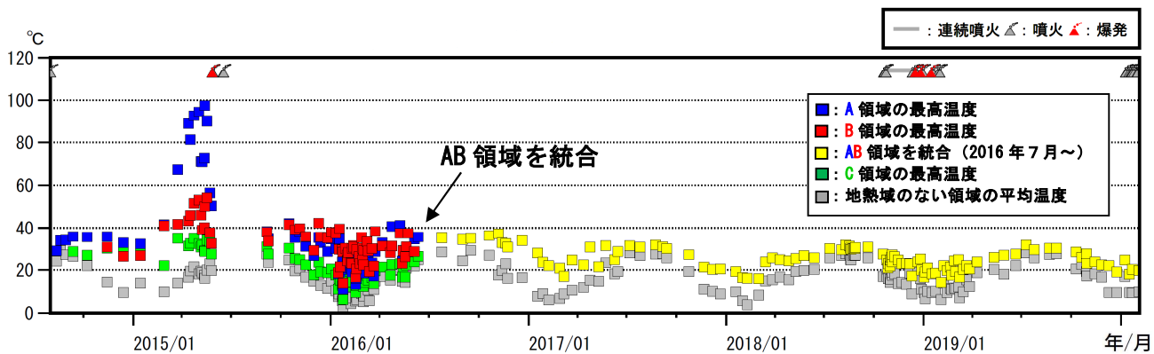
図8 口永良部島 新岳西斜面及び新岳南西側斜面の地熱域の温度時系列(2014年8月～2020年2月3日)
