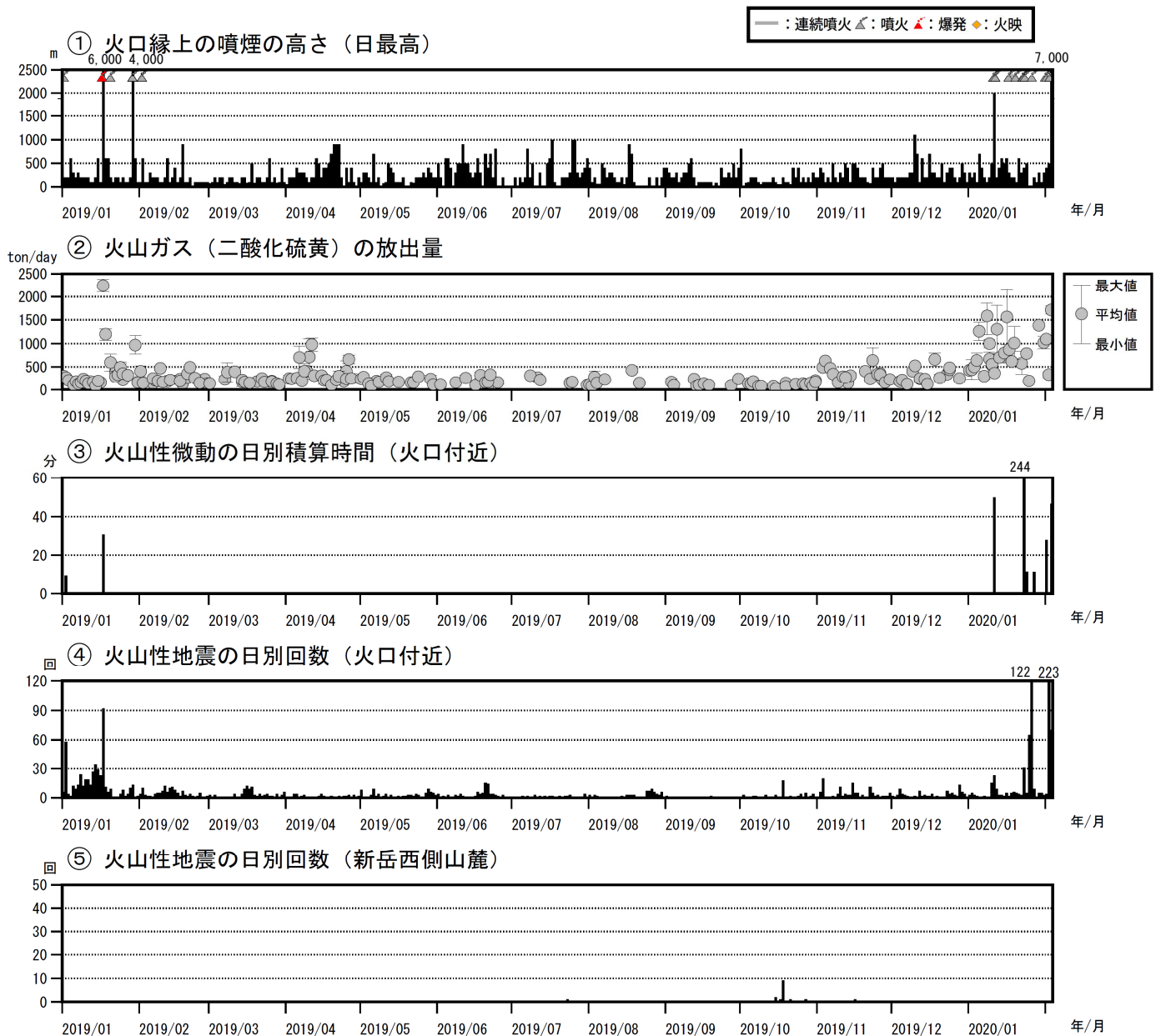
図 17 口永良部島 最近の火山活動経過図（2019年1月～2020年2月3日）
