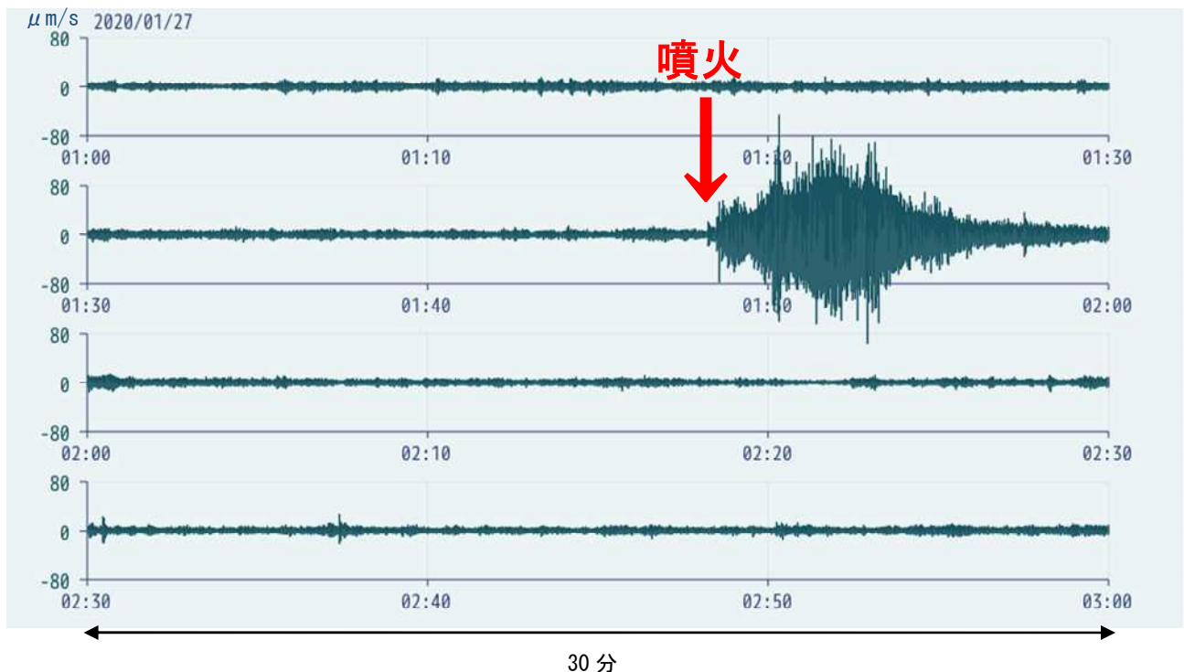
図 20 口永良部島 地震波形（FDKL（京）観測点：上下動 1月27日01時00分～03時00分） 1月27日にやや規模の大きな噴火が発生し火山性微動が発生しました。噴火の規模は2019年1月17日の噴火より小さいと推定されます。
