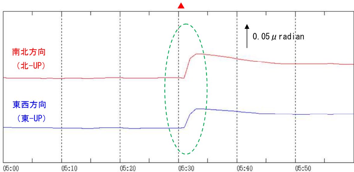
図23 口永良部島 新岳北東山麓観測点傾斜計の傾斜変動（2月3日05時00分～06時00分）
