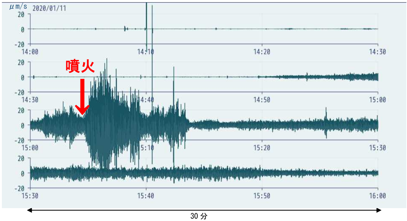
図 19 口永良部島 地震波形（野池山3観測点：上下動 1月11日14時00分～16時00分） 火山性微動は、1月11日の噴火が発生する前から振幅が次第に大きくなり、噴火発生に伴いさらに大きくなりました。
