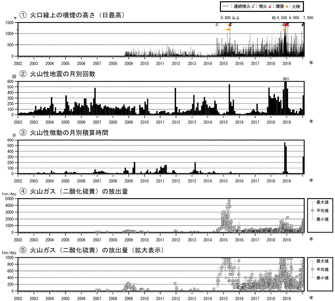
図 16 口永良部島 火山活動経過図（2002年1月～2020年2月3日）
