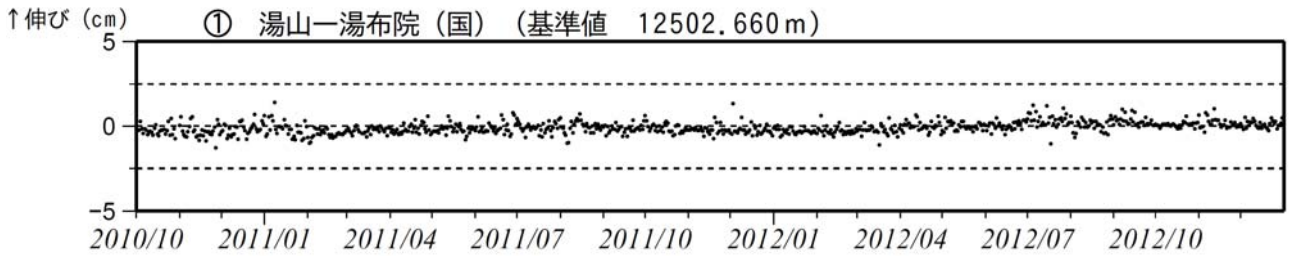
図 2※ 鶴見岳・伽藍岳 GPS連続観測による基線長変化 (2010年10月～2012年12月) 火山活動によると考えられる変化は認められませんでした。
