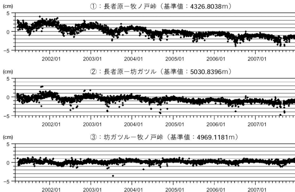
図3 九重山 GPS 連続観測による基線長変化図(2001年3月1日～2007年12月31日)
