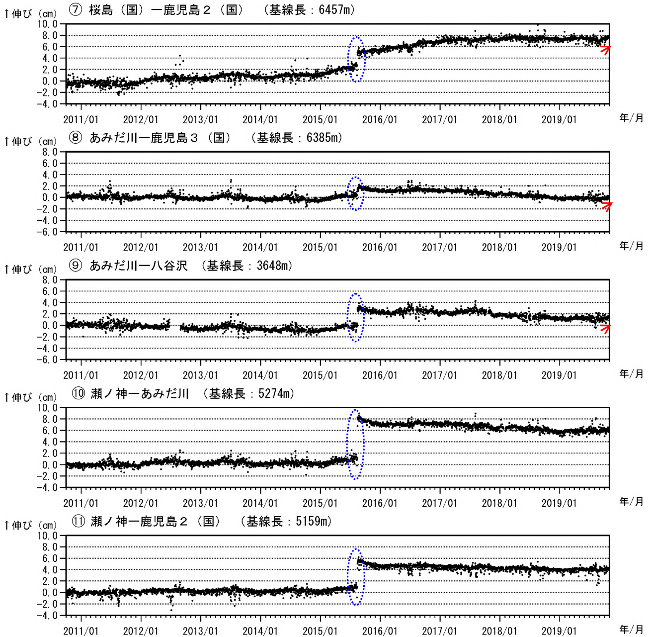
図 7-2 桜島 GNSS 連続観測による基線長変化（2010 年 11 月～2019 年 10 月）
