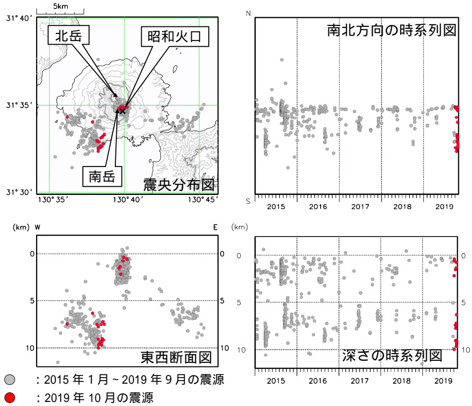
図5 桜島 震源分布図(2015年1月～2019年10月)
