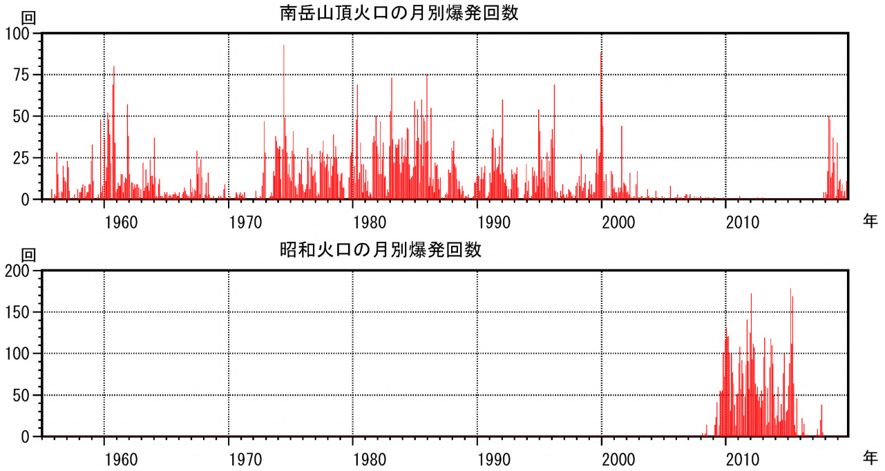
図 3-1 桜島 南岳山頂火口（上図）と昭和火口（下図）の月別爆発回数 （1955年1月～2019年10月）
