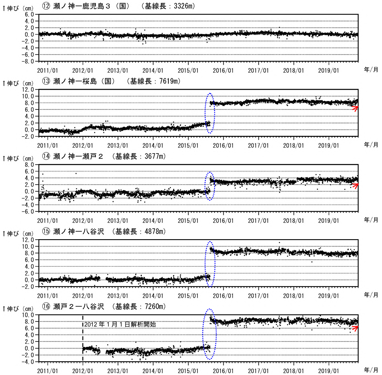
図 7-3 桜島 GNSS 連続観測による基線長変化（2010年11月～2019年10月）
