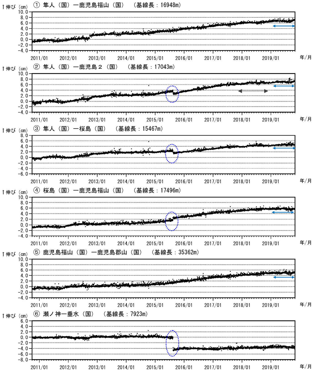
図 7-1 桜島 GNSS 連続観測による基線長変化（2010 年 11 月～2019 年 10 月）
