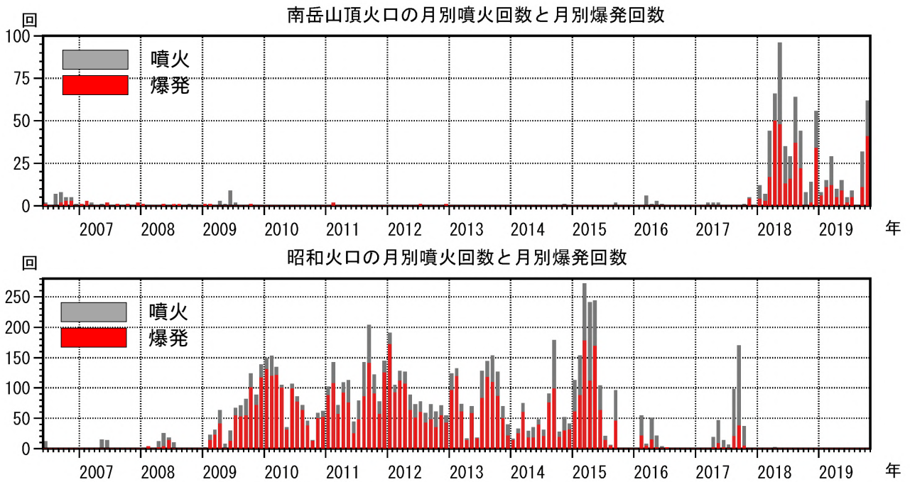
図 3-2 桜島 南岳山頂火口（上図）と昭和火口（下図）の月別噴火回数と月別爆発回数 （2006年6月～2019年10月）
