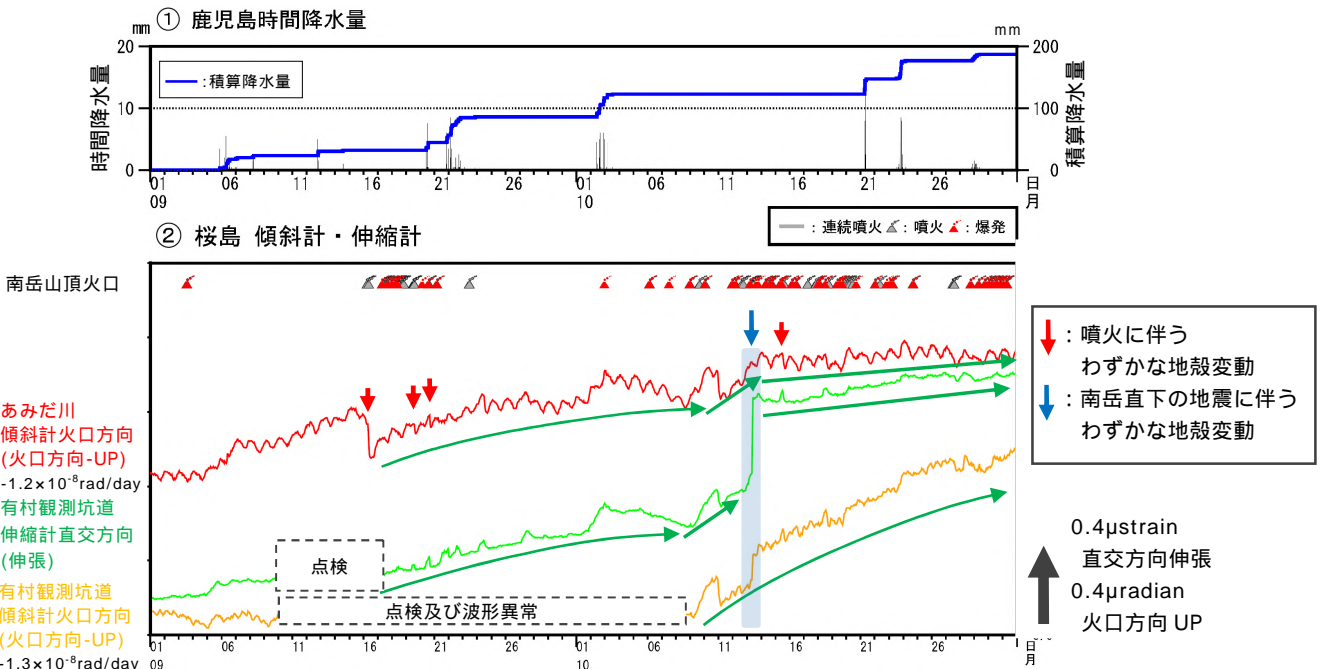
図 6-1 桜島 傾斜計及び伸縮計による地殻変動の状況（2019 年 9 月 1 日～10 月 31 日）
