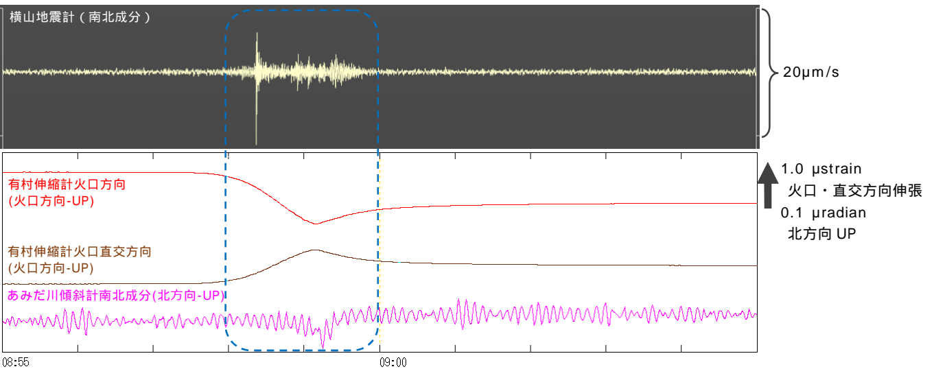
図 6-2 桜島 10 月 13 日 08 時 58 分～59 分頃の火山性地震の発生状況と地殻変動
